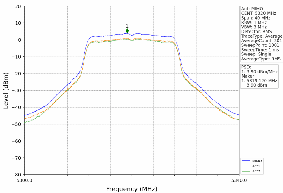
802.11a_HCH_5320MHz_MIMO_NTNV
