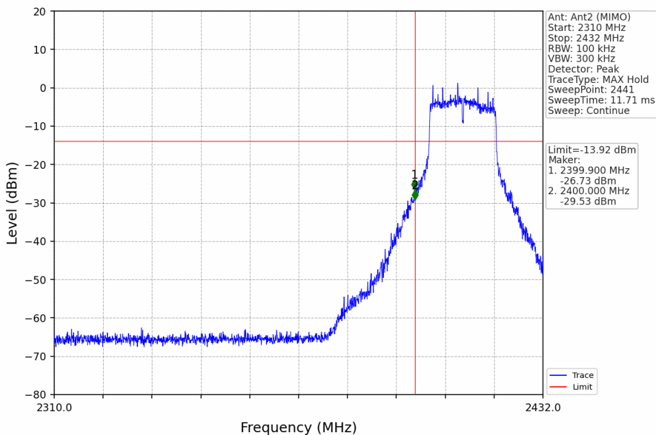
802.11g_LCH_2412MHz_Ant2 (MIMO)_NTNV
