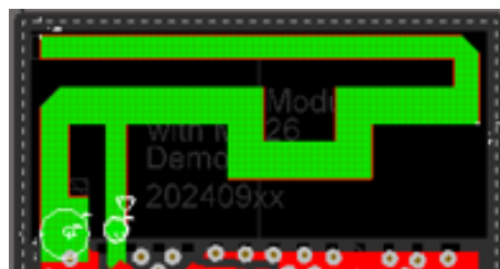
PIFA antenna
