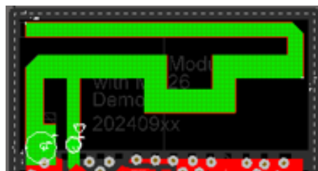
PIFA antenna
