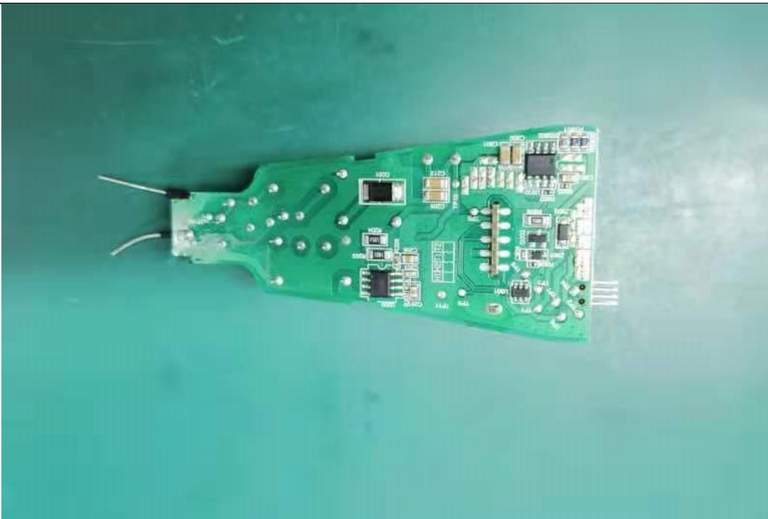
EUT Photo(2)
