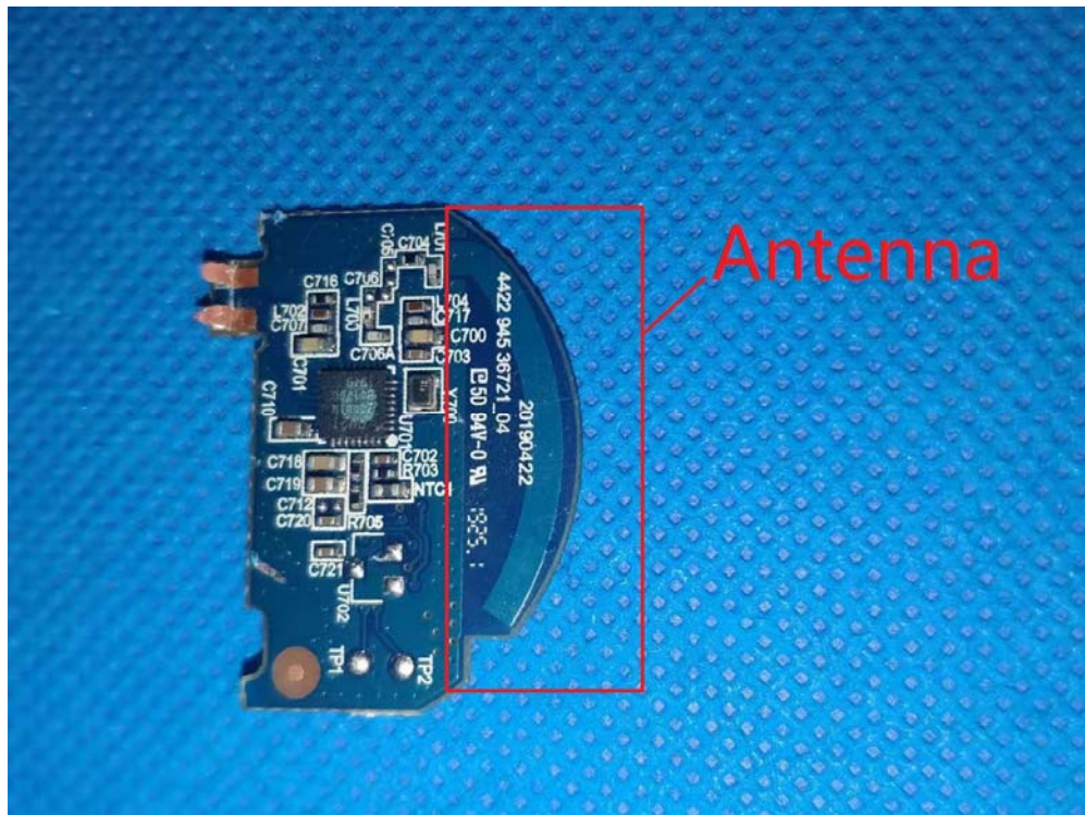
(7) EUT Photo (Zigbee)
