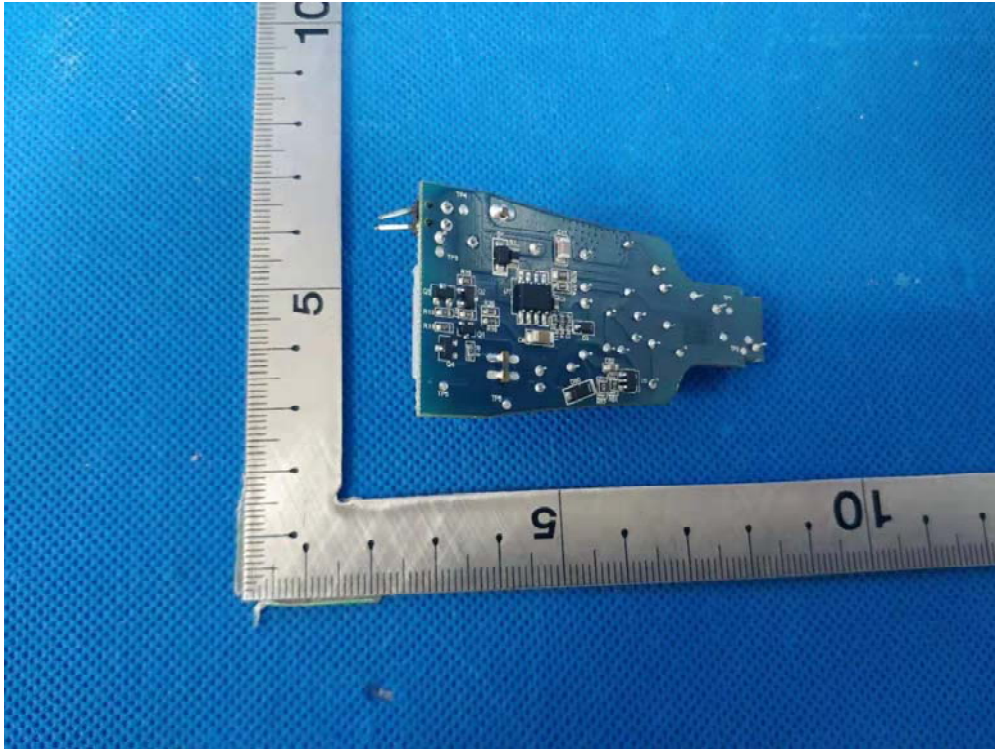
(9) EUT Photo (Zigbee)
