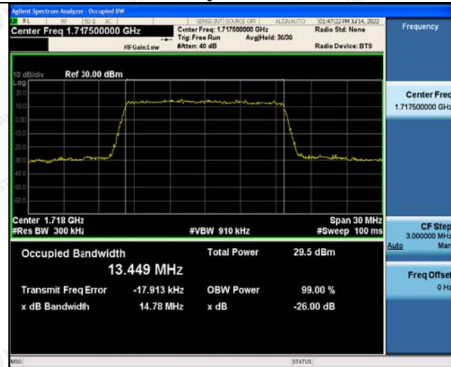
QPSK
