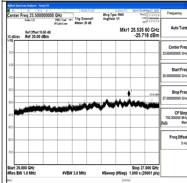
Band38_15MHz_QPSK_38000_1RB#0_20000~27000_2 0000~27000
