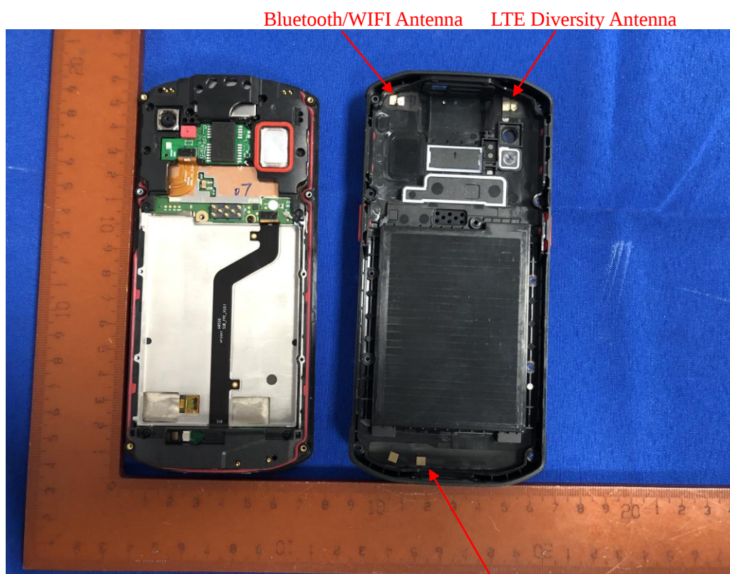
Fig. 5 GSM/WCDMA/LTE Main Antenna
