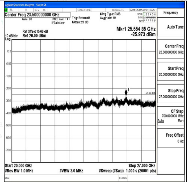
Band38_15MHz_16QAM_38175_1RB#0_20000~27000_0 20000~27000
