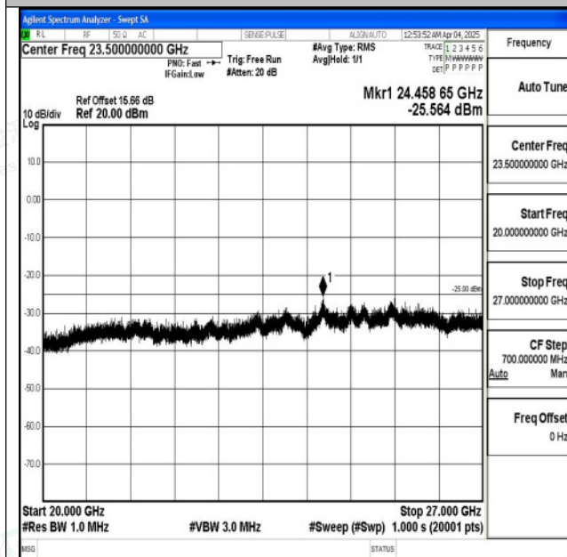
Band7_20MHz_QPSK_21350_1RB#0_20000~27000_20000~27000 000~27000
