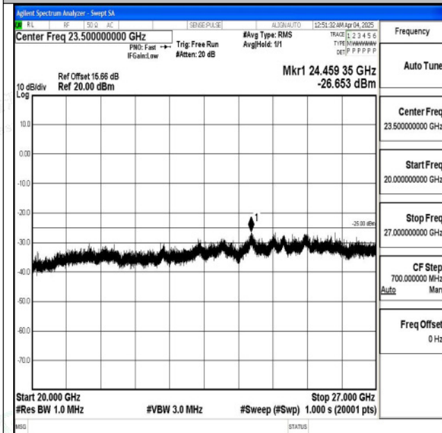
Band7_20MHz_QPSK_20850_1RB#0_20000~27000_20000~27000 000~27000
