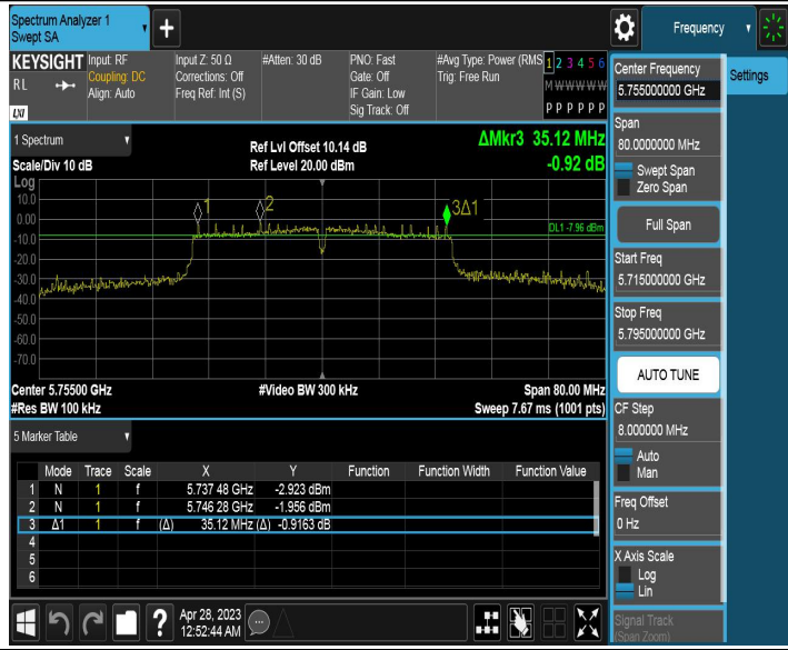
11AC40MIMO_Ant2_5755
