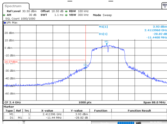
802.11n20_2412MHz_Chain 0
