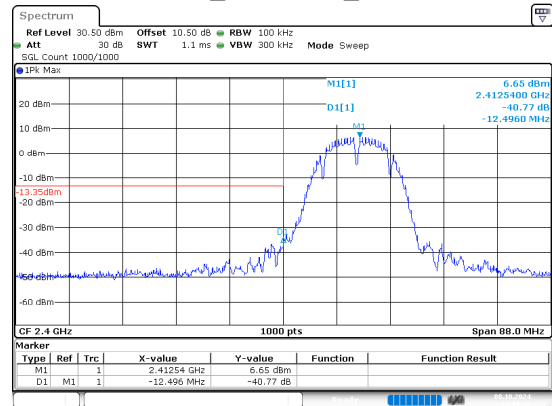
802.11b_2412MHz_Chain 1
