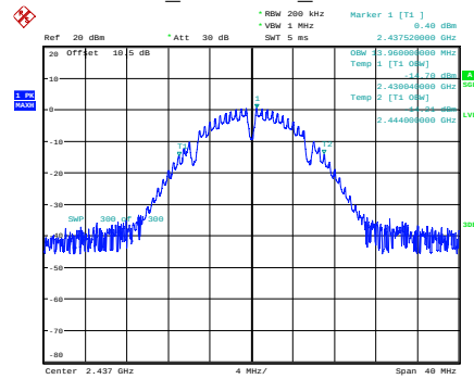
b_2437MHz_Chain 0
