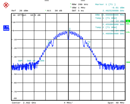
b_2462MHz_Chain 0
