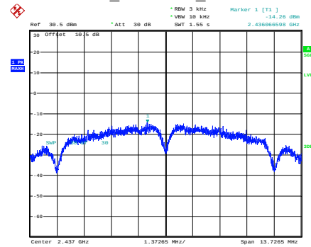
b_2437MHz_Chain 0
