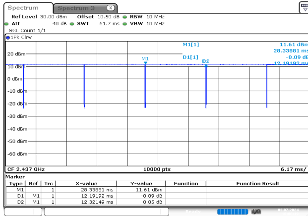
b_2437MHz_Chain 0
