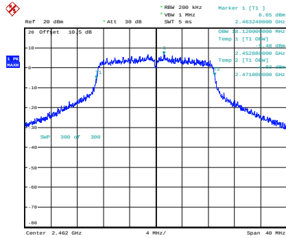
n20_2462MHz_Chain 0
