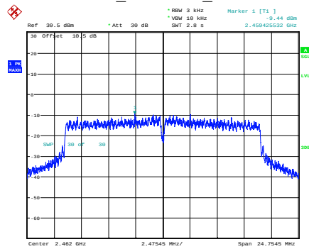
n20_2462MHz_Chain 0
