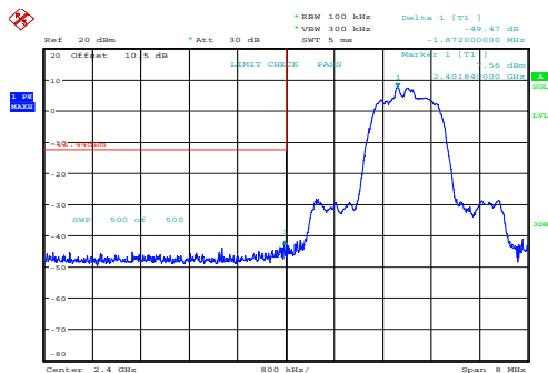
\pi/4 -DQPSK_Low
