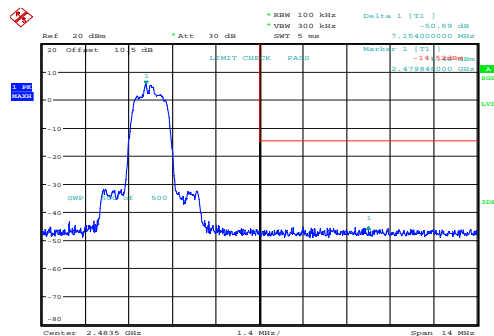
\pi/4 -DQPSK_High
