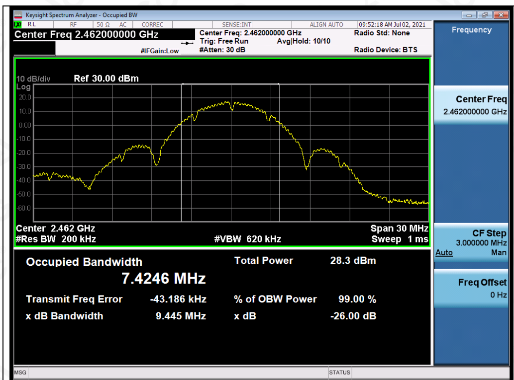
Test_Graph_CCK_ANT1_2462_1Mbps_OBW
