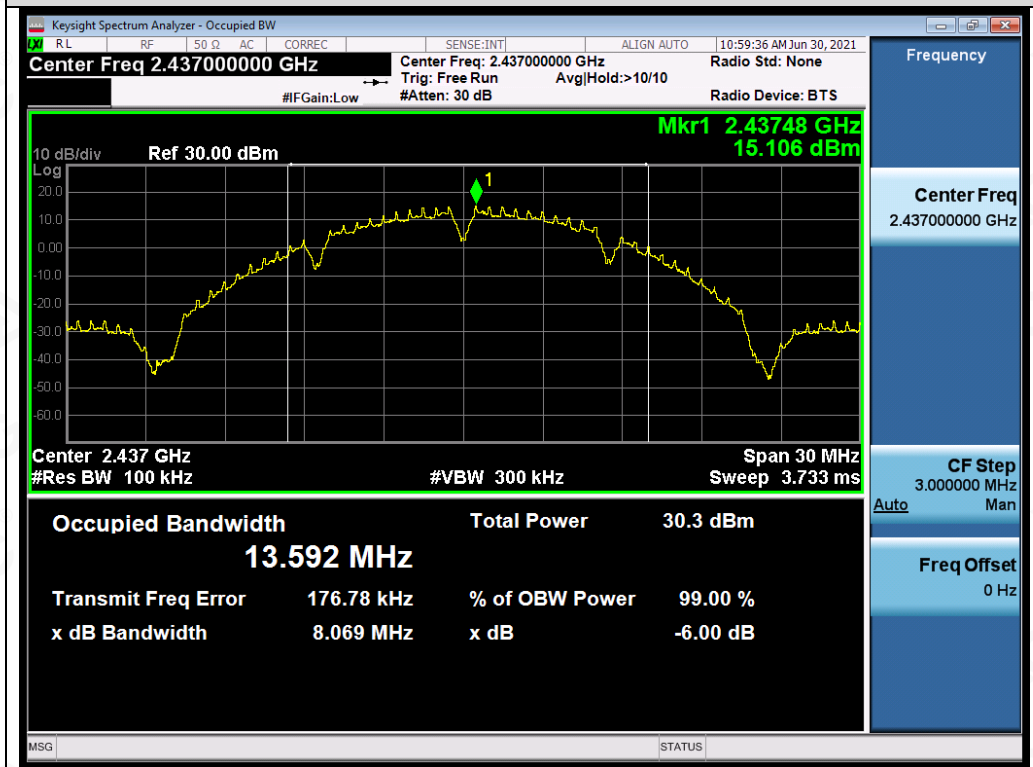
Test_Graph_802.11b_ANT1_2437_1Mbps_DTSSW
