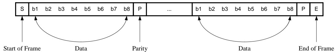
그림 2-4 Framing
