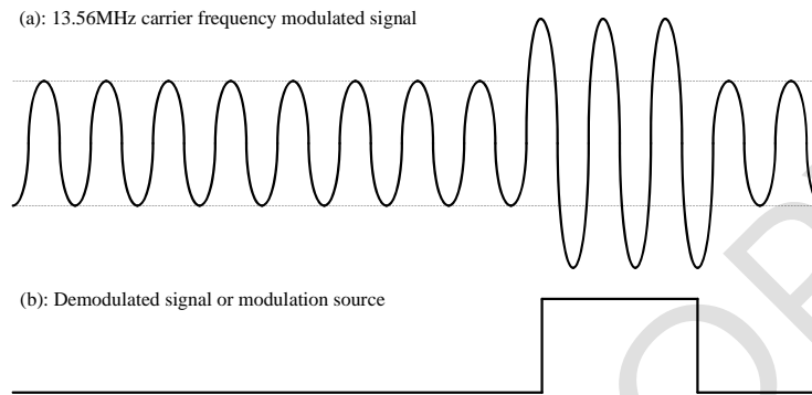
그림 2-2 Modulation / Demodulation
