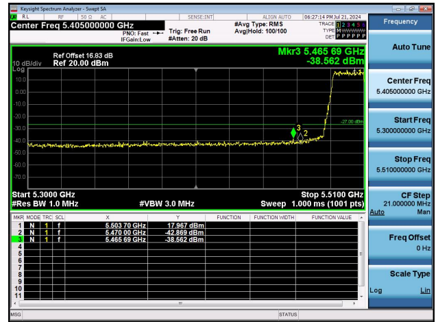
11AX20MIMO-Ant1-5500-PASS
