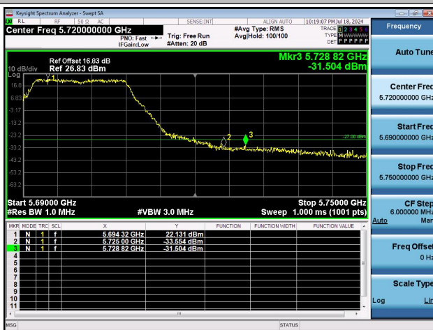
11A-Ant0-5700-PASS
