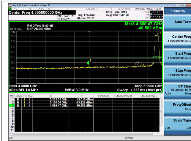
11AC20MIMO-Ant0-5320-PASS
