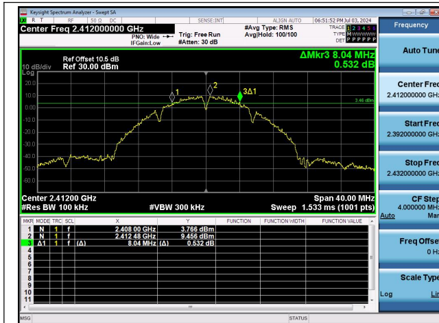
11B-Ant0-2412-PASS
