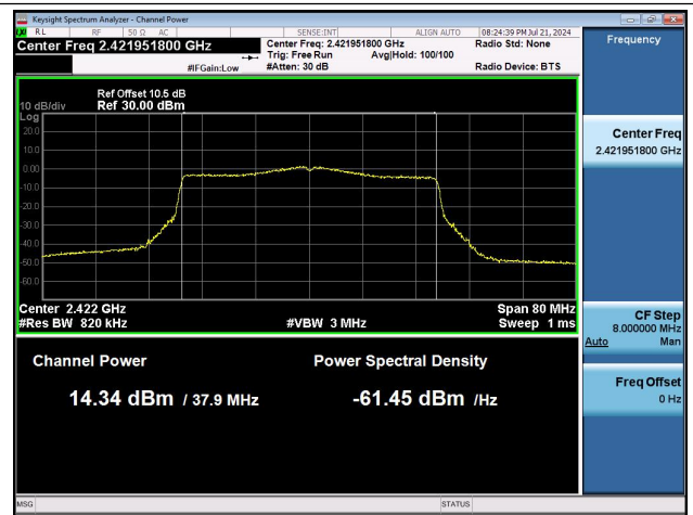
11AX40MIMO-Ant0-2422-PASS
