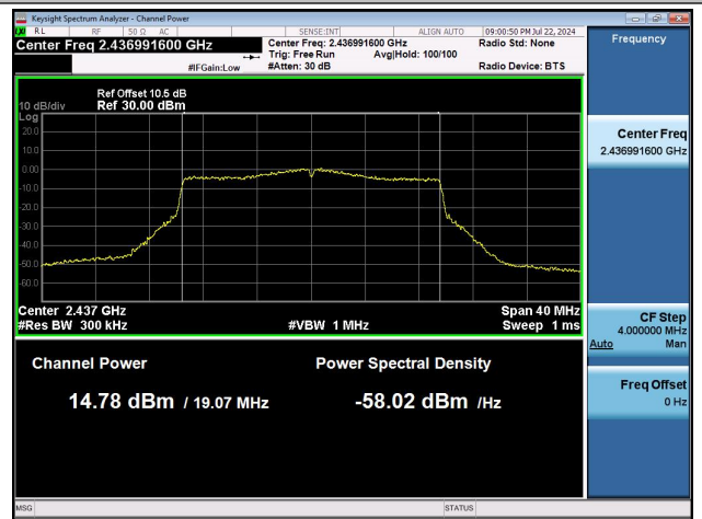
11AX20MIMO-Ant1-2437-PASS
