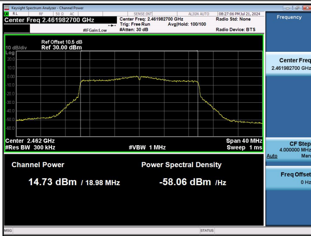
11AX20MIMO-Ant0-2462-PASS
