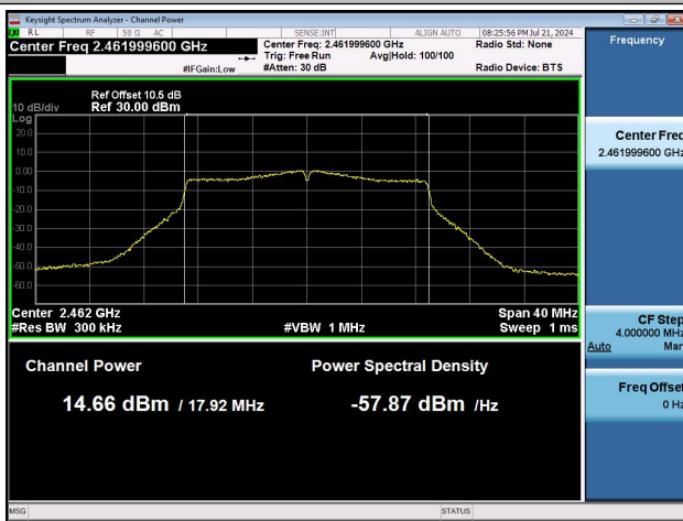
11N20MIMO-Ant0-2462-PASS
