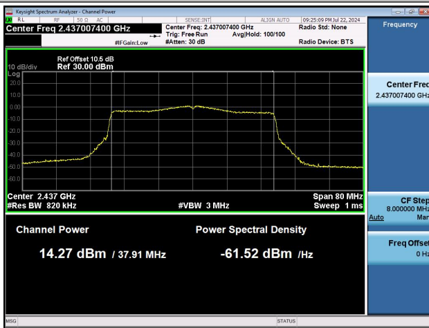
11AX40MIMO-Ant1-2437-PASS
