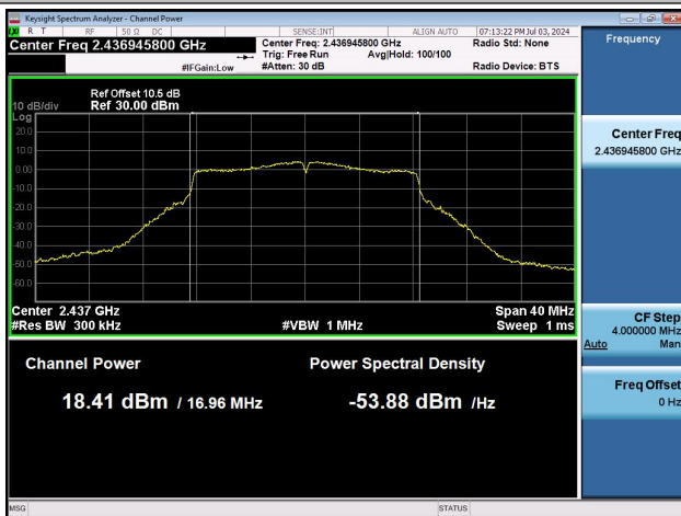
11G-Ant0-2437-PASS
