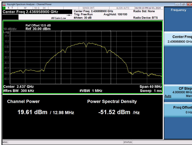
11B-Ant0-2437-PASS
