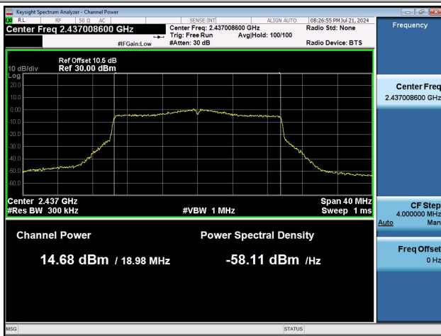
11AX20MIMO-Ant0-2437-PASS
