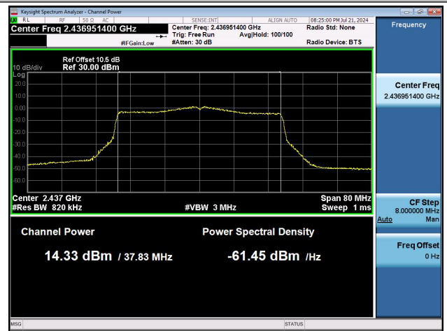
11AX40MIMO-Ant0-2437-PASS
