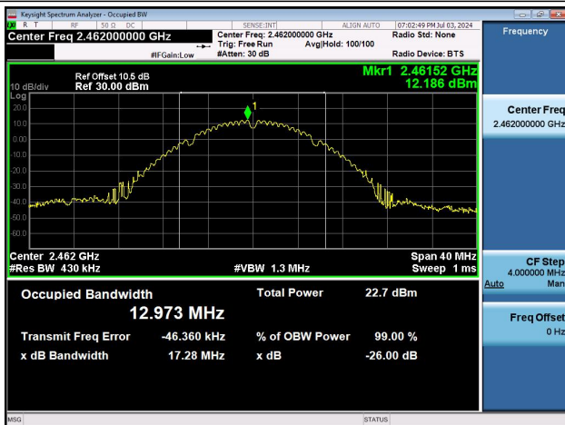
11B-Ant0-2462
