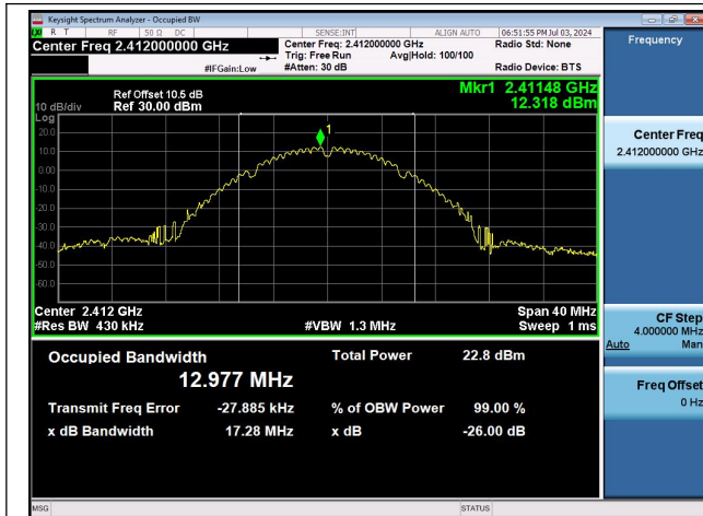
11B-Ant0-2412
