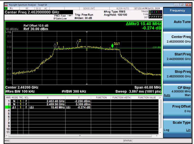
11N20MIMO-Ant0-2462-PASS
