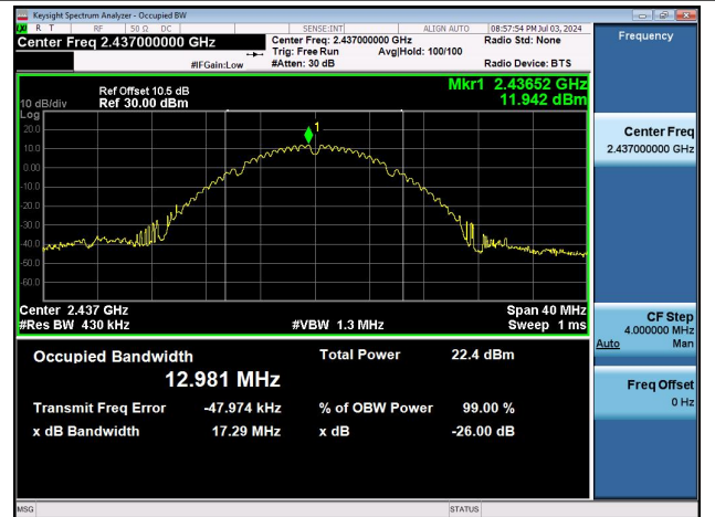
11B-Ant1-2437
