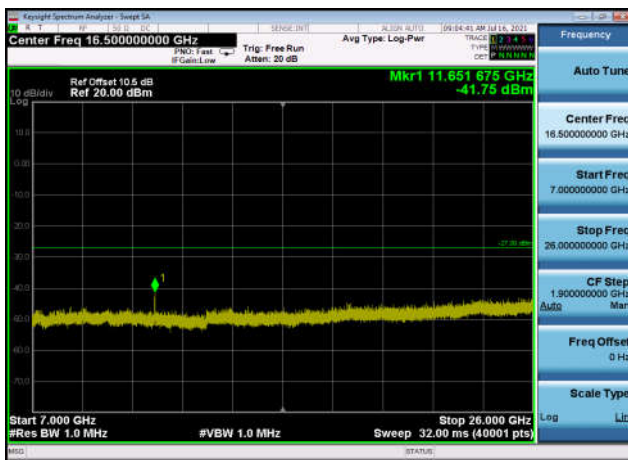
U-NII-3 ,Plot 4,7000MHz~26000MHz-802. 11ac(20MHz),5825MHz,Ant0
