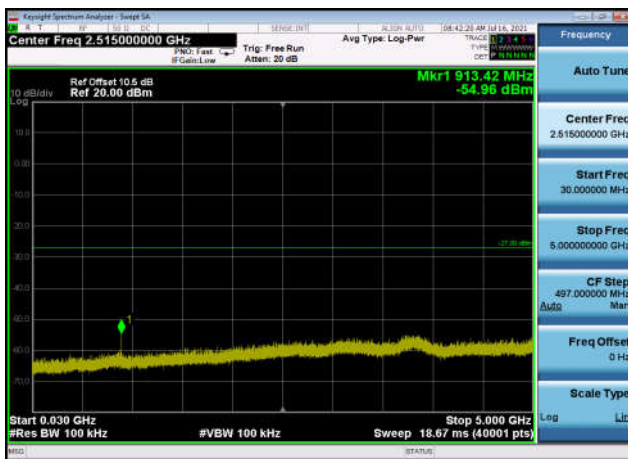
U-NII-3 ,Plot 2,30MHz~5000MHz-802.11a c(20MHz),5825MHz,Ant0
