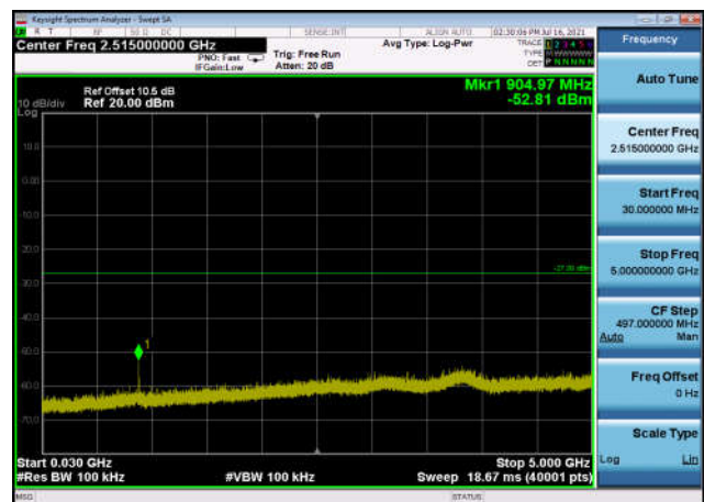
U-NII-3 ,Plot 2,30MHz~5000MHz-802.11a x(40MHz),5755MHz,Ant0
