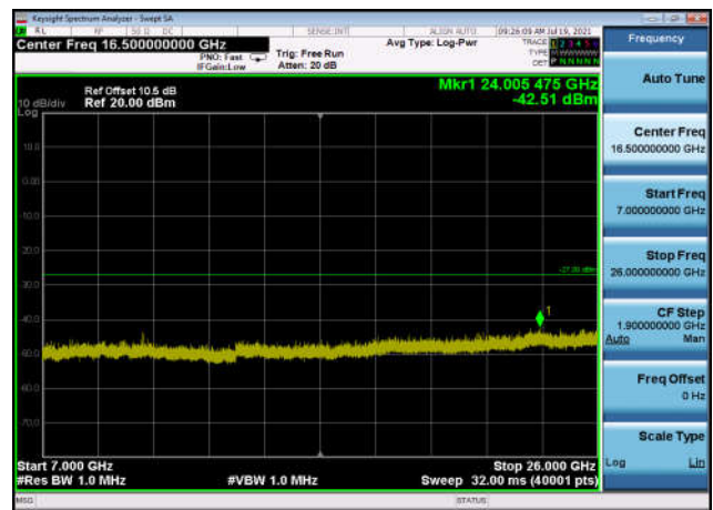
U-NII-1 ,Plot 4,7000MHz~26000MHz-802. 11ax(20MHz),5220MHz,Ant1
