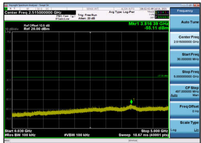
U-NII-3 ,Plot 2,30MHz~5000MHz-802.11n (20MHz),5825MHz,Ant0
