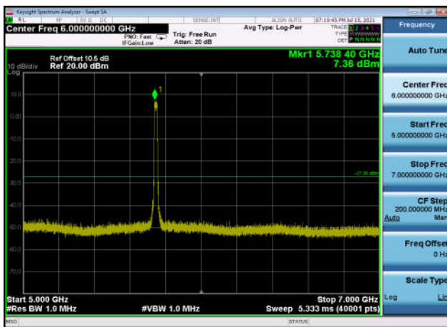
U-NII-3 ,Plot 3,5000MHz~7000MHz-802.1 1a(20MHz),5825MHz,Ant0
