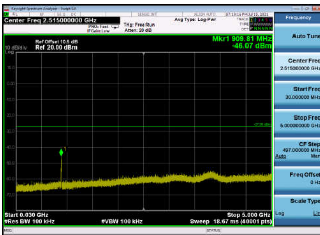
U-NII-3 ,Plot 2,30MHz~5000MHz-802.11a (20MHz),5745MHz,Ant0
