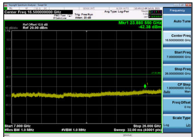
U-NII-1 ,Plot 4,7000MHz~26000MHz-802. 11ax(80MHz),5210MHz,Ant1
