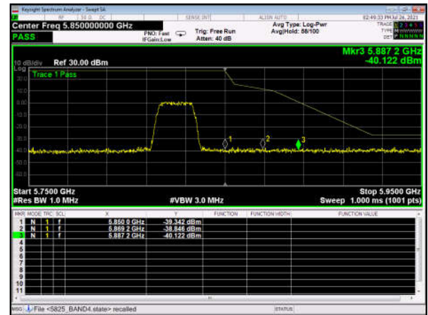
U-NII-3 ,Plot 1,Band Edge-802.11ac(20 MHz),5825MHz,Ant0
