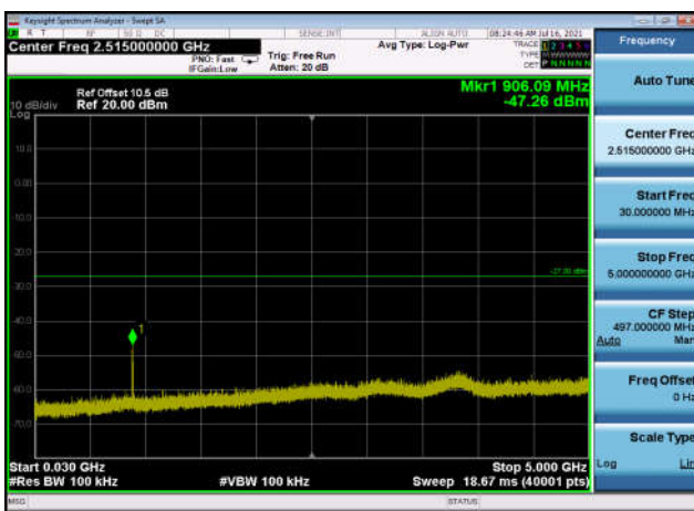
U-NII-3 ,Plot 2,30MHz~5000MHz-802.11n (20MHz),5785MHz,Ant0
