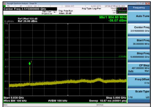
U-NII-3 ,Plot 2,30MHz~5000MHz-802.11a c(20MHz),5785MHz,Ant0
