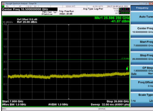
U-NII-1 ,Plot 4,7000MHz~26000MHz-802. 11ax(40MHz),5230MHz,Ant1
