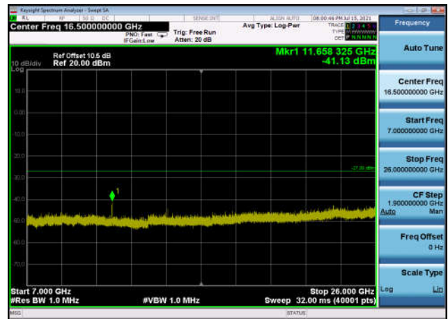
U-NII-3 ,Plot 4,7000MHz~26000MHz-802. 11ac(20MHz),5785MHz,Ant0
