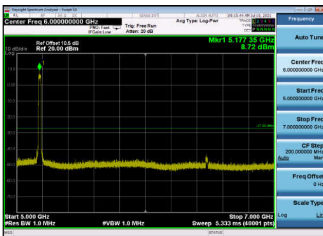
U-NII-1 ,Plot 3,5000MHz~7000MHz-802.1 1ax(20MHz),5180MHz,Ant1
