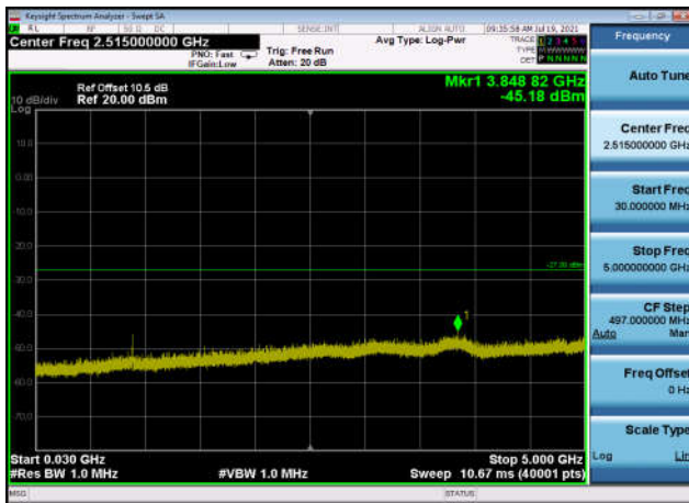
U-NII-1 ,Plot 2,30MHz~5000MHz-802.11a x(40MHz),5230MHz,Ant1
