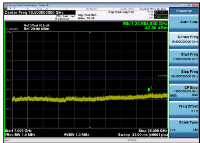
U-NII-3 ,Plot 4,7000MHz~26000MHz-802. 11ac(40MHz),5755MHz,Ant0
