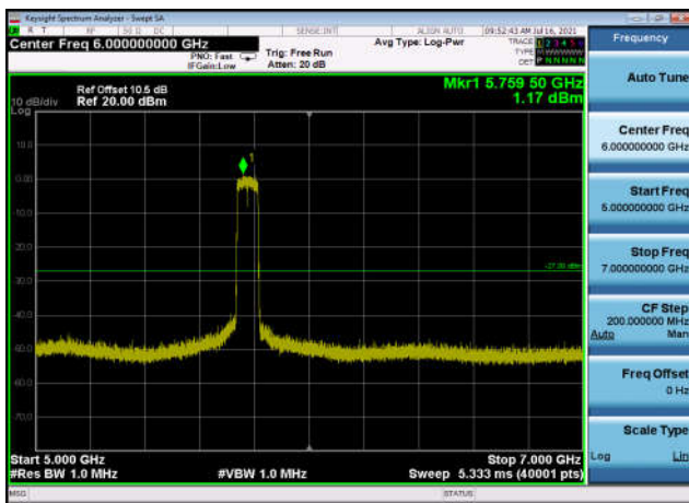
U-NII-3 ,Plot 3,5000MHz~7000MHz-802.1 1ac(80MHz),5775MHz,Ant0
