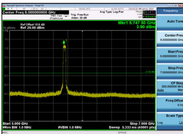
U-NII-3 ,Plot 3,5000MHz~7000MHz-802.1 1n(40MHz),5755MHz,Ant0
