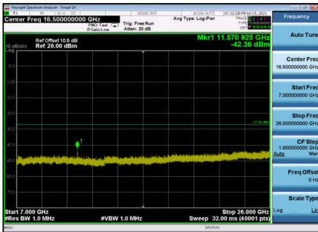
U-NII-3 ,Plot 4,7000MHz~26000MHz-802. 11ac(20MHz),5745MHz,Ant0
