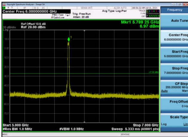
U-NII-3 ,Plot 3,5000MHz~7000MHz-802.1 1ac(40MHz),5755MHz,Ant0
