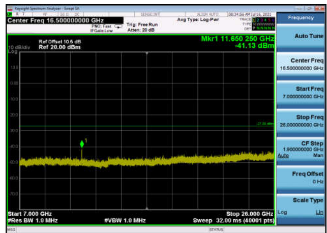
U-NII-3 ,Plot 4,7000MHz~26000MHz-802. 11n(20MHz),5825MHz,Ant0
