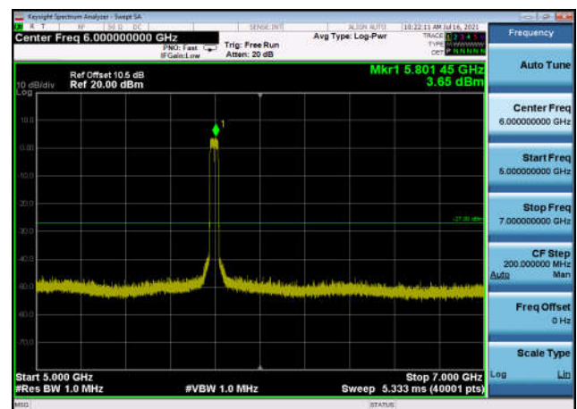
U-NII-3 ,Plot 3,5000MHz~7000MHz-802.1 1n(40MHz),5795MHz,Ant0
