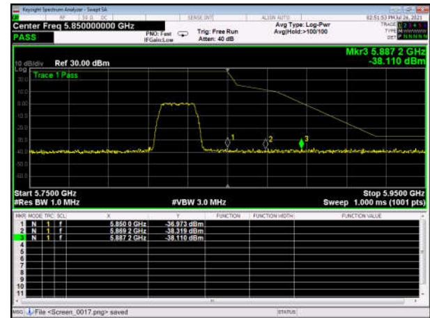
U-NII-3 ,Plot 1,Band Edge-802.11ax(40 MHz),5795MHz,Ant0
