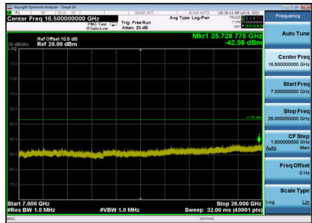
U-NII-1 ,Plot 4,7000MHz~26000MHz-802. 11ac(80MHz),5210MHz,Ant1
