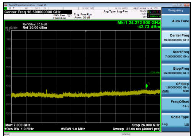
U-NII-3 ,Plot 4,7000MHz~26000MHz-802. 11n(20MHz),5825MHz,Ant0
