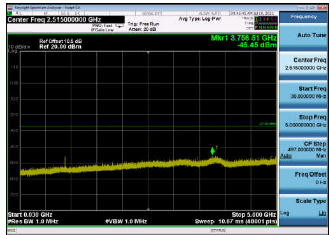
U-NII-1 ,Plot 2,30MHz~5000MHz-802.11a x(80MHz),5210MHz,Ant1
