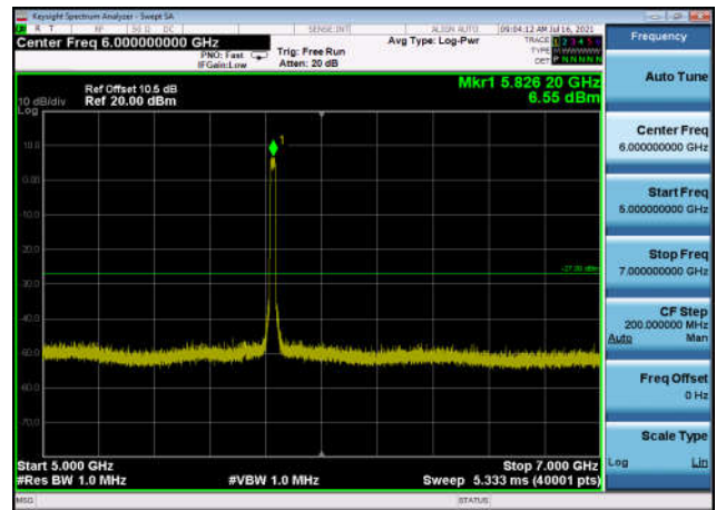
U-NII-3 ,Plot 3,5000MHz~7000MHz-802.1 1ac(40MHz),5795MHz,Ant0
