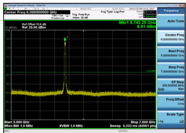
U-NII-3 ,Plot 3,5000MHz~7000MHz-802.1 1ac(20MHz),5745MHz,Ant0
