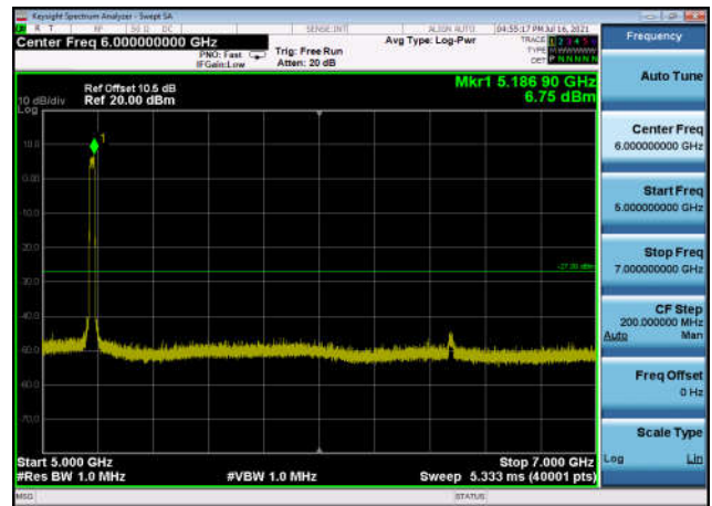
U-NII-1 ,Plot 3,5000MHz~7000MHz-802.1 1ac(20MHz),5240MHz,Ant1
