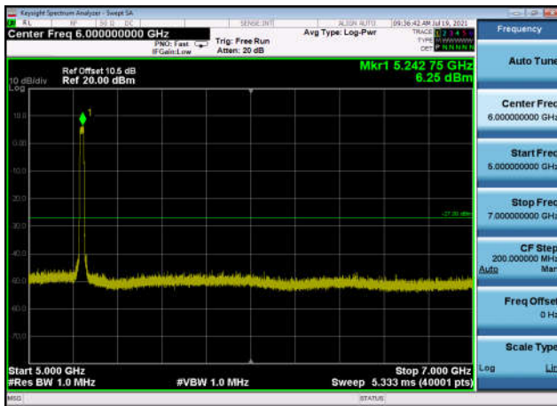
U-NII-1 ,Plot 3,5000MHz~7000MHz-802.1 1ax(40MHz),5230MHz,Ant1
