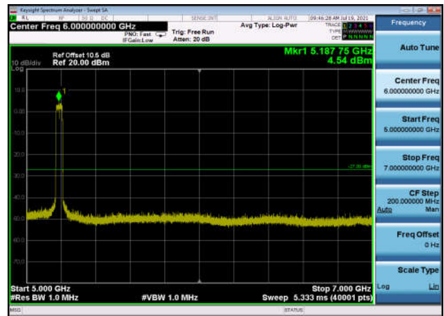
U-NII-1 ,Plot 3,5000MHz~7000MHz-802.1 1ax(80MHz),5210MHz,Ant1
