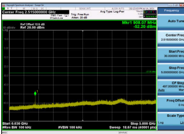
U-NII-3 ,Plot 2,30MHz~5000MHz-802.11a x(20MHz),5825MHz,Ant0
