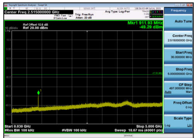
U-NII-3 ,Plot 2,30MHz~5000MHz-802.11a c(40MHz),5755MHz,Ant0
