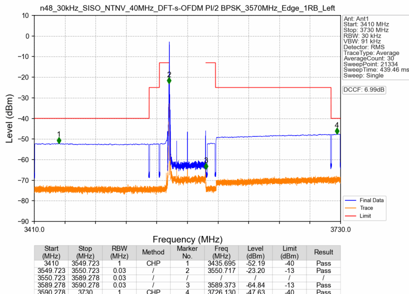
n48_30kHz_SISO_NTNV_40MHz_DFT-s-OFDM PI/2 BPSK_3570MHz_Edge_1RB_Left
