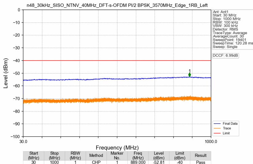
n48_30kHz_SISO_NTNV_40MHz_DFT-s-OFDM PI/2 BPSK_3570MHz_Edge_1RB_Left
