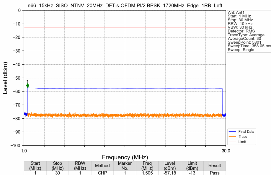
n66_15kHz_SISO_NTNV_20MHz_DFT-s-OFDM PI/2 BPSK_1720MHz_Edge_1RB_Left
