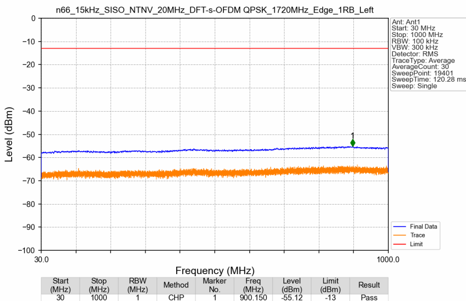
n66_15kHz_SISO_NTNV_20MHz_DFT-s-OFDM QPSK_1720MHz_Edge_1RB_Left
