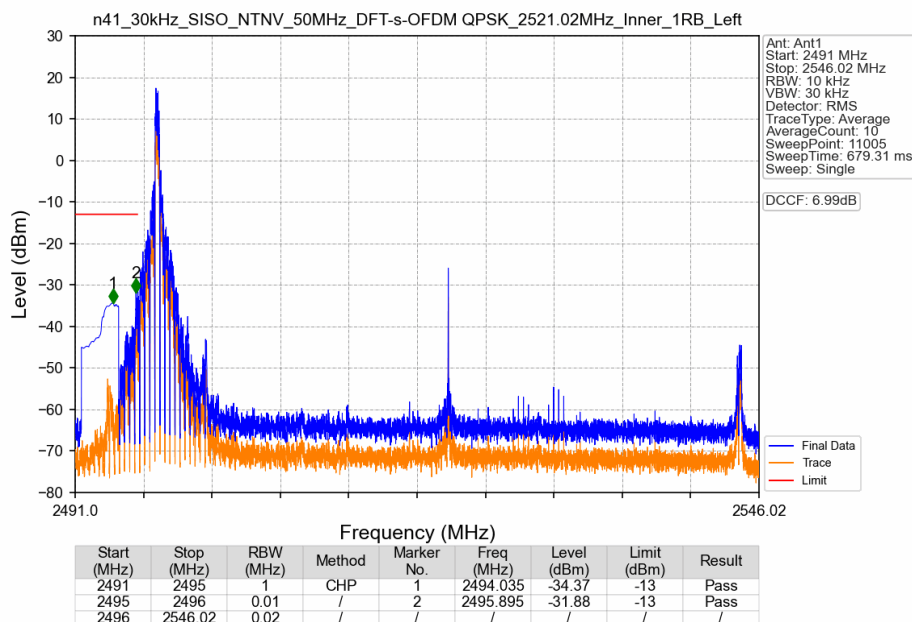
n41_30kHz_SISO_NTNV_50MHz_DFT-s-OFDM QPSK_2521.02MHz_Inner_1RB_Left
