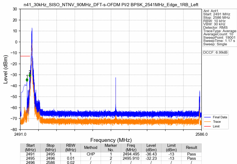
n41_30kHz_SISO_NTNV_90MHz_DFT-s-OFDM PI/2 BPSK_2541MHz_Edge_1RB_Left
