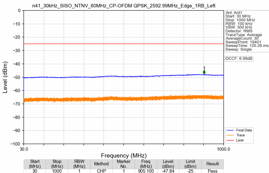
n41_30kHz_SISO_NTNV_60MHz_CP-OFDM QPSK_2592.99MHz_Edge_1RB_Left
