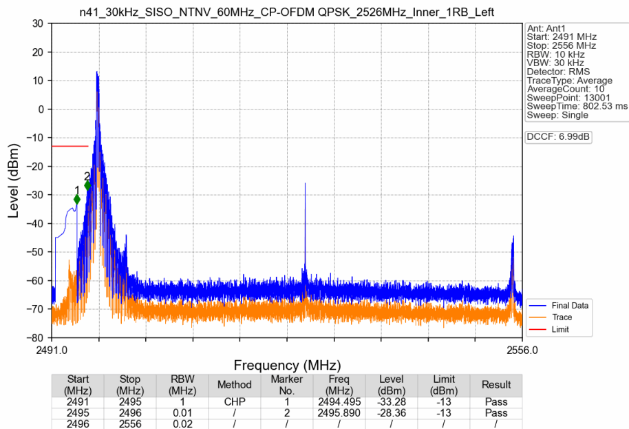
n41_30kHz_SISO_NTNV_60MHz_CP-OFDM QPSK_2526MHz_Inner_1RB_Left
