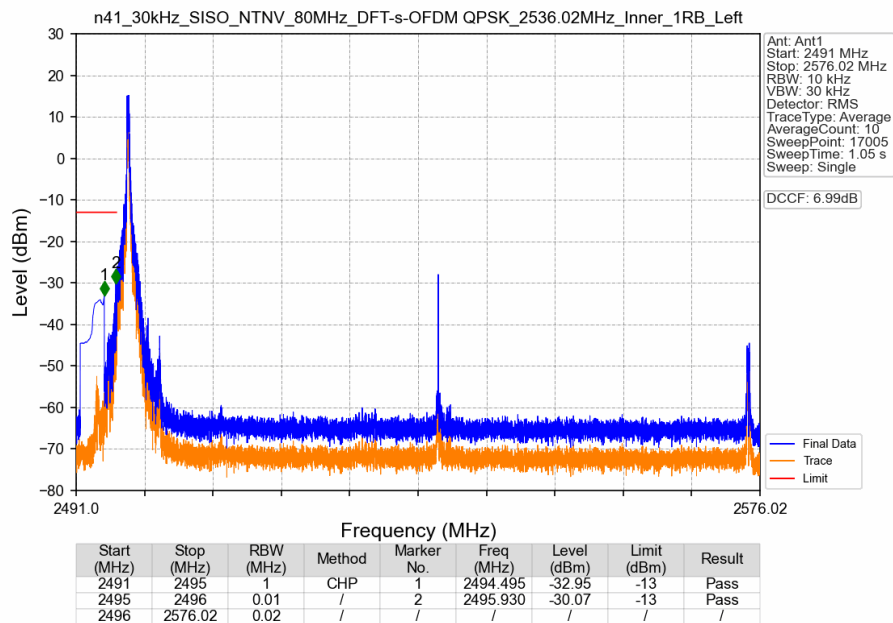
n41_30kHz_SISO_NTNV_80MHz_DFT-s-OFDM QPSK_2536.02MHz_Inner_1RB_Left
