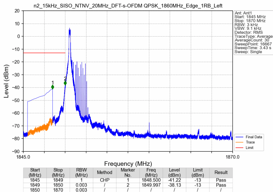
n2_15kHz_SISO_NTNV_20MHz_DFT-s-OFDM QPSK_1860MHz_Edge_1RB_Left
