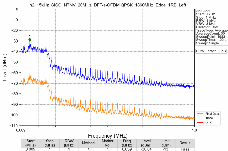
n2_15kHz_SISO_NTNV_20MHz_DFT-s-OFDM QPSK_1860MHz_Edge_1RB_Left
