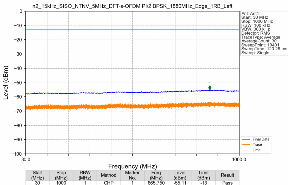
n2_15kHz_SISO_NTNV_5MHz_DFT-s-OFDM PI/2 BPSK_1880MHz_Edge_1RB_Left
