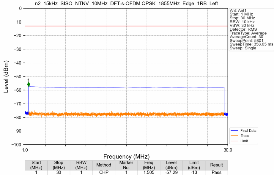
n2_15kHz_SISO_NTNV_10MHz_DFT-s-OFDM QPSK_1855MHz_Edge_1RB_Left
