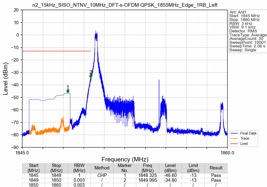
n2_15kHz_SISO_NTNV_10MHz_DFT-s-OFDM QPSK_1855MHz_Edge_1RB_Left
