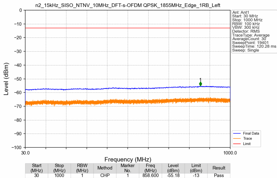
n2_15kHz_SISO_NTNV_10MHz_DFT-s-OFDM QPSK_1855MHz_Edge_1RB_Left
