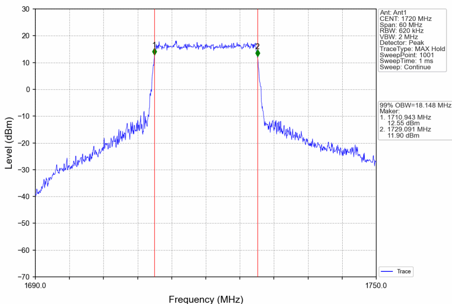
Band66_20MHz_16QAM_LCH_1720MHz_RB_100_0_NTNV
