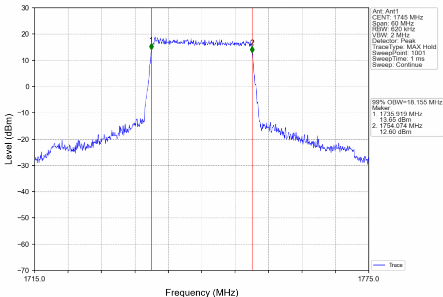
Band66_20MHz_QPSK_MCH_1745MHz_RB_100_0_NTNV
