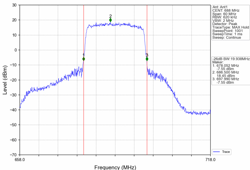
Band71_20MHz_16QAM_HCH_688MHz_RB_100_0_NTNV
