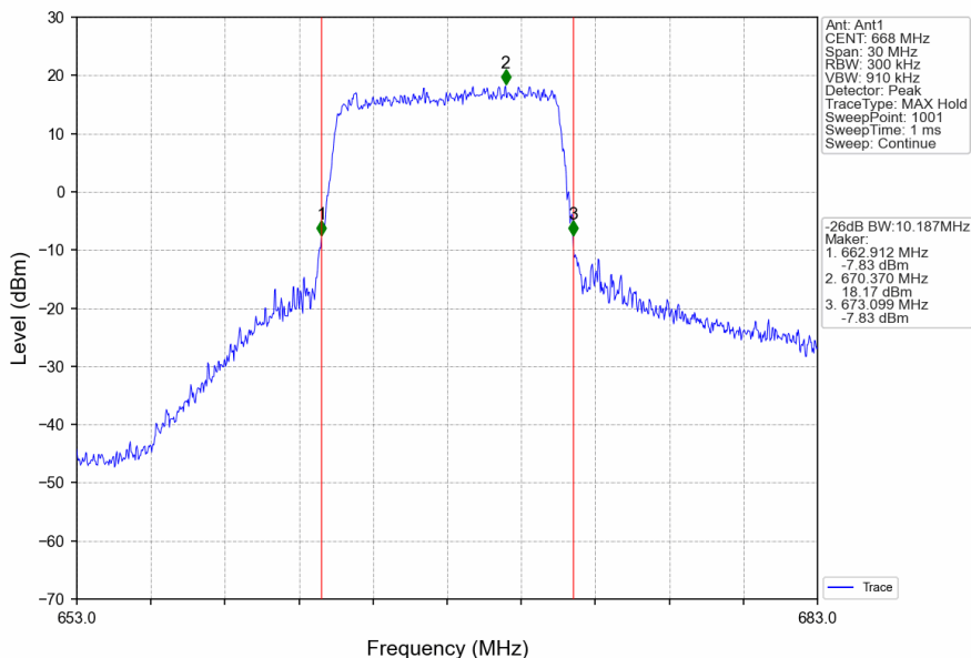
Band71_10MHz_16QAM_LCH_668MHz_RB_50_0_NTNV
