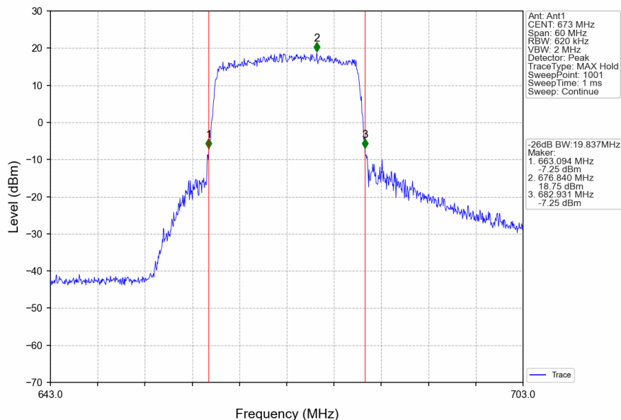
Band71_20MHz_16QAM_LCH_673MHz_RB_100_0_NTNV
