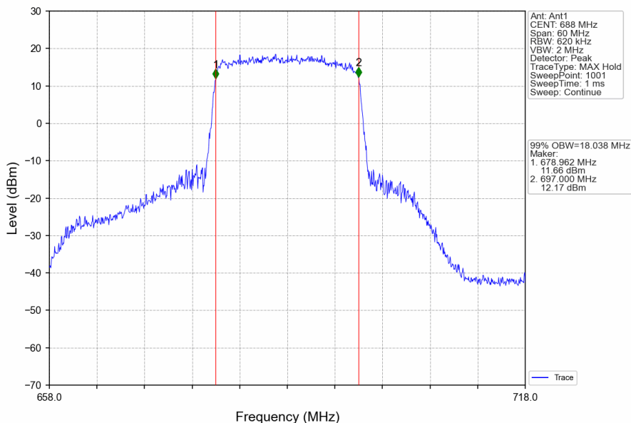
Band71_20MHz_16QAM_HCH_688MHz_RB_100_0_NTNV
