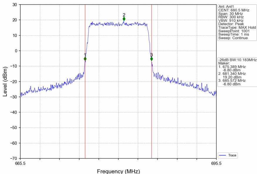
Band71_10MHz_QPSK_MCH_680.5MHz_RB_50_0_NTNV
