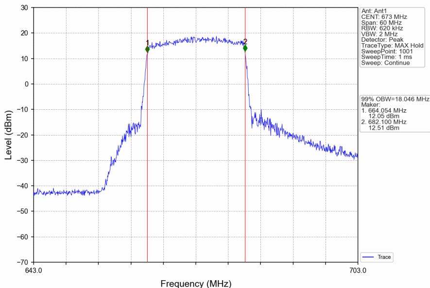
Band71_20MHz_16QAM_LCH_673MHz_RB_100_0_NTNV
