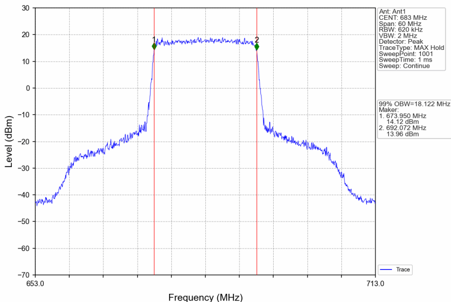
Band71_20MHz_QPSK_MCH_683MHz_RB_100_0_NTNV
