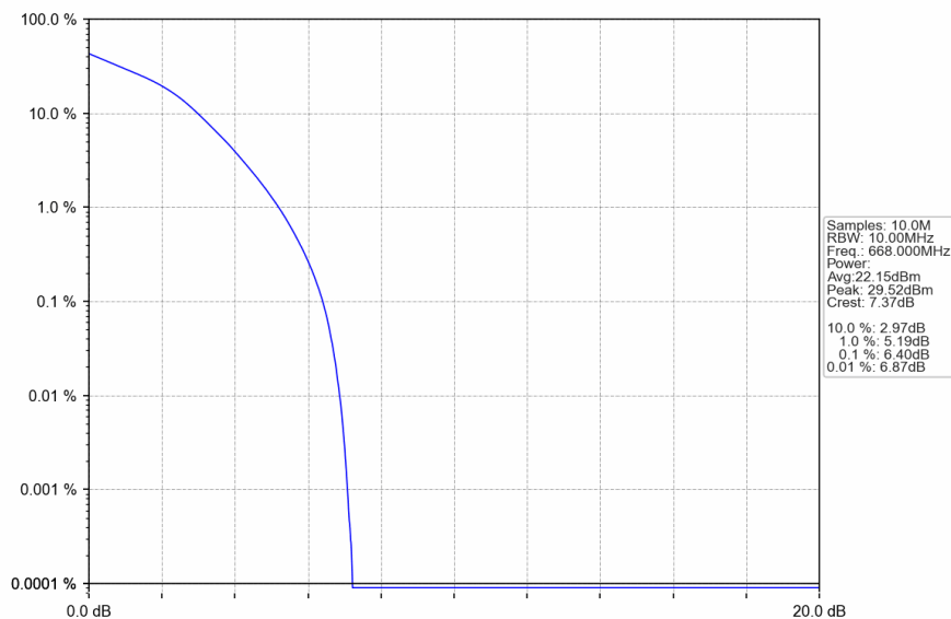
Band71_10MHz_16QAM_LCH_668MHz_RB_50_0_NTNV
