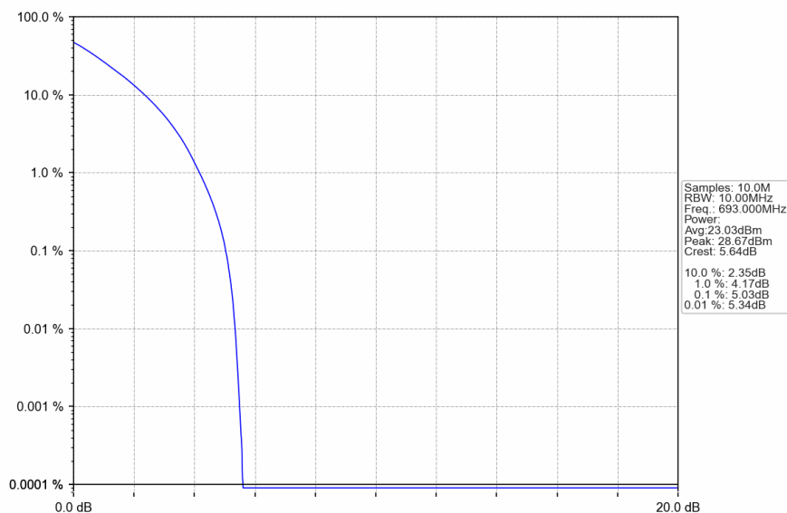
Band71_10MHz_QPSK_HCH_693MHz_RB_50_0_NTNV
