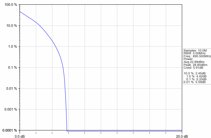
Band71_5MHz_QPSK_HCH_695.5MHz_RB_25_0_NTNV
