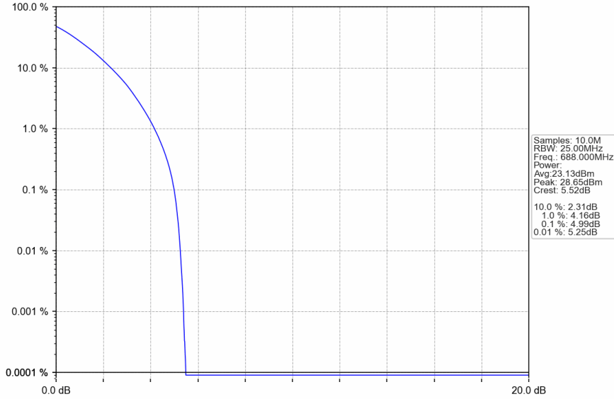
Band71_20MHz_QPSK_HCH_688MHz_RB_100_0_NTNV
