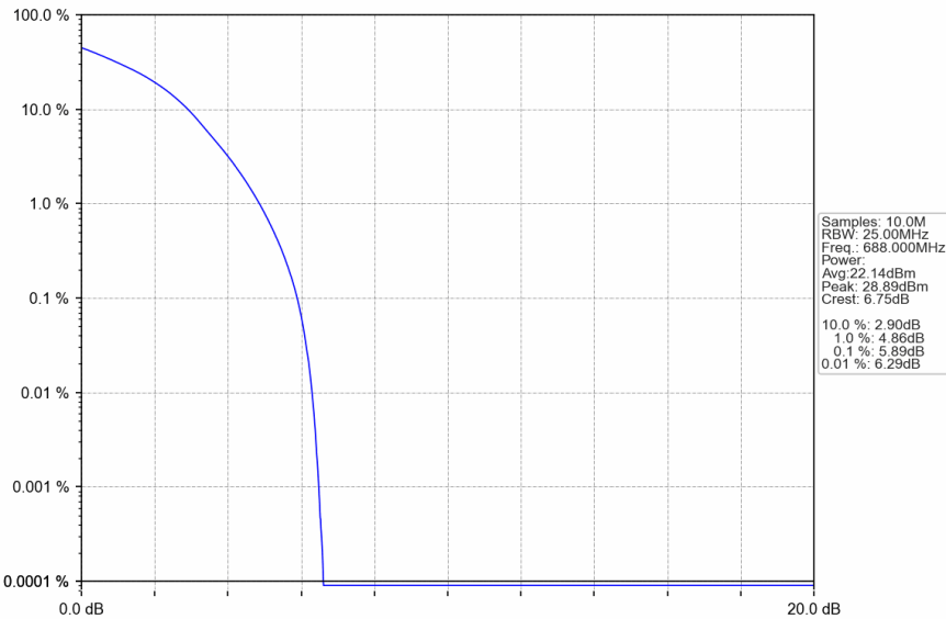
Band71_20MHz_16QAM_HCH_688MHz_RB_100_0_NTNV
