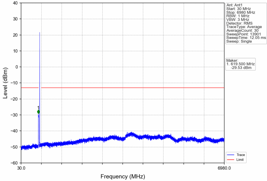
Band71_20MHz_16QAM_LCH_673MHz_RB_100_0_NTNV
