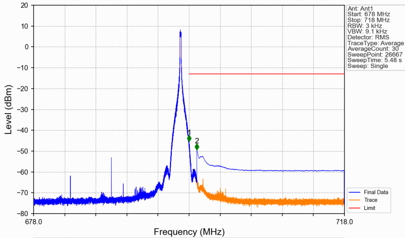
Band71_20MHz_QPSK_HCH_688MHz_RB_1_99_NTNV
