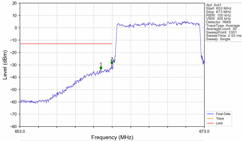
Band71_10MHz_16QAM_LCH_668MHz_RB_50_0_NTNV
