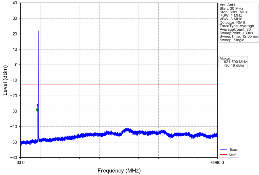
Band71_10MHz_16QAM_LCH_668MHz_RB_50_0_NTNV
