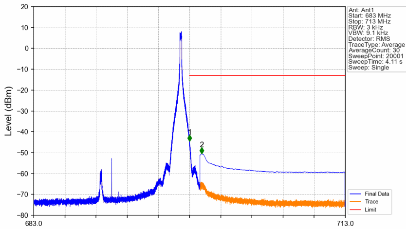
Band71_15MHz_QPSK_HCH_690.5MHz_RB_1_74_NTNV
