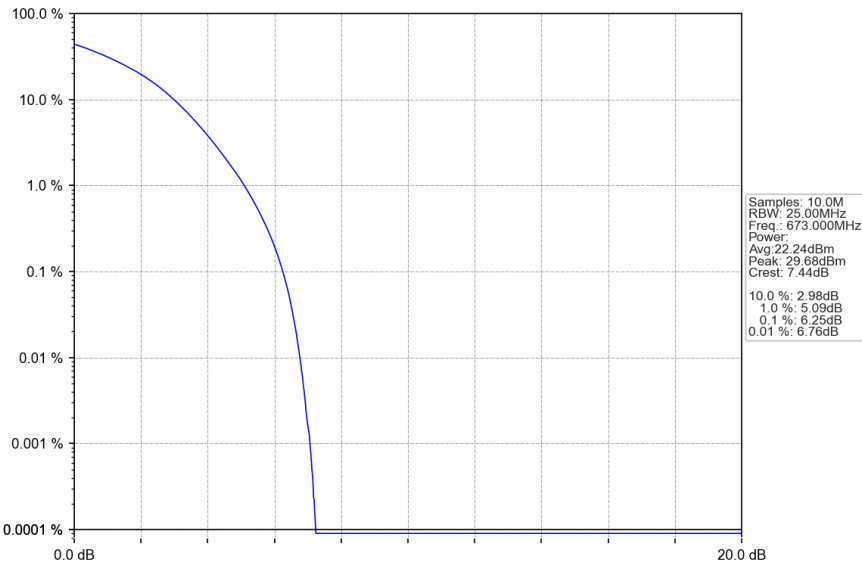
Band71_20MHz_16QAM_LCH_673MHz_RB_100_0_NTNV
