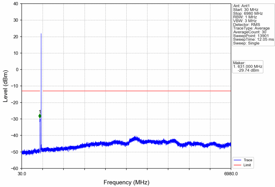
Band71_20MHz_16QAM_HCH_688MHz_RB_1_0_NTNV
