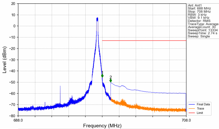
Band71_10MHz_QPSK_HCH_693MHz_RB_1_49_NTNV
