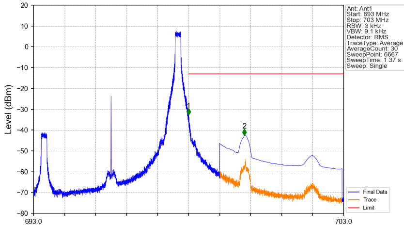
Band71_5MHz_QPSK_HCH_695.5MHz_RB_1_24_NTNV
