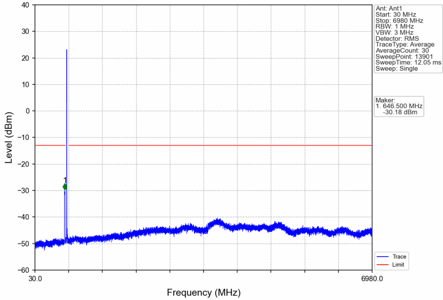
Band71_15MHz_QPSK_HCH_690.5MHz_RB_1_74_NTNV
