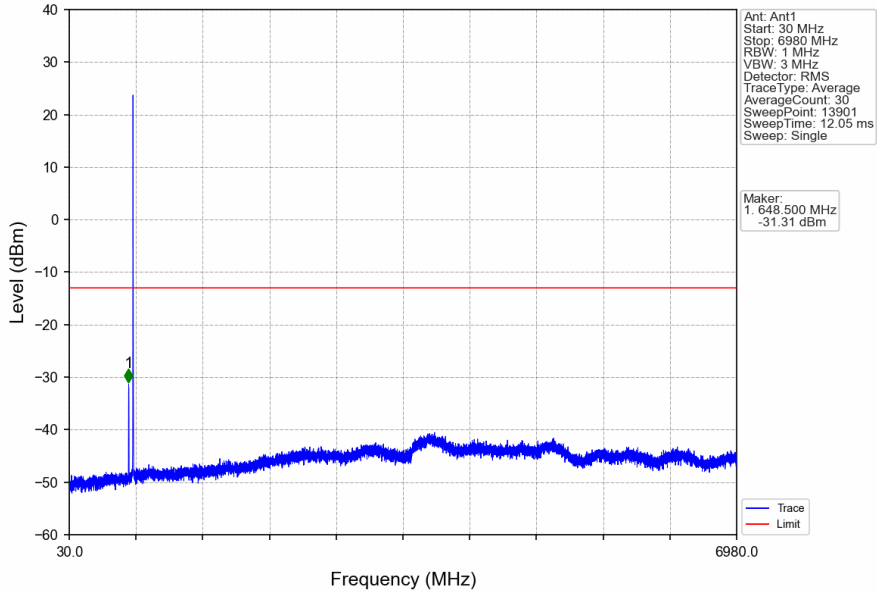
Band71_5MHz_QPSK_HCH_695.5MHz_RB_1_24_NTNV
