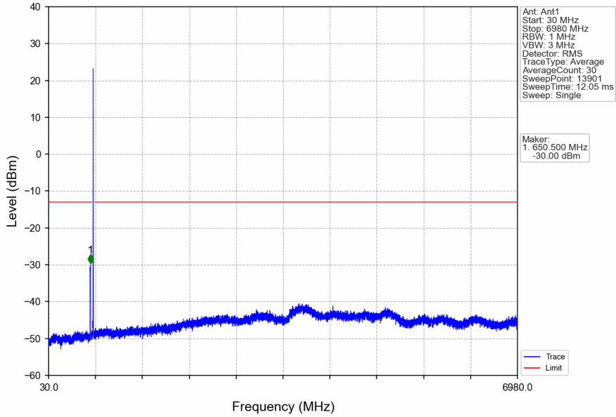
Band71_10MHz_QPSK_HCH_693MHz_RB_1_49_NTNV
