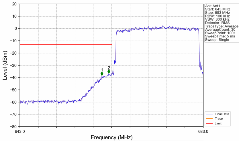
Band71_20MHz_16QAM_LCH_673MHz_RB_100_0_NTNV
