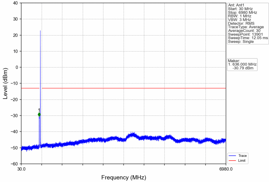
Band71_20MHz_QPSK_HCH_688MHz_RB_1_99_NTNV
