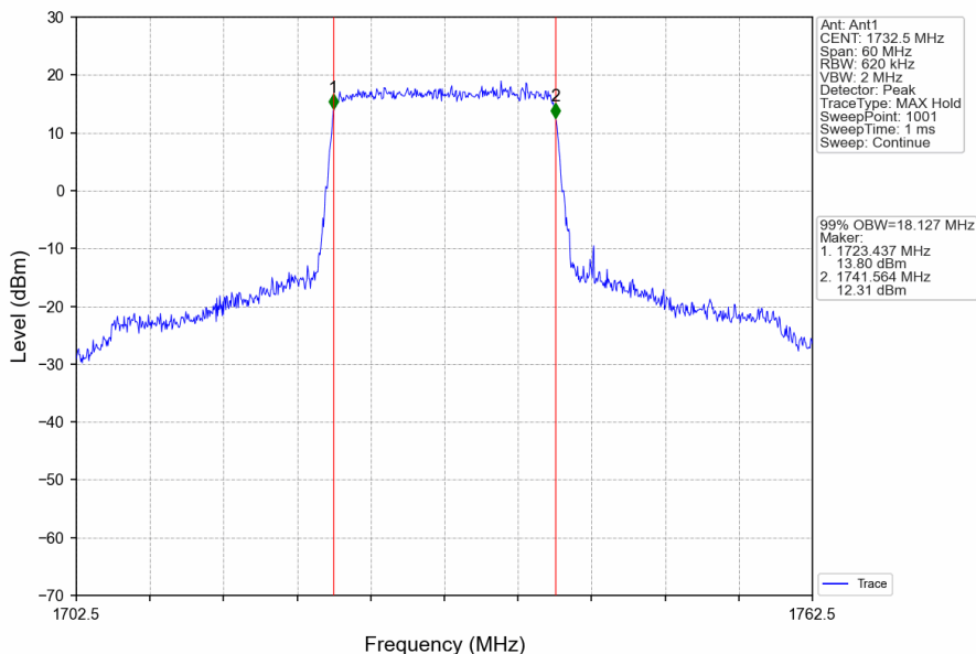
Band4_20MHz_QPSK_MCH_1732.5MHz_RB_100_0_NTNV
