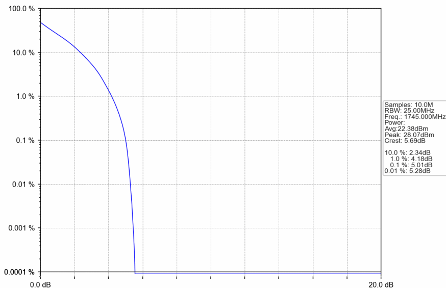
Band4_20MHz_QPSK_HCH_1745MHz_RB_100_0_NTNV
