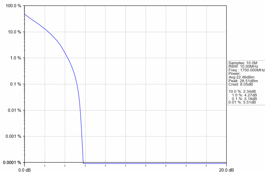
Band4_10MHz_QPSK_HCH_1750MHz_RB_50_0_NTNV
