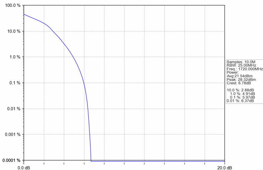
Band4_20MHz_16QAM_LCH_1720MHz_RB_100_0_NTNV
