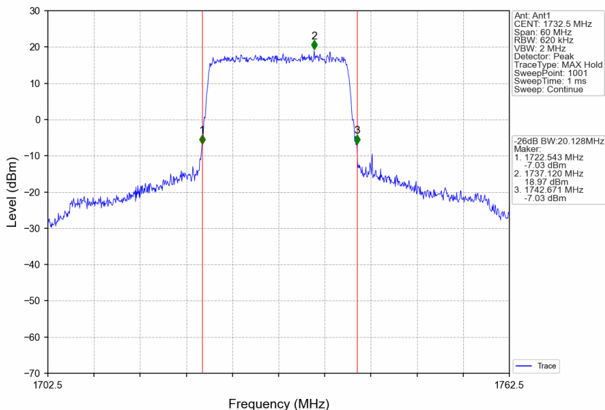
Band4_20MHz_QPSK_MCH_1732.5MHz_RB_100_0_NTNV
