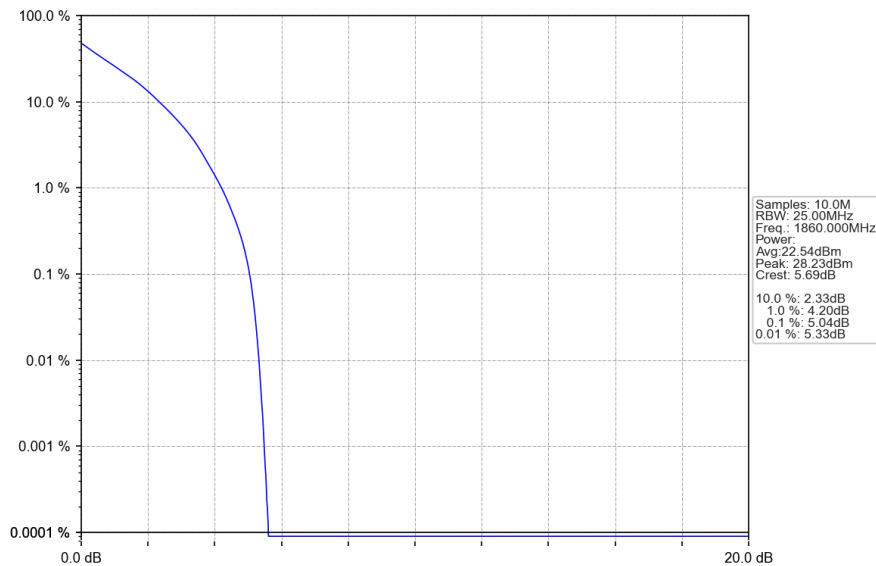
Band25_20MHz_QPSK_LCH_1860MHz_RB_100_0_NTNV
