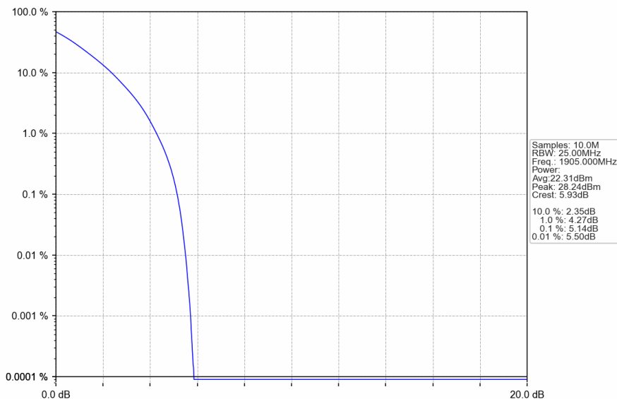
Band25_20MHz_QPSK_HCH_1905MHz_RB_100_0_NTNV
