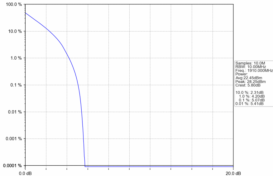
Band25_10MHz_QPSK_HCH_1910MHz_RB_50_0_NTNV
