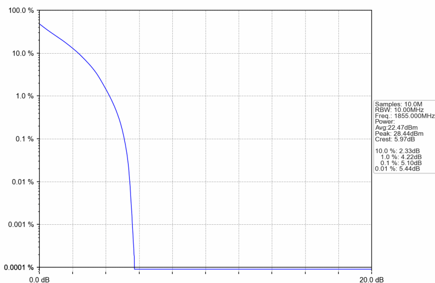
Band25_10MHz_QPSK_LCH_1855MHz_RB_50_0_NTNV
