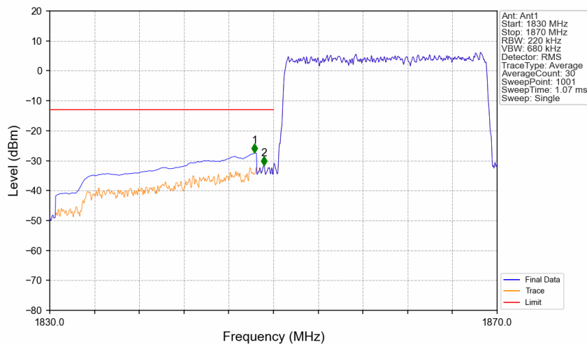
Band25_20MHz_QPSK_LCH_1860MHz_RB_100_0_NTNV
