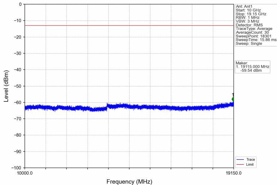
Band25_20MHz_QPSK_HCH_1905MHz_RB_1_0_NTNV
