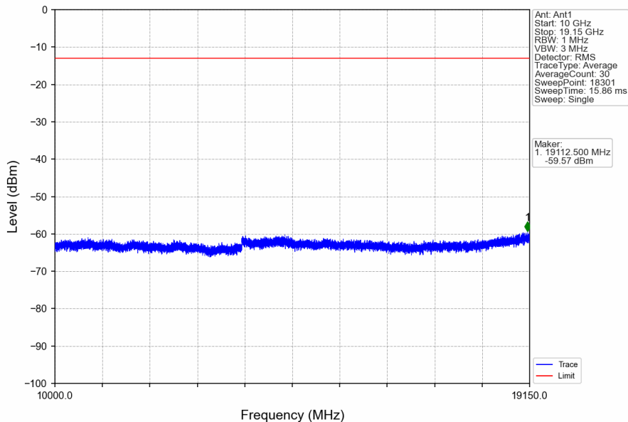
Band25_10MHz_QPSK_LCH_1855MHz_RB_50_0_NTNV
