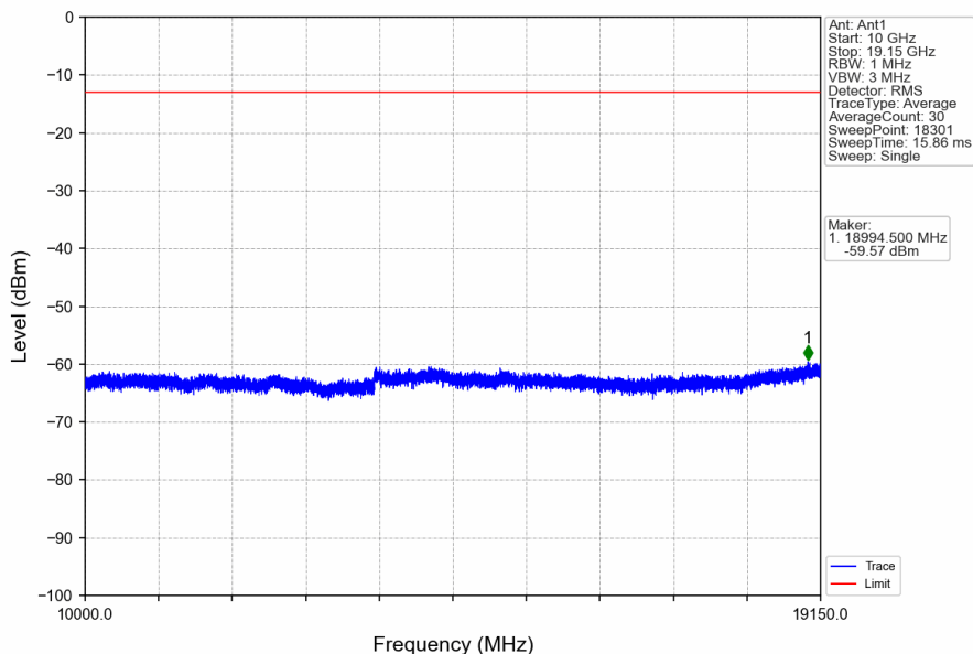
Band25_10MHz_QPSK_HCH_1910MHz_RB_1_0_NTNV
