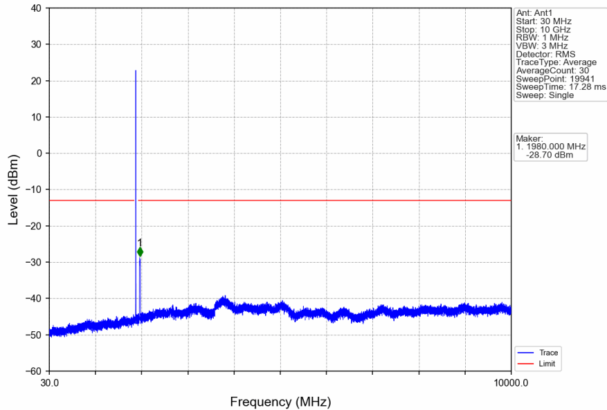
Band25_20MHz_QPSK_HCH_1905MHz_RB_1_0_NTNV
