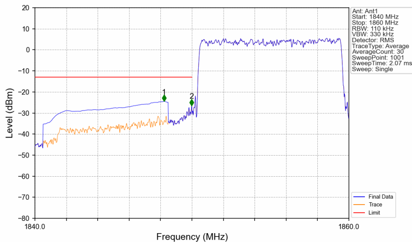
Band25_10MHz_QPSK_LCH_1855MHz_RB_50_0_NTNV
