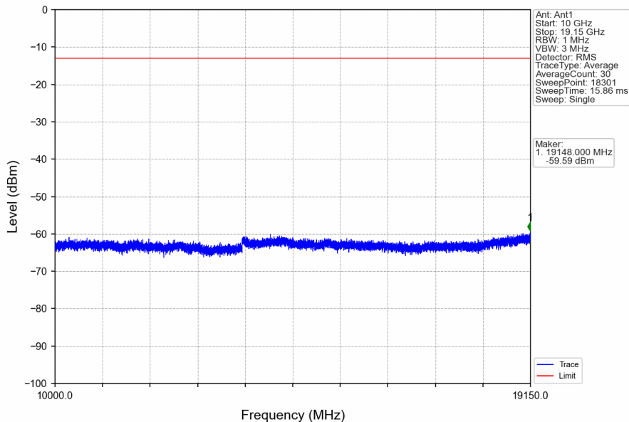
Band25_20MHz_QPSK_LCH_1860MHz_RB_100_0_NTNV
