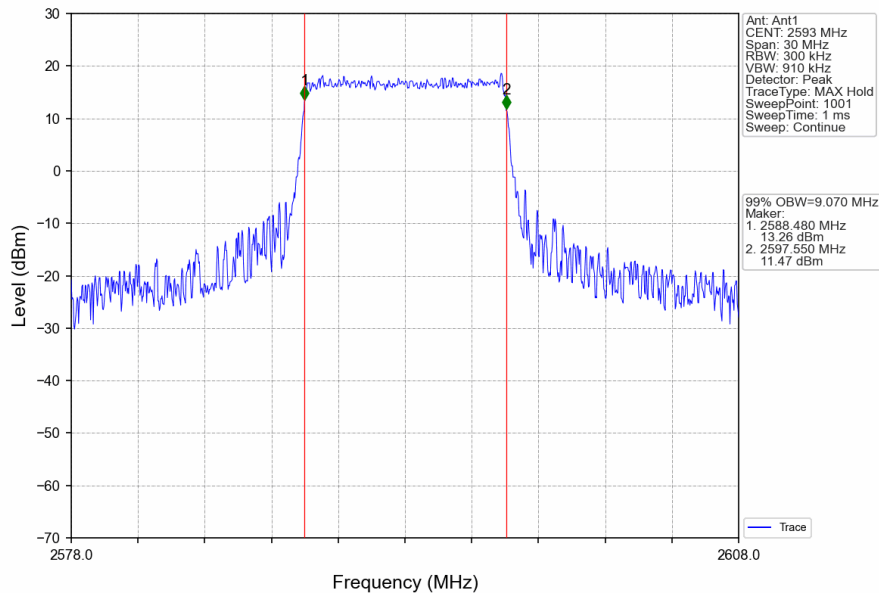
Band41_10MHz_QPSK_MCH_2593MHz_RB_50_0_NTNV
