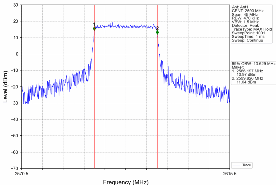
Band41_15MHz_QPSK_MCH_2593MHz_RB_75_0_NTNV
