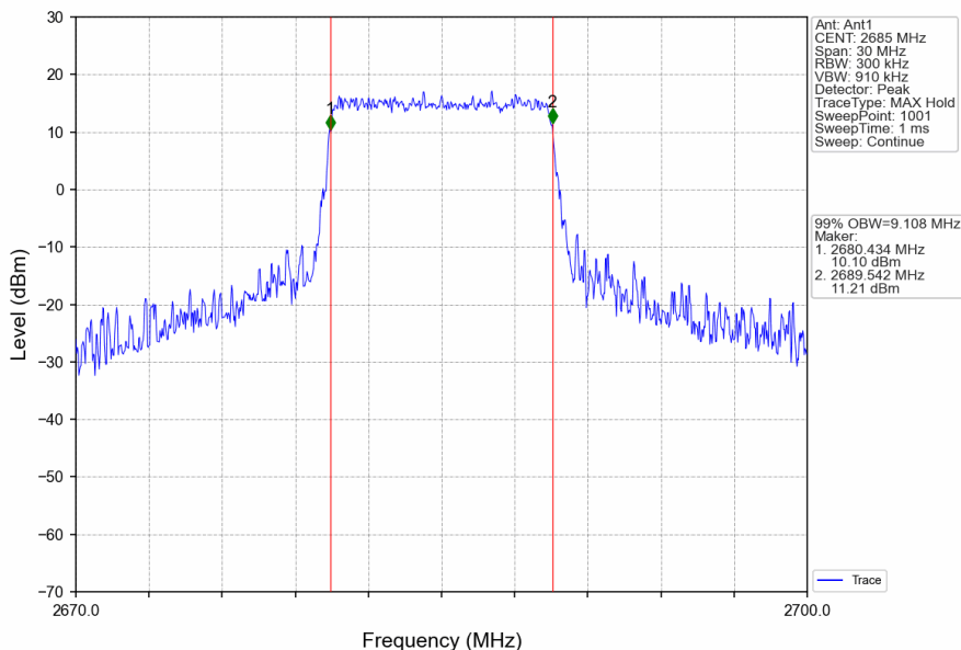
Band41_10MHz_16QAM_HCH_2685MHz_RB_50_0_NTNV
