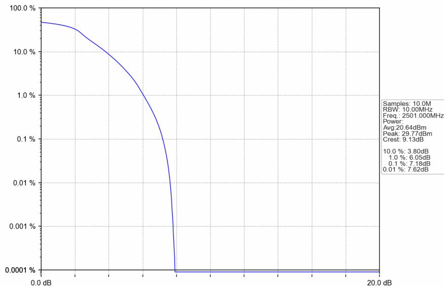
Band41_10MHz_QPSK_LCH_2501MHz_RB_50_0_NTNV
