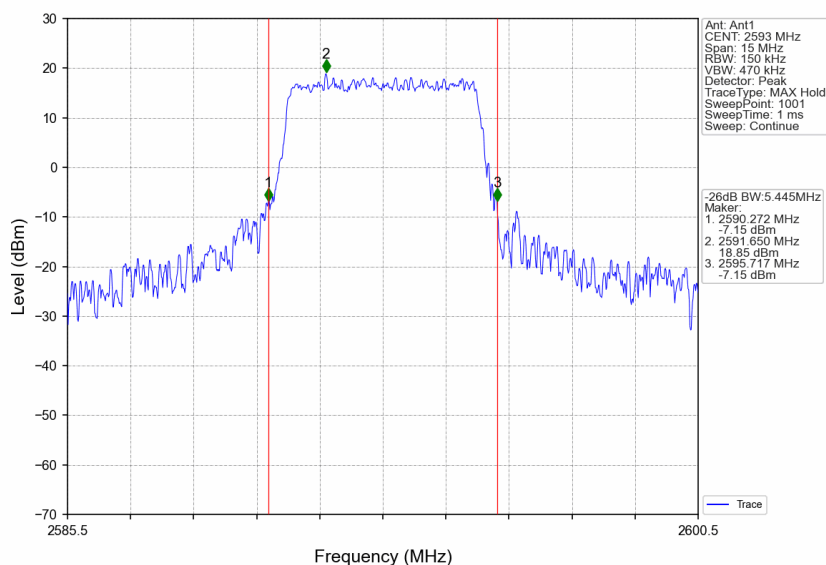
Band41_5MHz_QPSK_MCH_2593MHz_RB_25_0_NTNV
