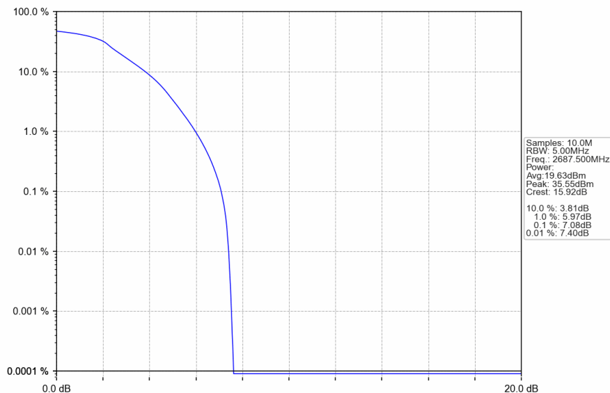
Band41_5MHz_QPSK_HCH_2687.5MHz_RB_25_0_NTNV
