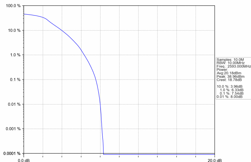
Band41_10MHz_QPSK_MCH_2593MHz_RB_50_0_NTNV
