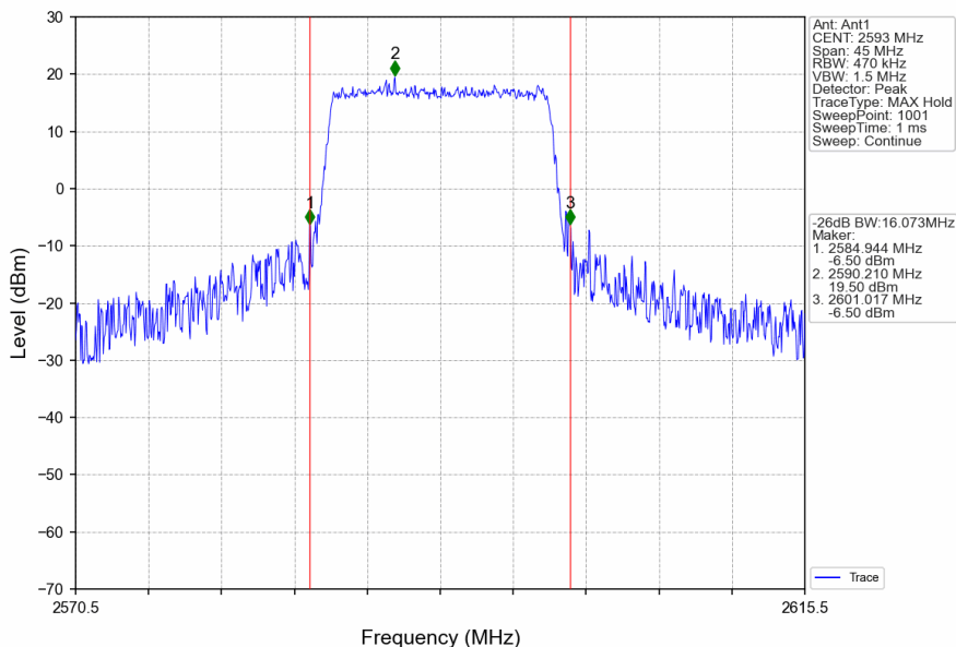
Band41_15MHz_QPSK_MCH_2593MHz_RB_75_0_NTNV
