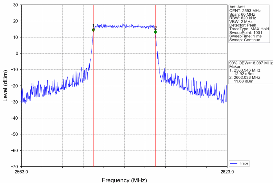
Band41_20MHz_QPSK_MCH_2593MHz_RB_100_0_NTNV
