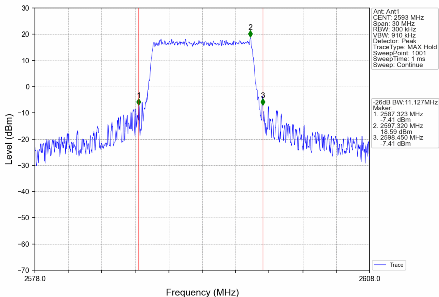
Band41_10MHz_QPSK_MCH_2593MHz_RB_50_0_NTNV
