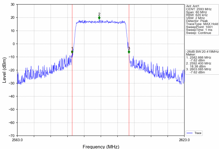
Band41_20MHz_QPSK_MCH_2593MHz_RB_100_0_NTNV
