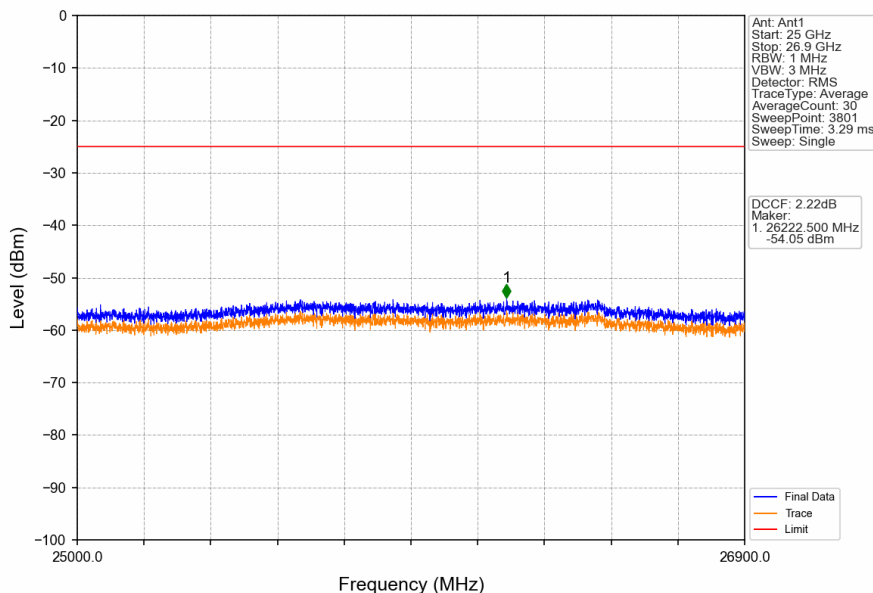
Band41_10MHz_QPSK_LCH_2501MHz_RB_1_0_NTNV
