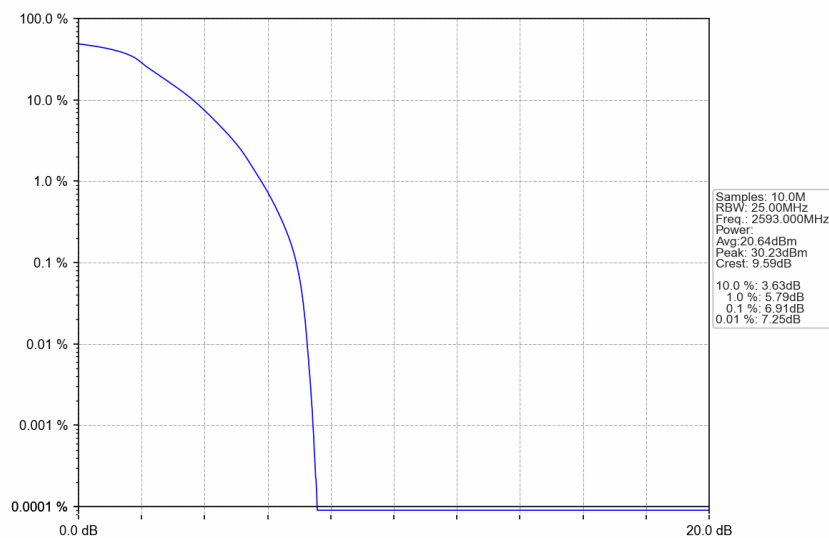
Band41_20MHz_QPSK_MCH_2593MHz_RB_100_0_NTNV
