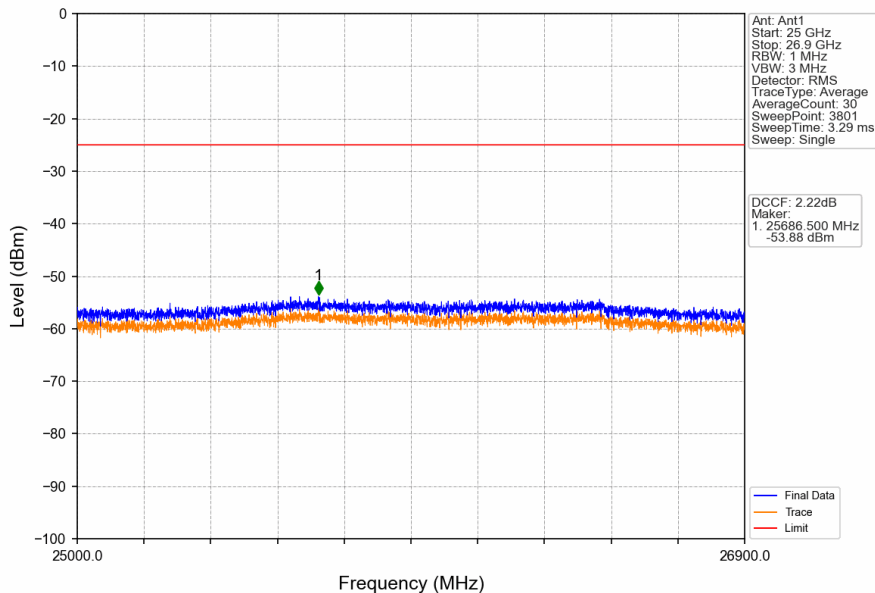
Band41_10MHz_16QAM_HCH_2685MHz_RB_1_0_NTNV
