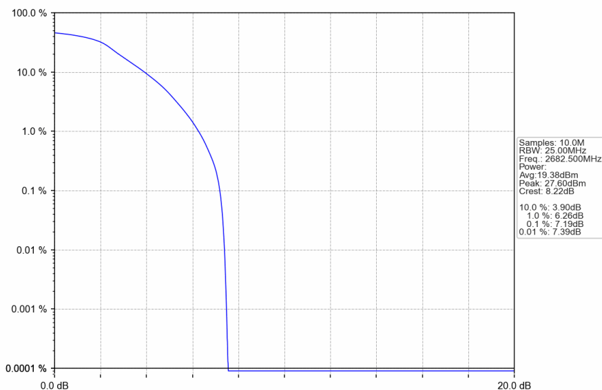
Band41_15MHz_QPSK_HCH_2682.5MHz_RB_75_0_NTNV
