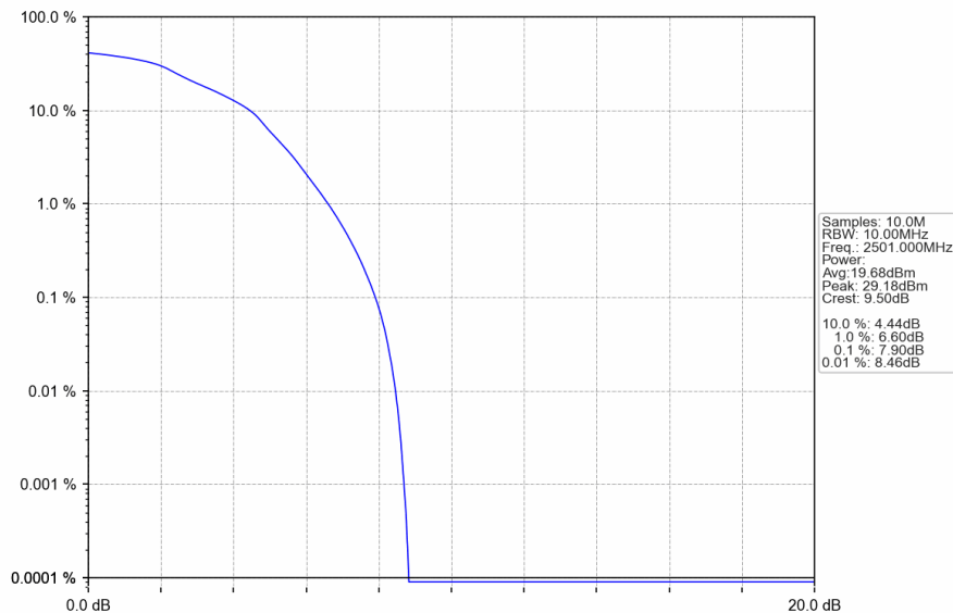
Band41_10MHz_16QAM_LCH_2501MHz_RB_50_0_NTNV
