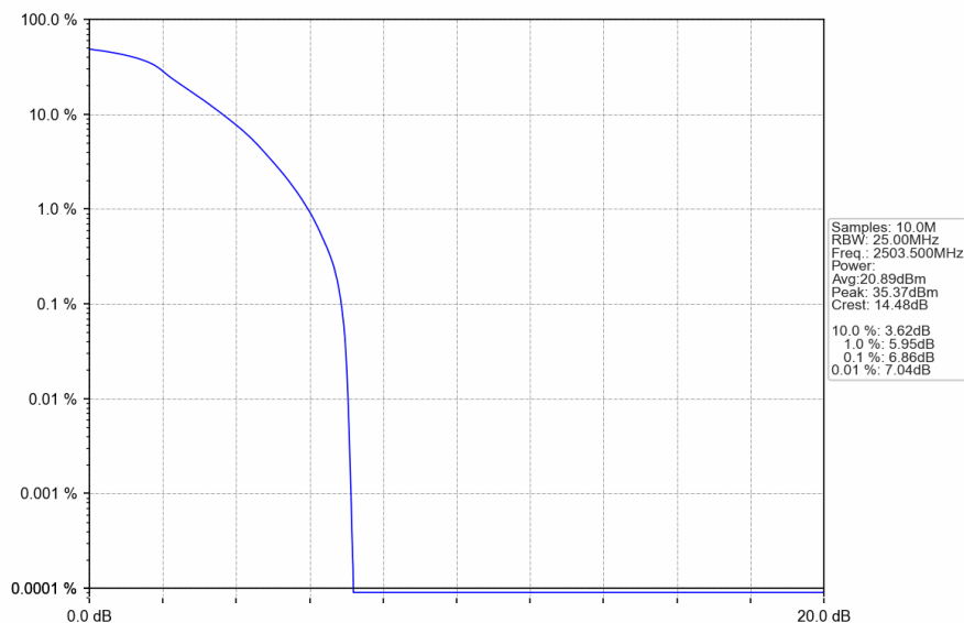
Band41_15MHz_QPSK_LCH_2503.5MHz_RB_75_0_NTNV
