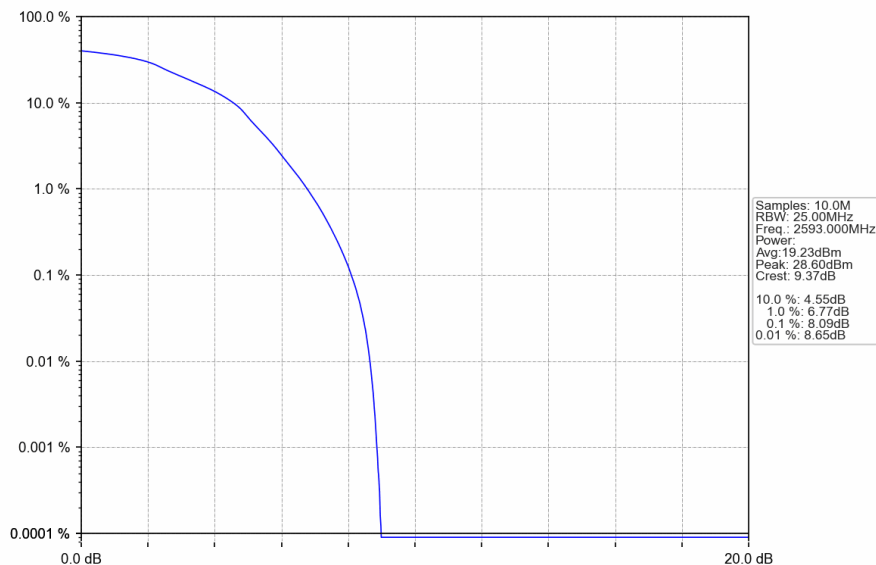
Band41_20MHz_16QAM_MCH_2593MHz_RB_100_0_NTNV
