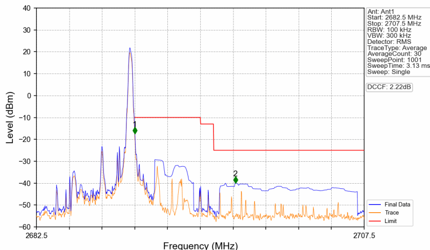
Band41_5MHz_QPSK_HCH_2687.5MHz_RB_1_24_NTNV
