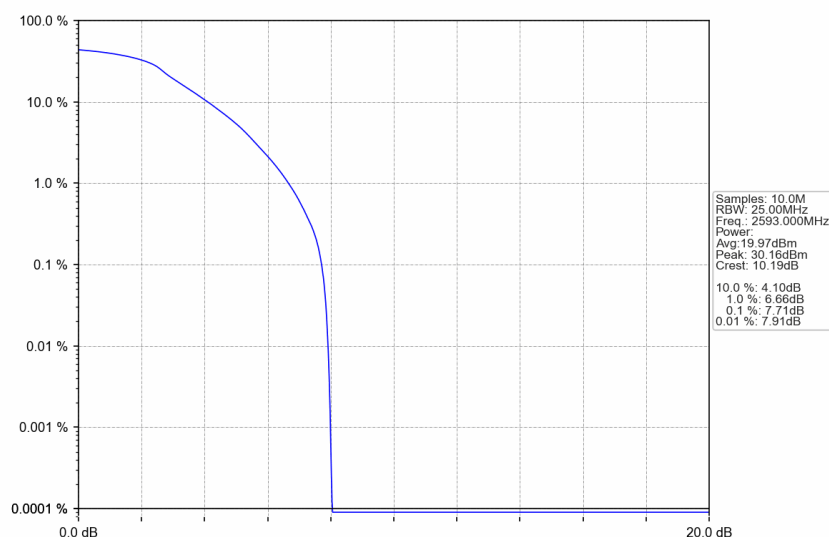
Band41_15MHz_QPSK_MCH_2593MHz_RB_75_0_NTNV
