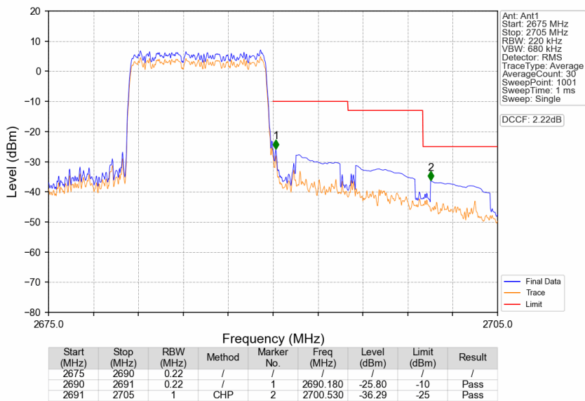
Band41_10MHz_16QAM_HCH_2685MHz_RB_50_0_NTNV
