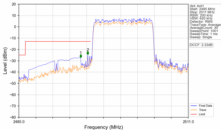
Band41_10MHz_16QAM_LCH_2501MHz_RB_50_0_NTNV
