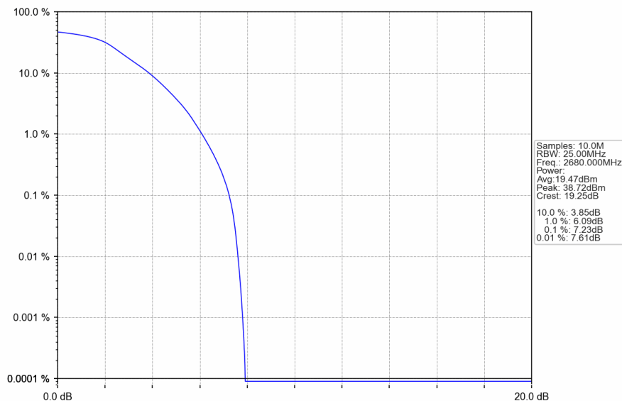
Band41_20MHz_QPSK_HCH_2680MHz_RB_100_0_NTNV
