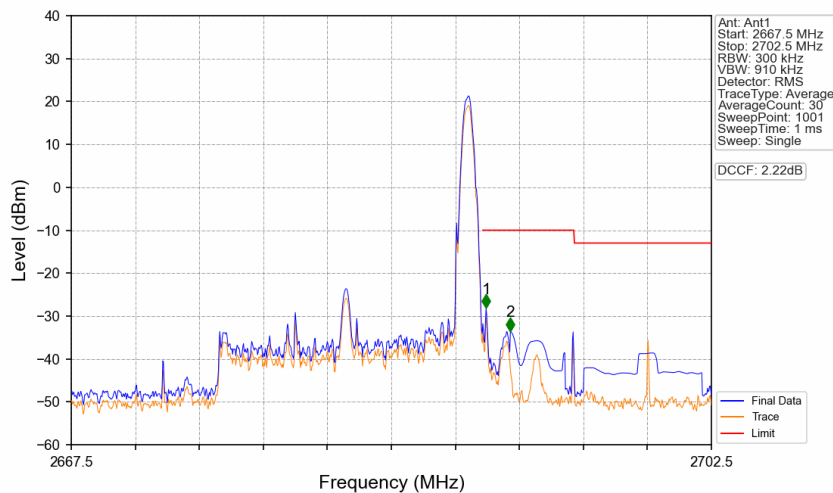
Band41_15MHz_QPSK_HCH_2682.5MHz_RB_1_74_NTNV
