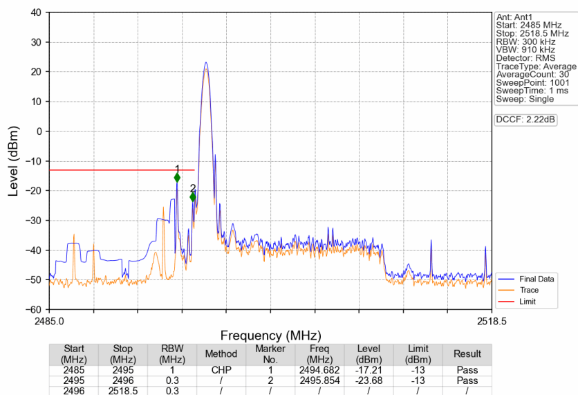
Band41_15MHz_QPSK_LCH_2503.5MHz_RB_1_0_NTNV
