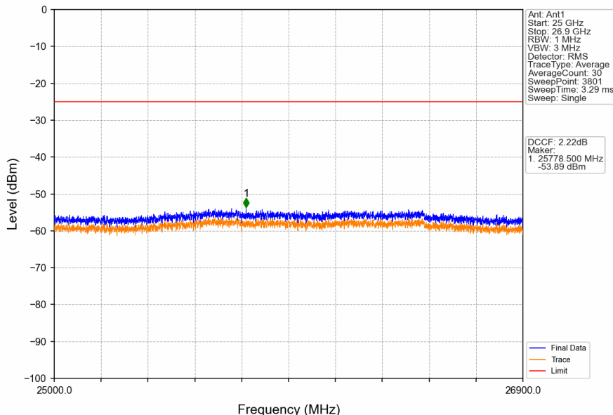
Band41_15MHz_QPSK_HCH_2682.5MHz_RB_1_74_NTNV
