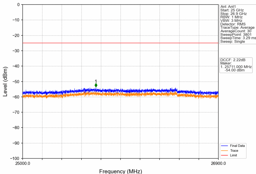
Band41_15MHz_QPSK_LCH_2503.5MHz_RB_1_0_NTNV
