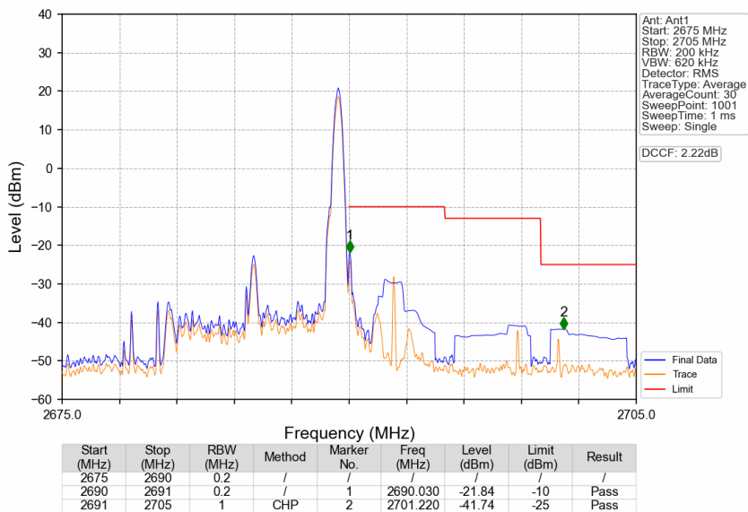
Band41_10MHz_16QAM_HCH_2685MHz_RB_1_49_NTNV
