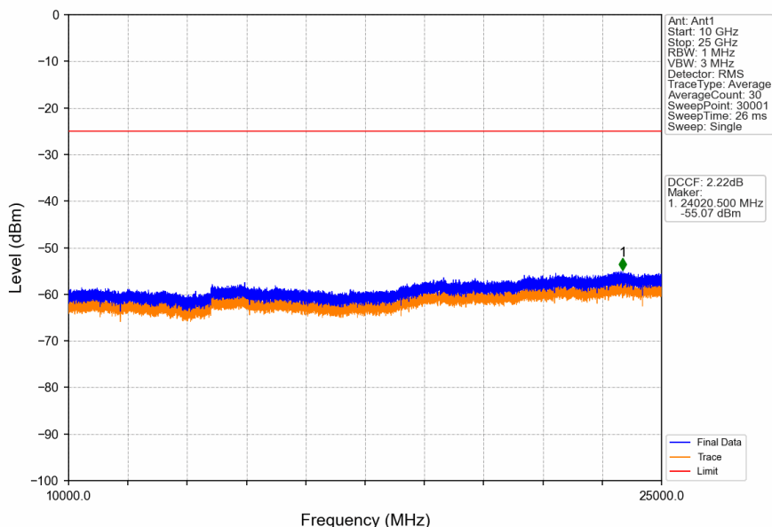
Band41_5MHz_QPSK_MCH_2593MHz_RB_1_0_NTNV
