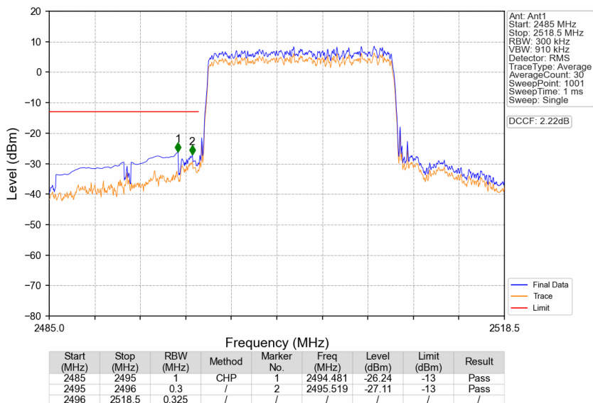
Band41_15MHz_QPSK_LCH_2503.5MHz_RB_75_0_NTNV
