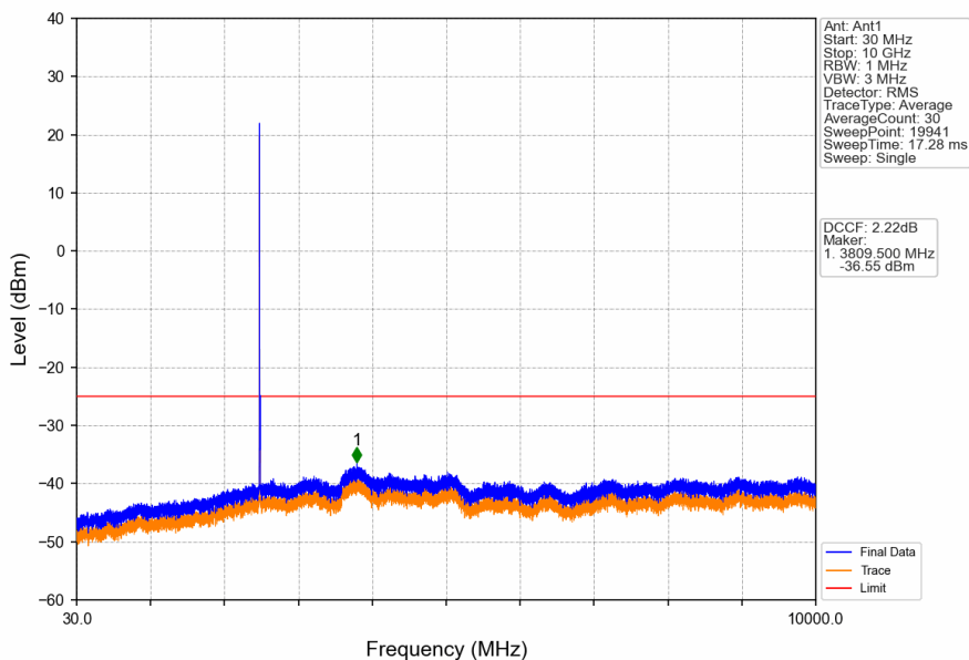
Band41_10MHz_16QAM_LCH_2501MHz_RB_1_0_NTNV
