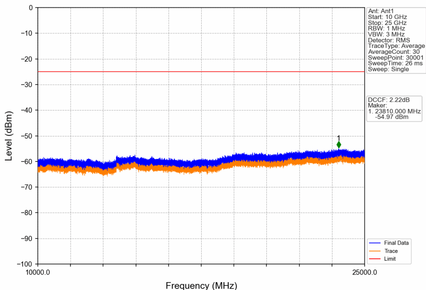
Band41_10MHz_QPSK_HCH_2685MHz_RB_1_0_NTNV
