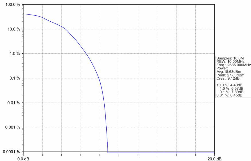
Band41_10MHz_16QAM_HCH_2685MHz_RB_50_0_NTNV
