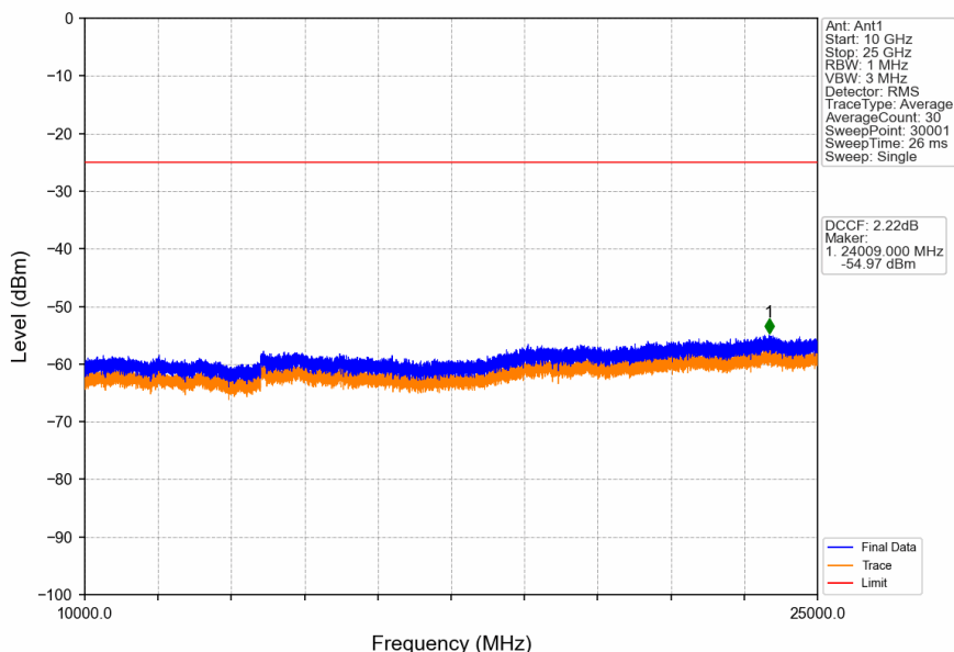
Band41_10MHz_QPSK_MCH_2593MHz_RB_1_0_NTNV
