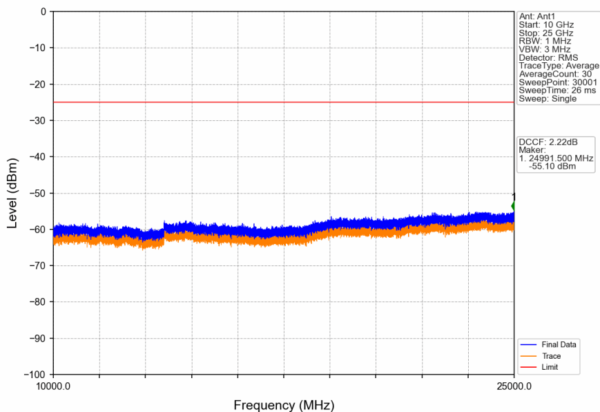
Band41_10MHz_16QAM_HCH_2685MHz_RB_1_0_NTNV
