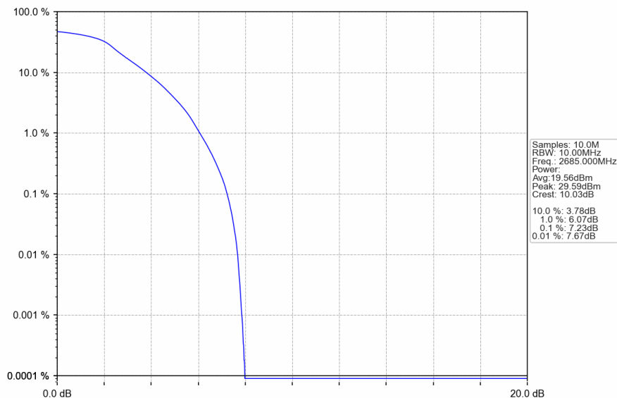
Band41_10MHz_QPSK_HCH_2685MHz_RB_50_0_NTNV
