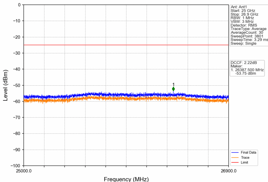
Band41_10MHz_QPSK_MCH_2593MHz_RB_1_0_NTNV
