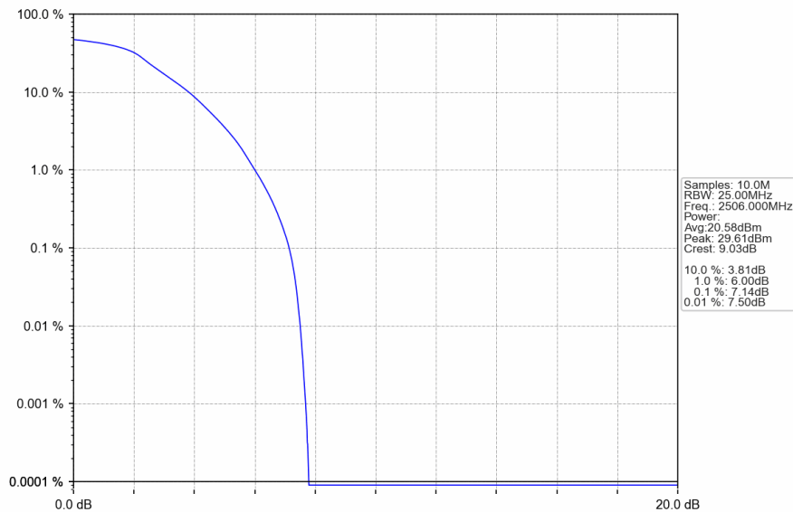
Band41_20MHz_QPSK_LCH_2506MHz_RB_100_0_NTNV
