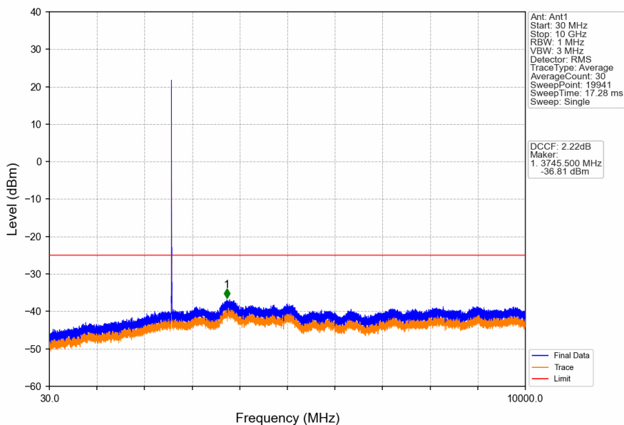
Band41_10MHz_16QAM_MCH_2593MHz_RB_1_0_NTNV
