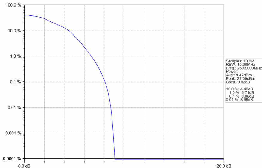
Band41_10MHz_16QAM_MCH_2593MHz_RB_50_0_NTNV
