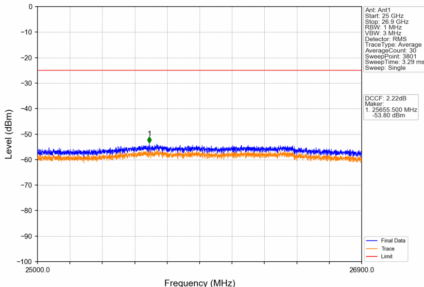
Band41_10MHz_QPSK_HCH_2685MHz_RB_1_49_NTNV
