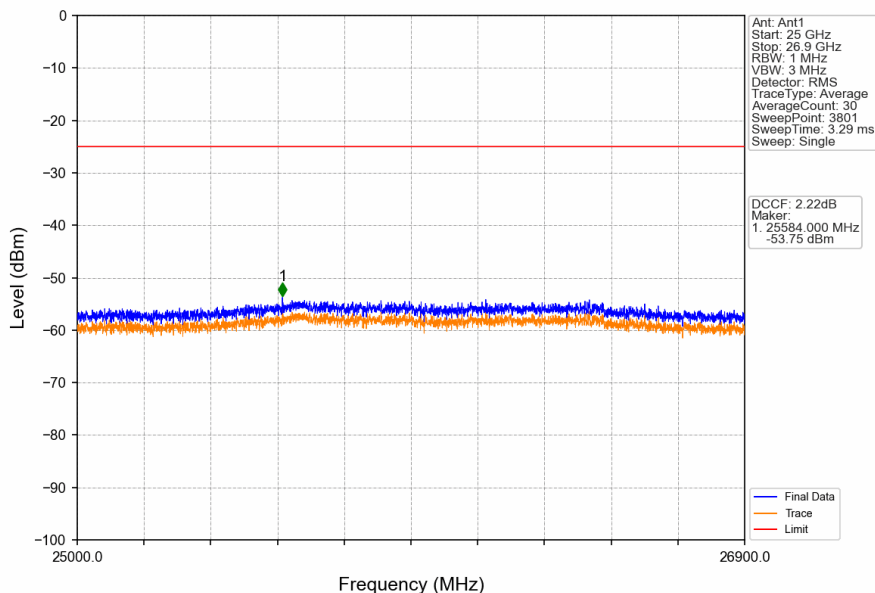
Band41_5MHz_QPSK_LCH_2498.5MHz_RB_1_0_NTNV
