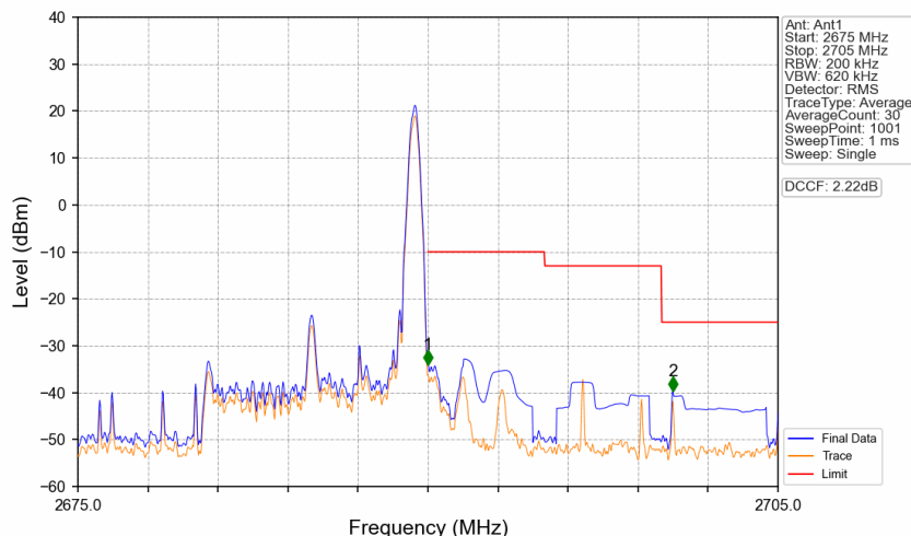
Band41_10MHz_QPSK_HCH_2685MHz_RB_1_49_NTNV
