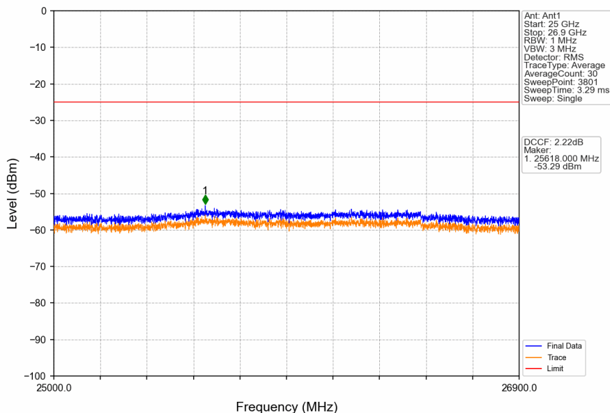
Band41_5MHz_QPSK_MCH_2593MHz_RB_1_0_NTNV
