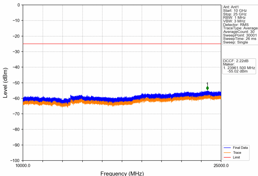
Band41_15MHz_QPSK_LCH_2503.5MHz_RB_1_0_NTNV
