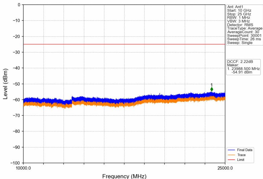
Band41_15MHz_QPSK_HCH_2682.5MHz_RB_1_0_NTNV
