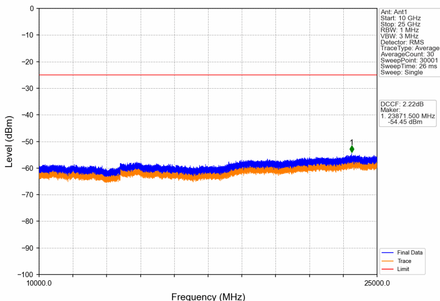
Band41_15MHz_QPSK_MCH_2593MHz_RB_1_0_NTNV
