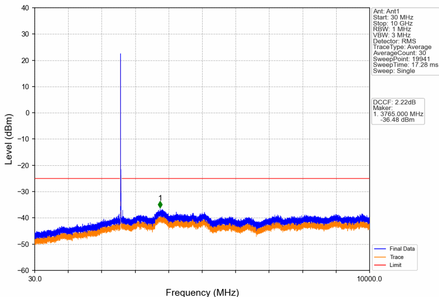
Band41_15MHz_QPSK_MCH_2593MHz_RB_1_0_NTNV
