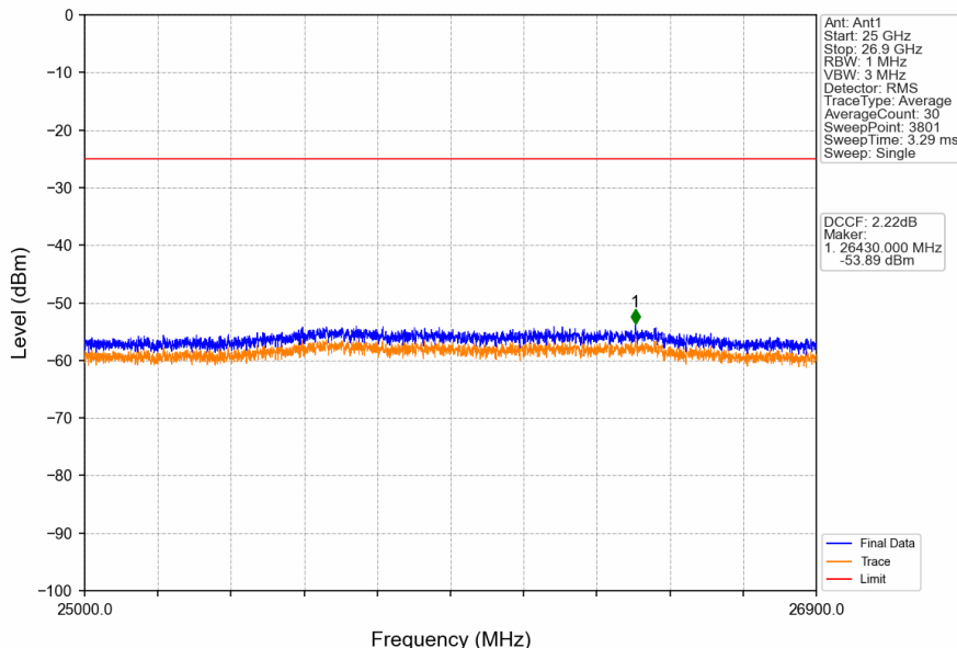
Band41_5MHz_QPSK_HCH_2687.5MHz_RB_1_24_NTNV
