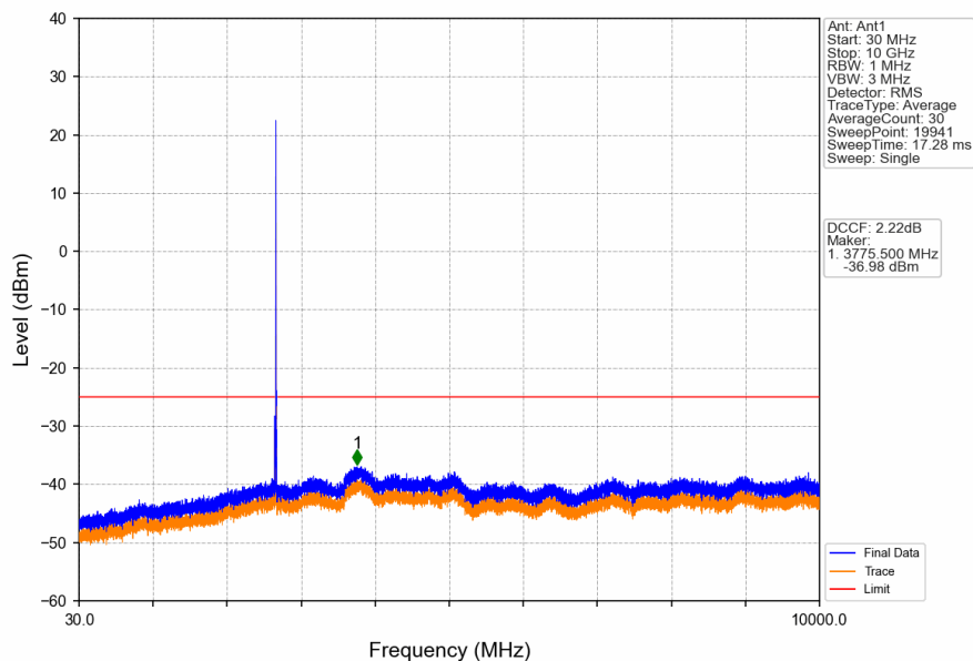
Band41_10MHz_QPSK_HCH_2685MHz_RB_1_0_NTNV
