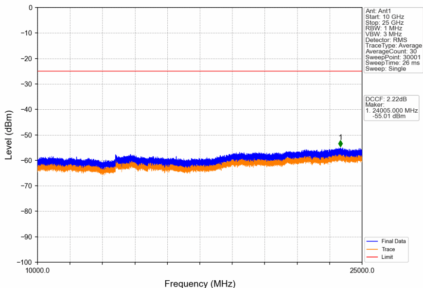
Band41_10MHz_16QAM_LCH_2501MHz_RB_1_0_NTNV
