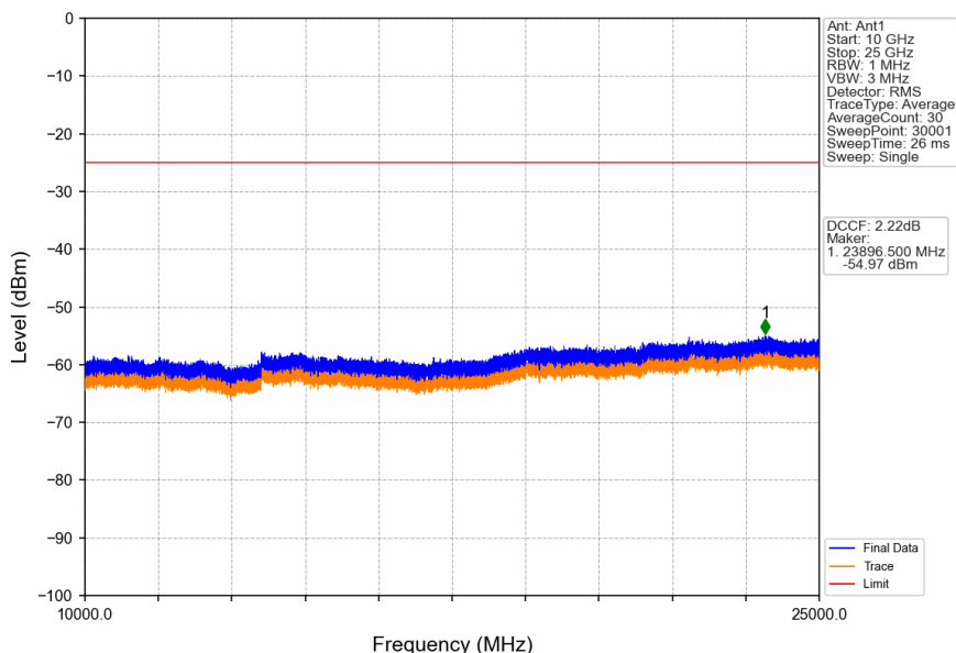
Band41_10MHz_QPSK_LCH_2501MHz_RB_1_0_NTNV
