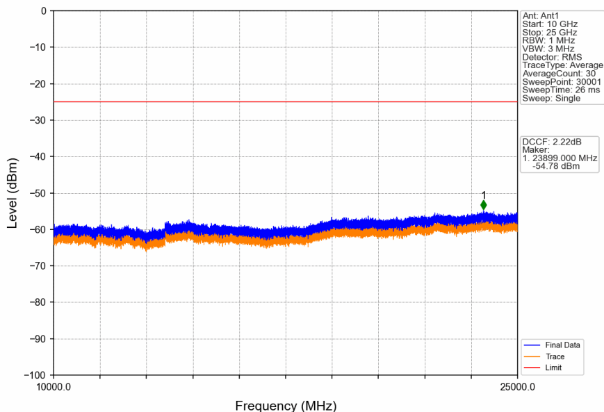
Band41_10MHz_16QAM_MCH_2593MHz_RB_1_0_NTNV
