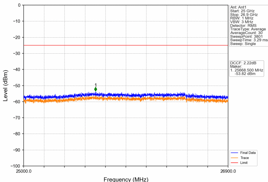
Band41_20MHz_QPSK_HCH_2680MHz_RB_1_99_NTNV
