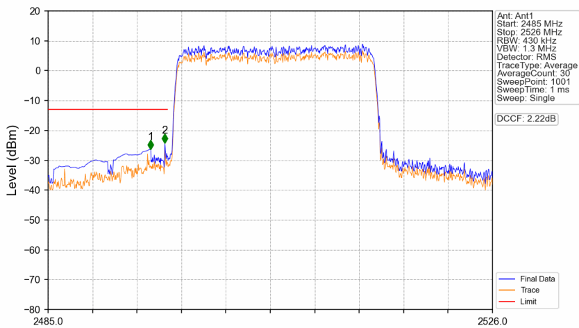
Band41_20MHz_QPSK_LCH_2506MHz_RB_100_0_NTNV
