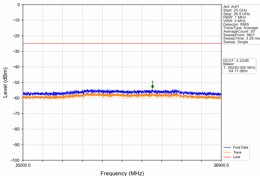
Band41_20MHz_QPSK_LCH_2506MHz_RB_1_0_NTNV
