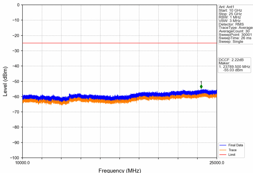
Band41_20MHz_QPSK_LCH_2506MHz_RB_1_0_NTNV
