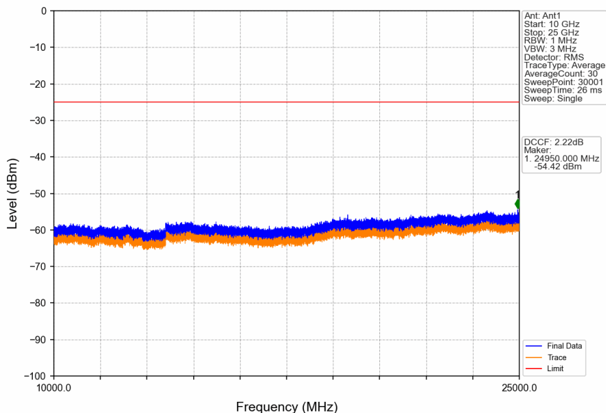
Band41_20MHz_QPSK_HCH_2680MHz_RB_1_0_NTNV
