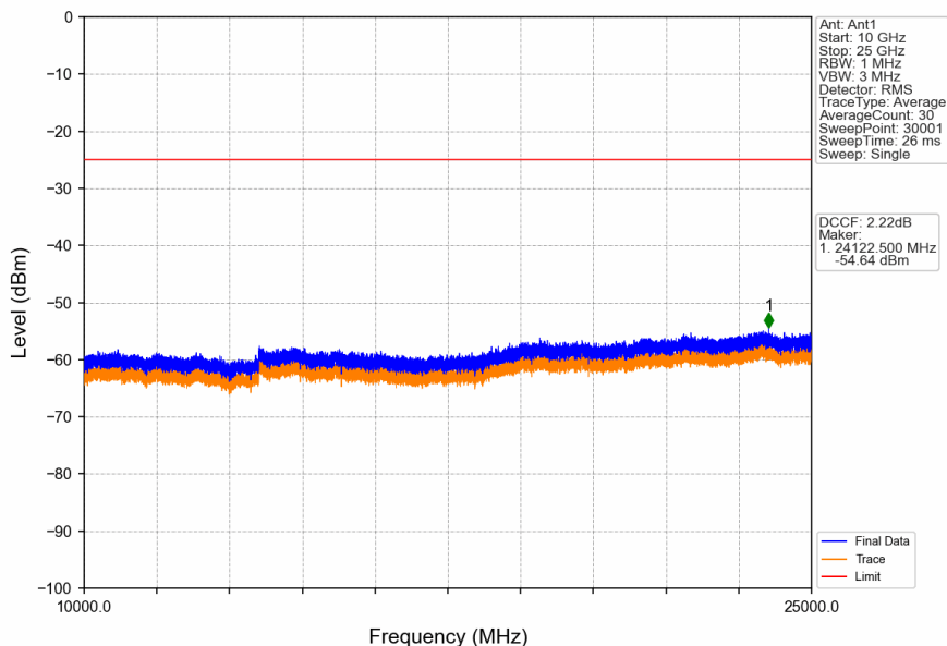
Band41_20MHz_16QAM_MCH_2593MHz_RB_1_0_NTNV
