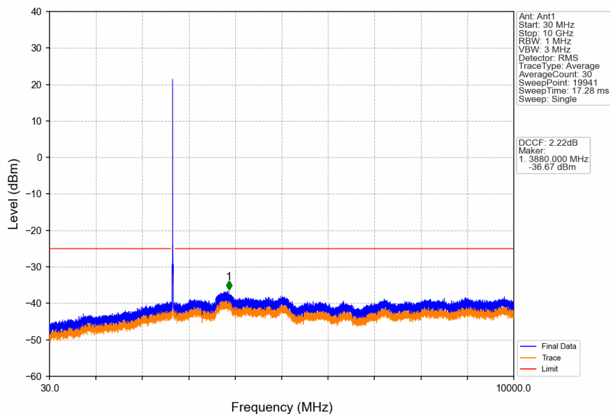
Band41_20MHz_QPSK_HCH_2680MHz_RB_1_0_NTNV
