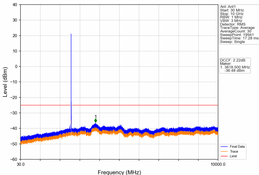
Band41_20MHz_QPSK_MCH_2593MHz_RB_1_0_NTNV
