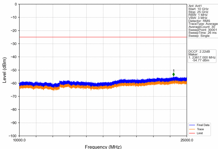
Band41_20MHz_QPSK_MCH_2593MHz_RB_1_0_NTNV
