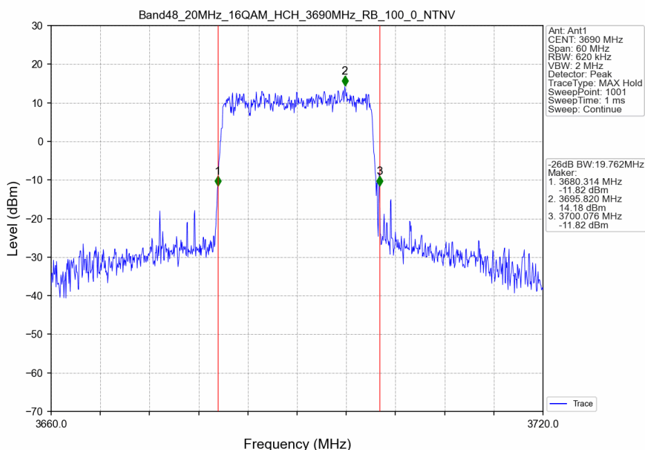
Band48_20MHz_16QAM_HCH_3690MHz_RB_100_0_NTNV
