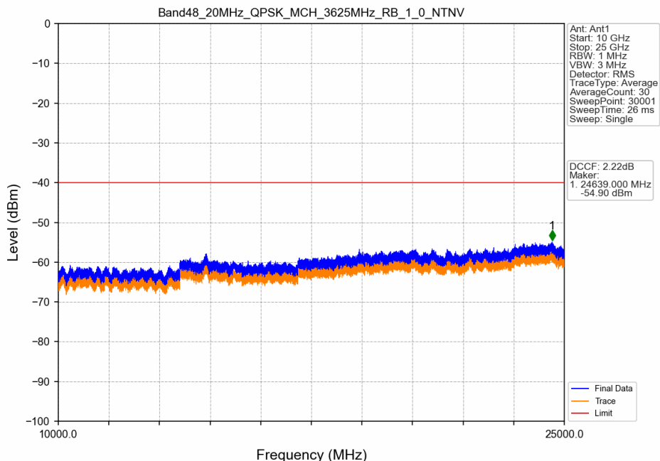
Band48_20MHz_QPSK_MCH_3625MHz_RB_1_0_NTNV
