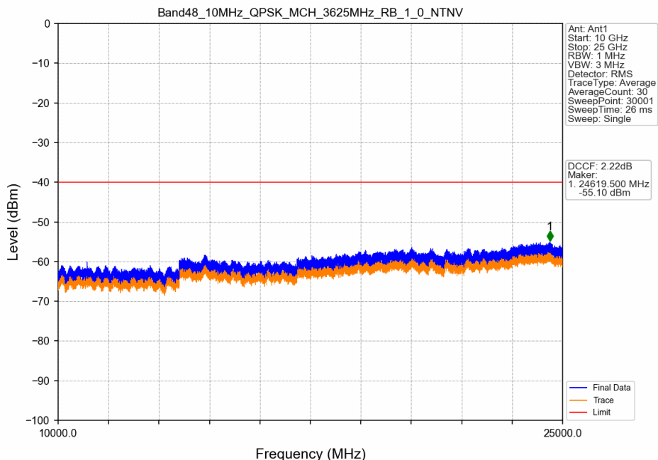
Band48_10MHz_QPSK_MCH_3625MHz_RB_1_0_NTNV
