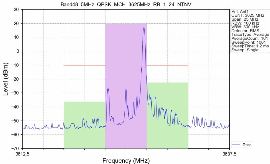
Band48_5MHz_QPSK_MCH_3625MHz_RB_1_24_NTNV
