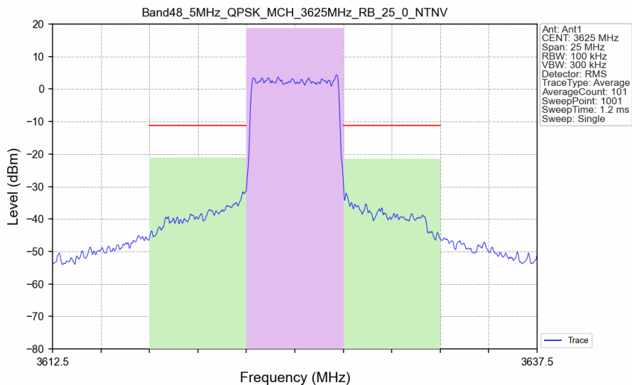
Band48_5MHz_QPSK_MCH_3625MHz_RB_25_0_NTNV
