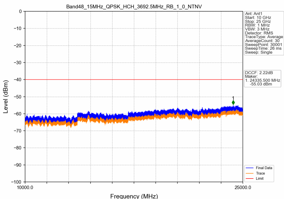
Band48_15MHz_QPSK_HCH_3692.5MHz_RB_1_0_NTNV
