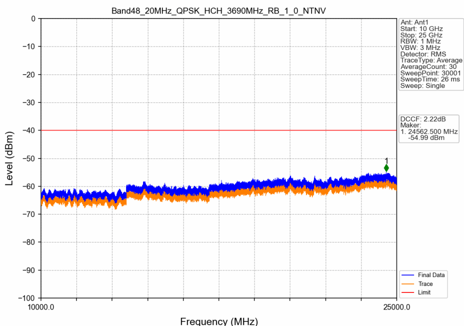
Band48_20MHz_QPSK_HCH_3690MHz_RB_1_0_NTNV
