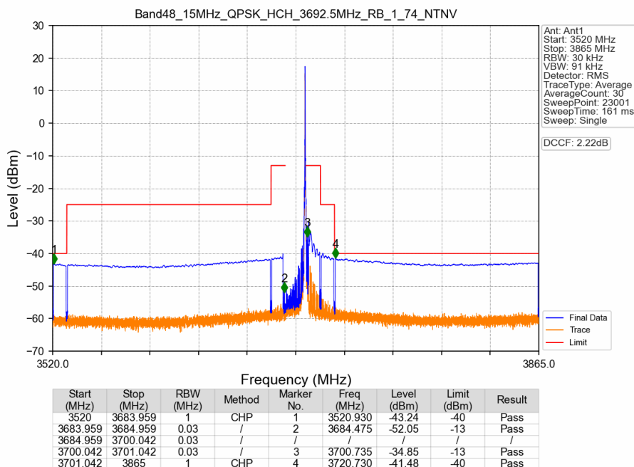
Band48_15MHz_QPSK_HCH_3692.5MHz_RB_1_74_NTNV
