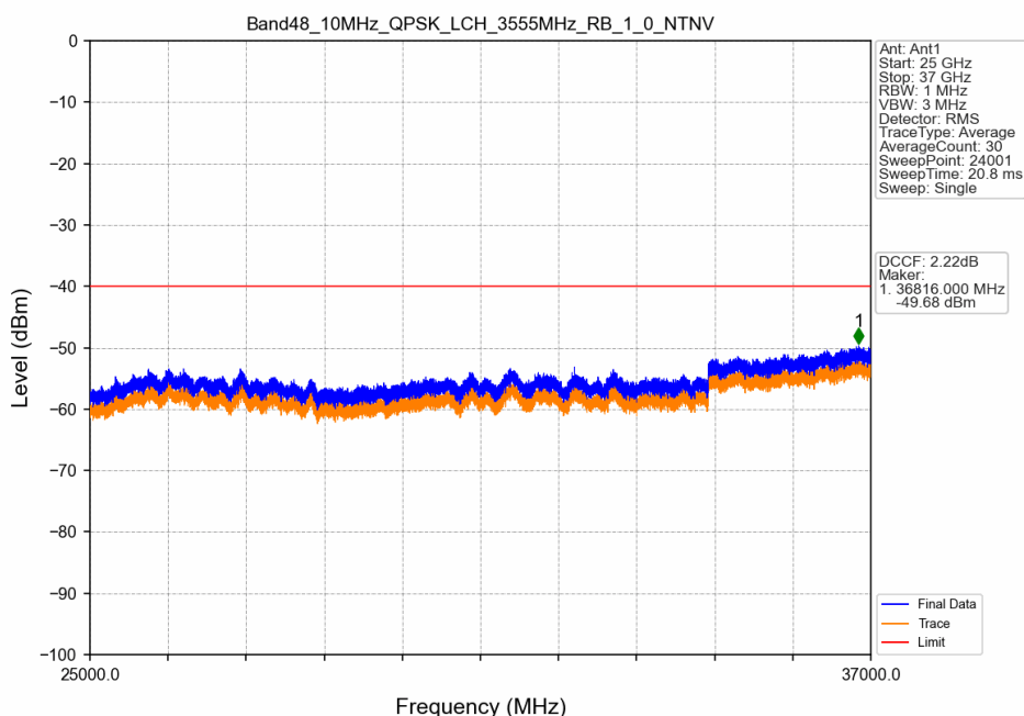
Band48_10MHz_QPSK_LCH_3555MHz_RB_1_0_NTNV
