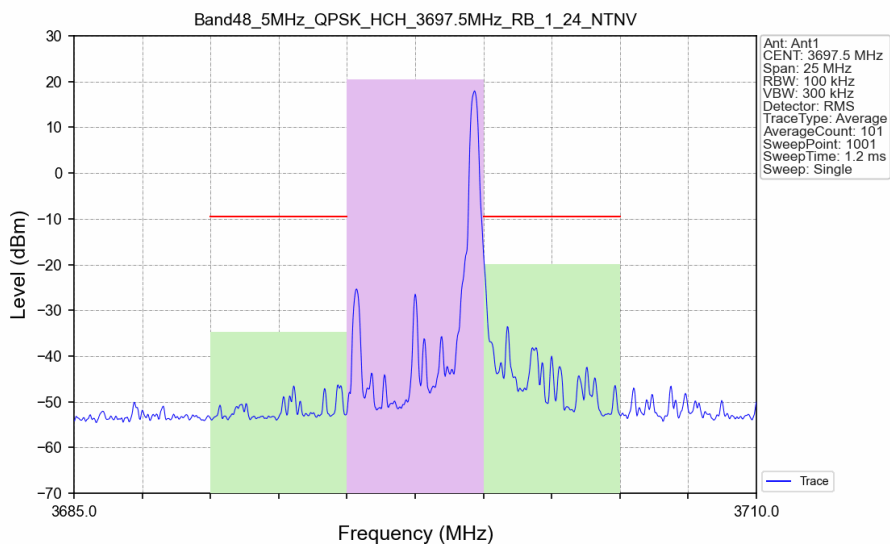
Band48_5MHz_QPSK_HCH_3697.5MHz_RB_1_24_NTNV
