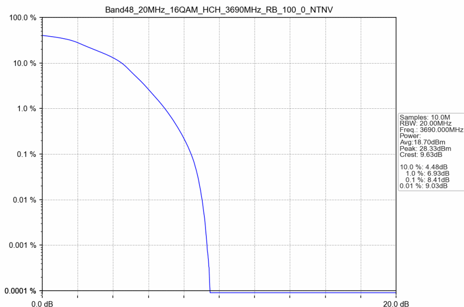
Band48_20MHz_16QAM_HCH_3690MHz_RB_100_0_NTNV
