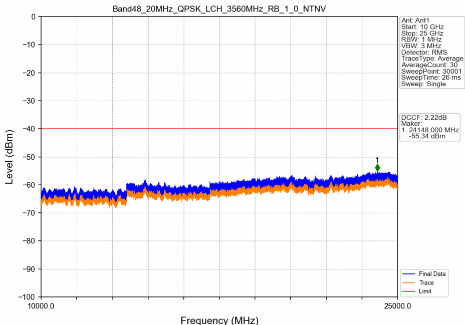
Band48_20MHz_QPSK_LCH_3560MHz_RB_1_0_NTNV
