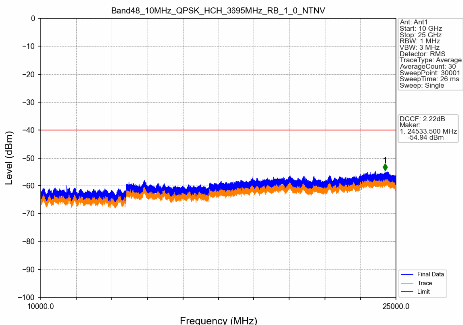
Band48_10MHz_QPSK_HCH_3695MHz_RB_1_0_NTNV
