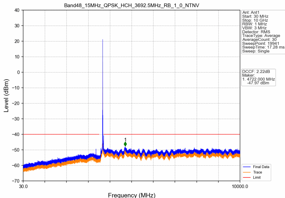
Band48_15MHz_QPSK_HCH_3692.5MHz_RB_1_0_NTNV
