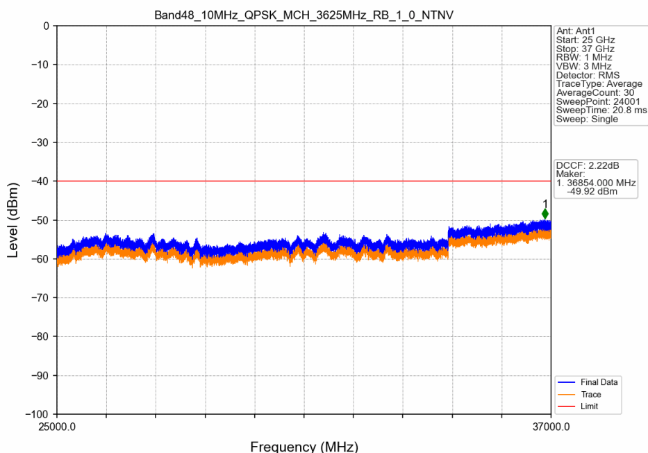
Band48_10MHz_QPSK_MCH_3625MHz_RB_1_0_NTNV
