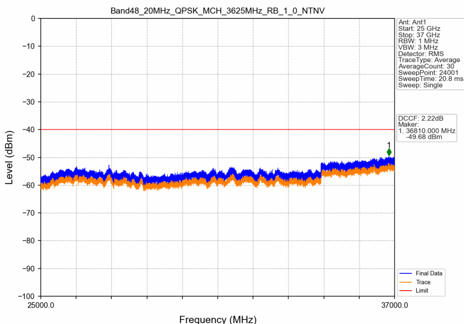
Band48_20MHz_QPSK_MCH_3625MHz_RB_1_0_NTNV
