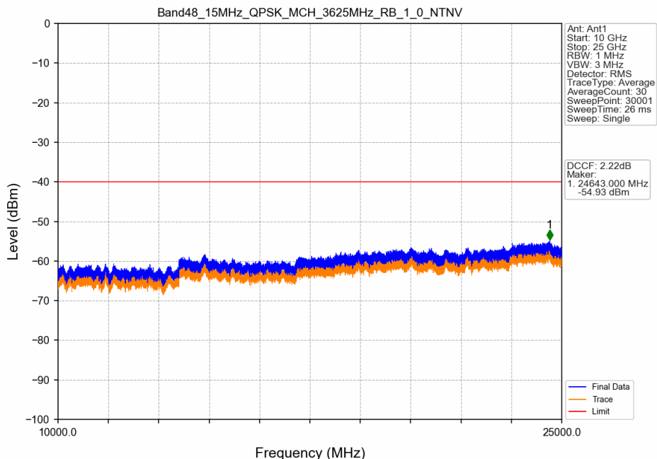
Band48_15MHz_QPSK_MCH_3625MHz_RB_1_0_NTNV
