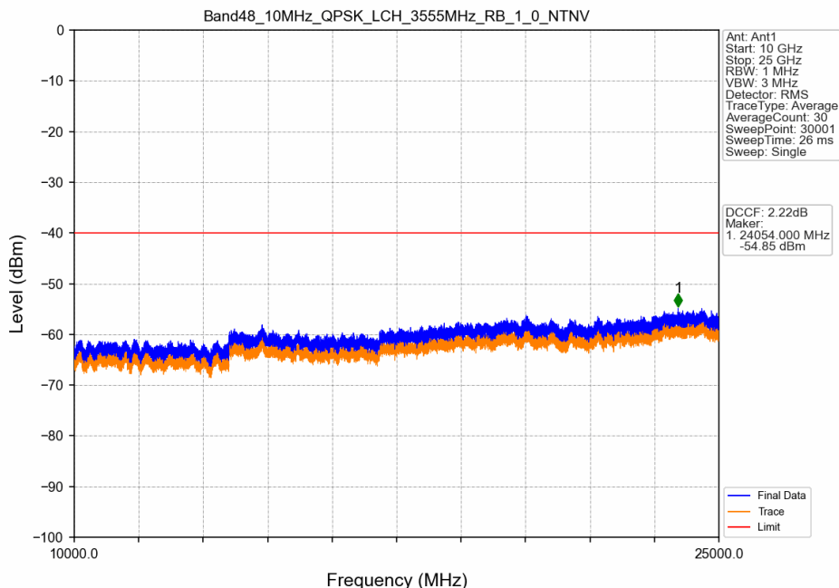
Band48_10MHz_QPSK_LCH_3555MHz_RB_1_0_NTNV
