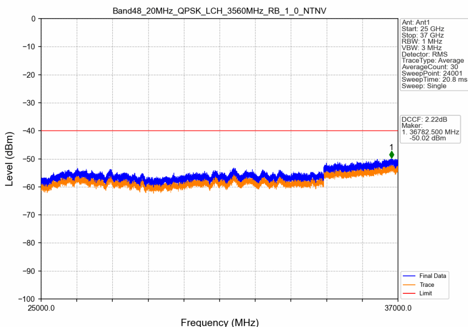
Band48_20MHz_QPSK_LCH_3560MHz_RB_1_0_NTNV
