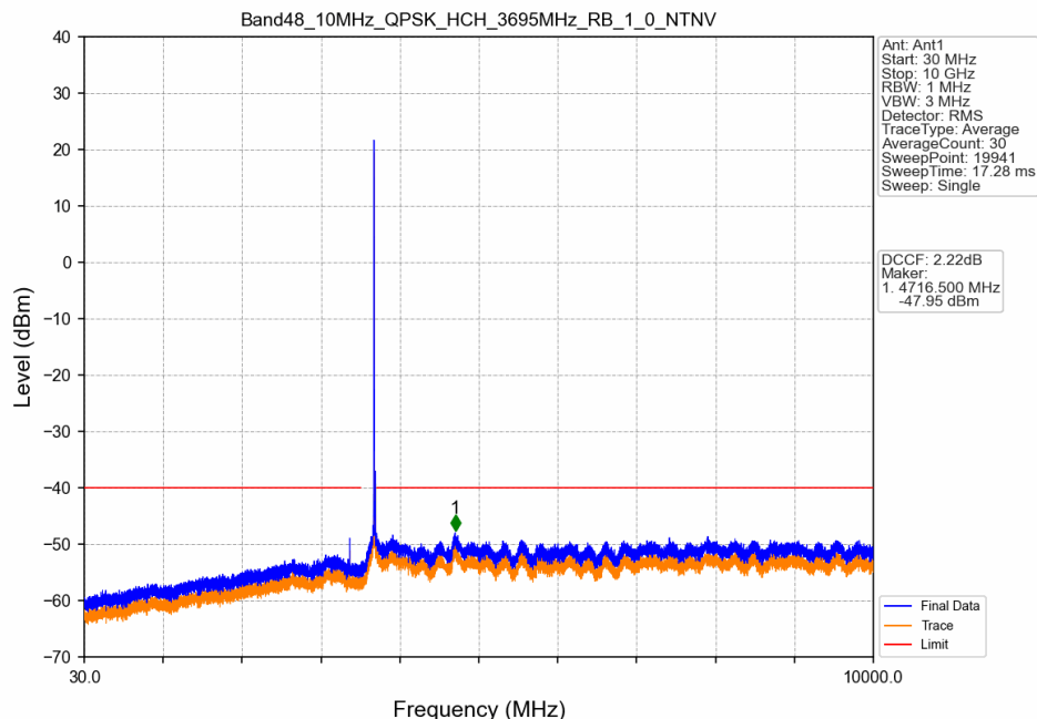
Band48_10MHz_QPSK_HCH_3695MHz_RB_1_0_NTNV
