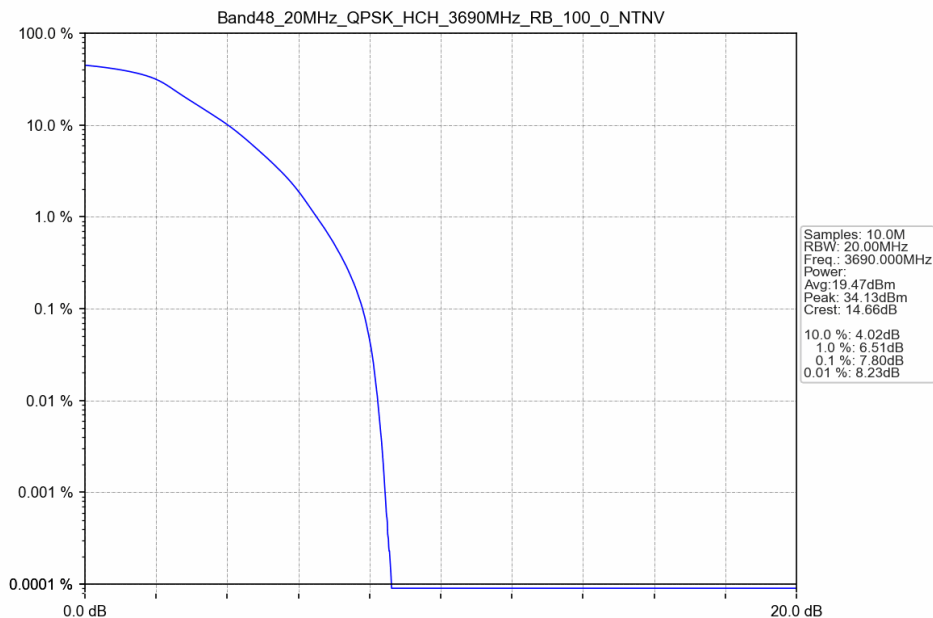
Band48_20MHz_QPSK_HCH_3690MHz_RB_100_0_NTNV
