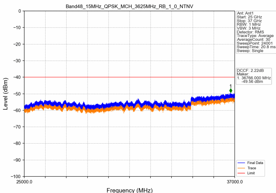
Band48_15MHz_QPSK_MCH_3625MHz_RB_1_0_NTNV
