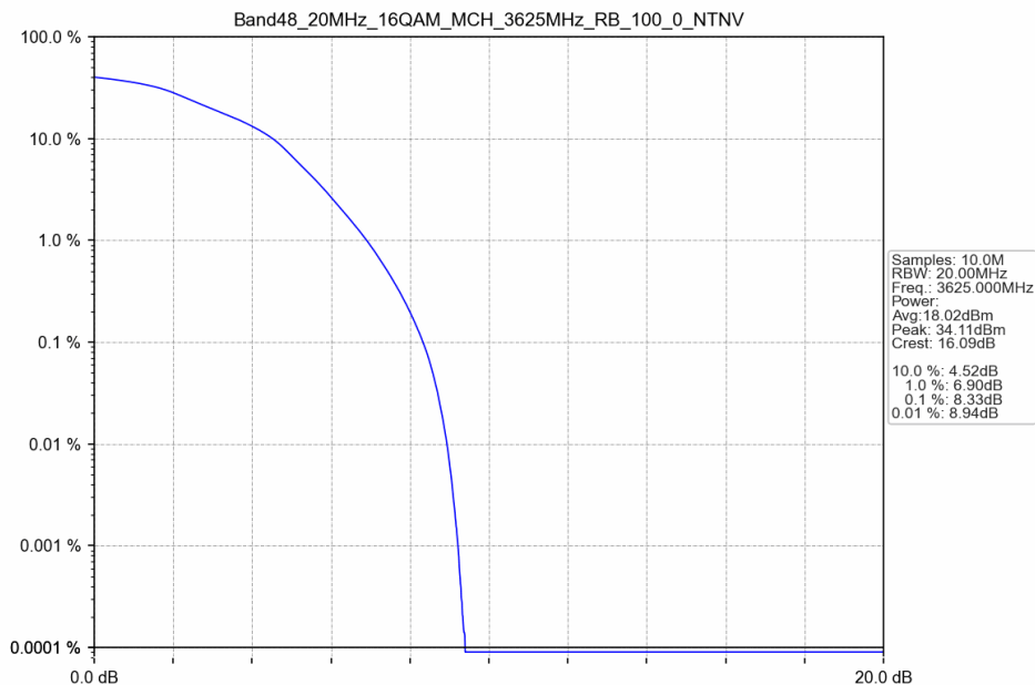
Band48_20MHz_16QAM_MCH_3625MHz_RB_100_0_NTNV
