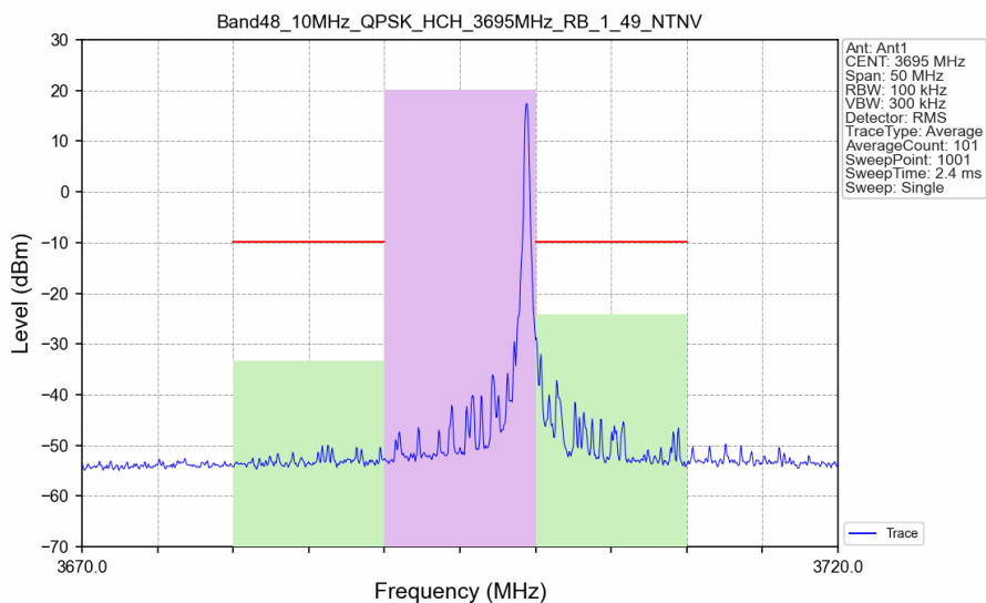
Band48_10MHz_QPSK_HCH_3695MHz_RB_1_49_NTNV
