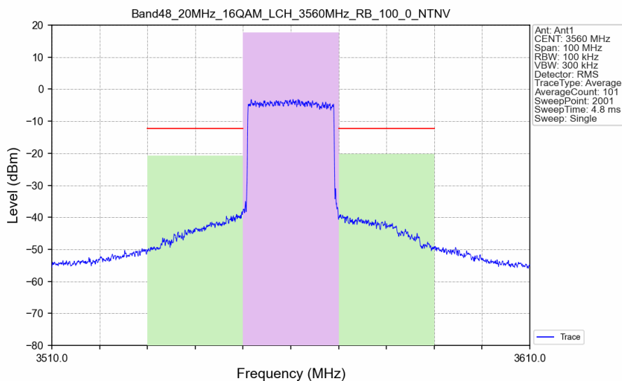
Band48_20MHz_16QAM_LCH_3560MHz_RB_100_0_NTNV
