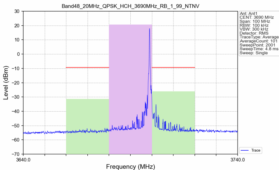
Band48_20MHz_QPSK_HCH_3690MHz_RB_1_99_NTNV
