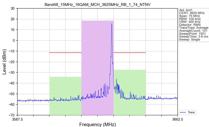
Band48_15MHz_16QAM_MCH_3625MHz_RB_1_74_NTNV
