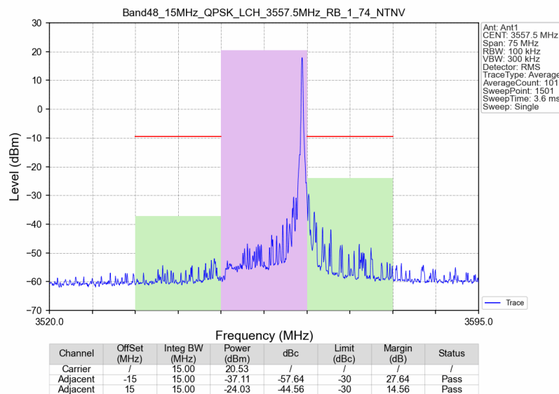
Band48_15MHz_QPSK_LCH_3557.5MHz_RB_1_74_NTNV
