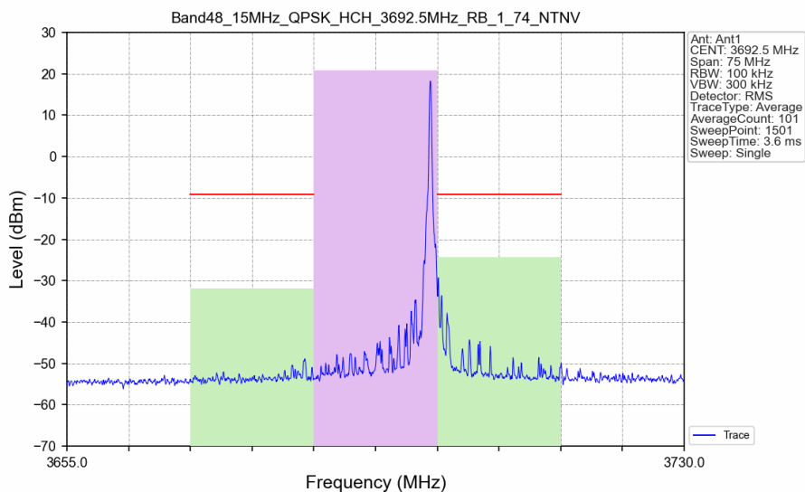
Band48_15MHz_QPSK_HCH_3692.5MHz_RB_1_74_NTNV
