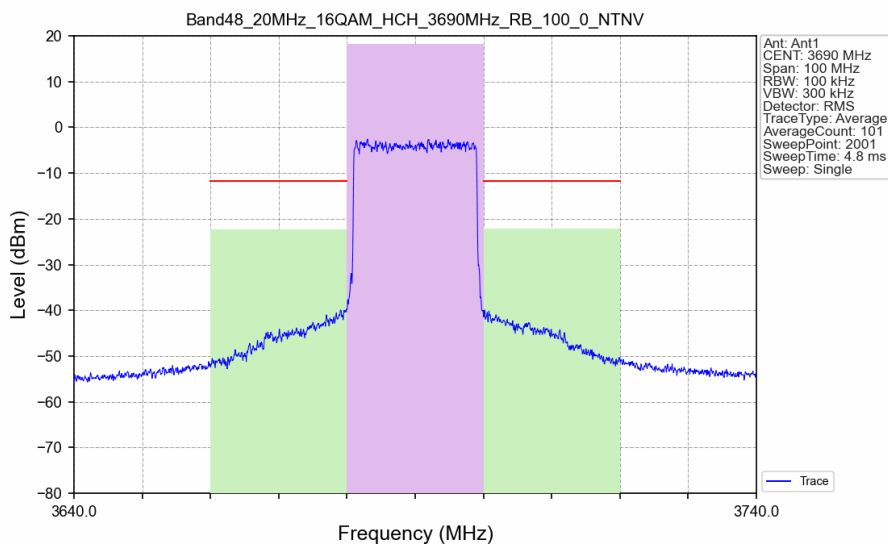
Band48_20MHz_16QAM_HCH_3690MHz_RB_100_0_NTNV
