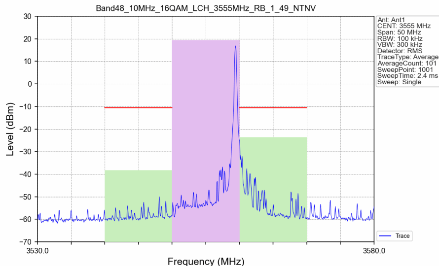
Band48_10MHz_16QAM_LCH_3555MHz_RB_1_49_NTNV
