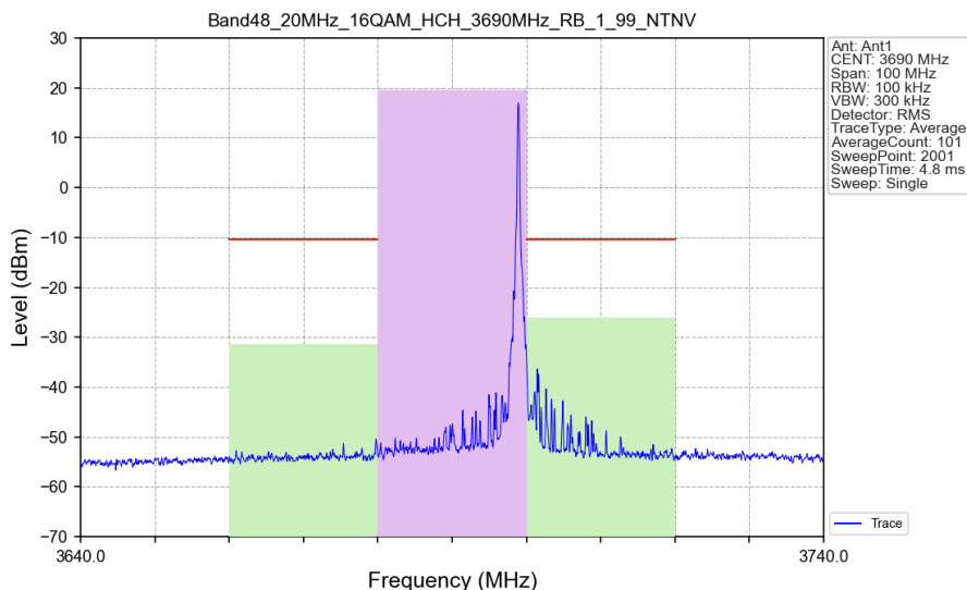
Band48_20MHz_16QAM_HCH_3690MHz_RB_1_99_NTNV
