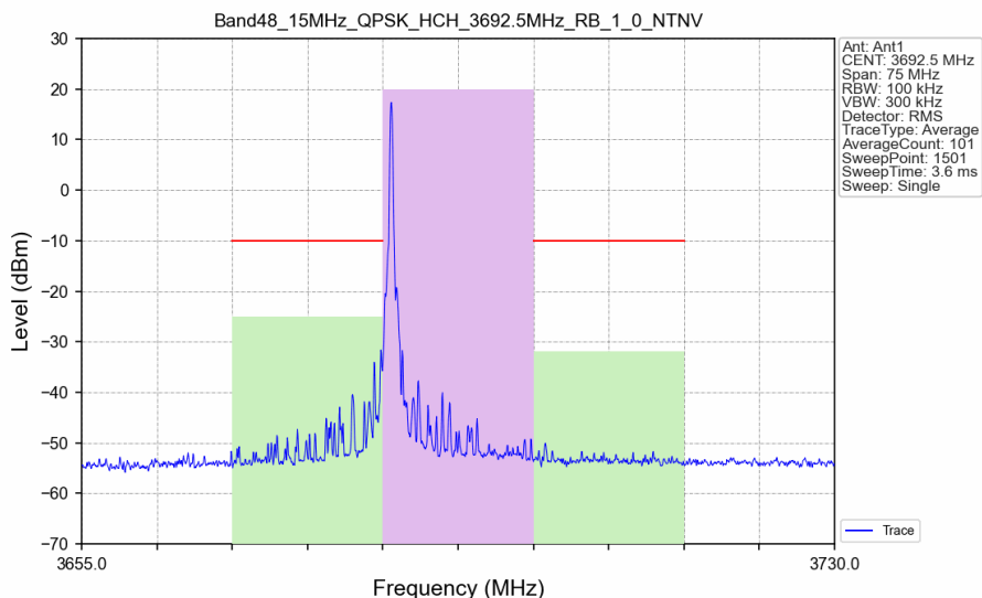
Band48_15MHz_QPSK_HCH_3692.5MHz_RB_1_0_NTNV
