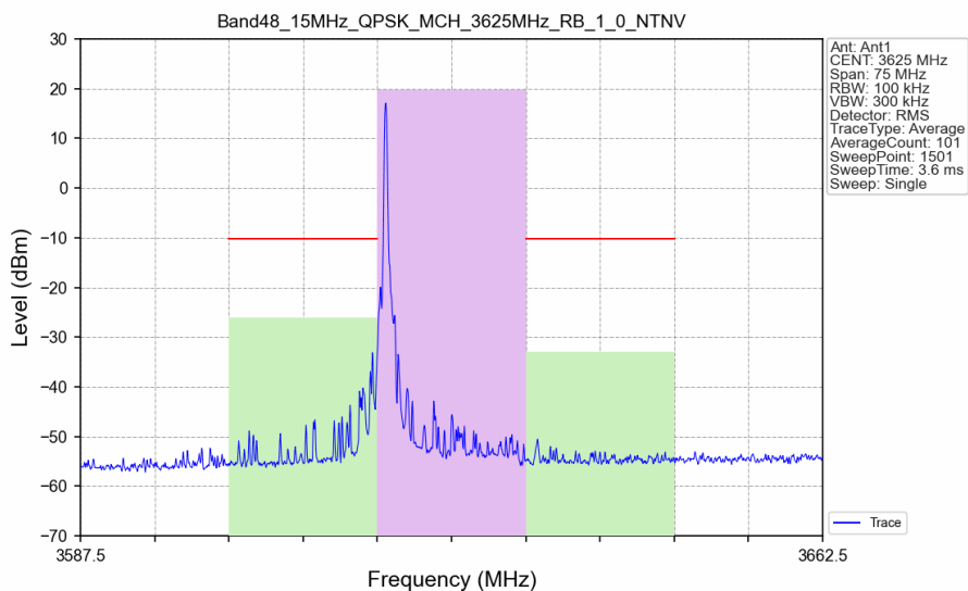
Band48_15MHz_QPSK_MCH_3625MHz_RB_1_0_NTNV
