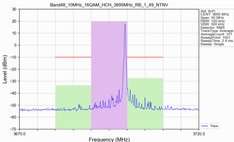
Band48_10MHz_16QAM_HCH_3695MHz_RB_1_49_NTNV
