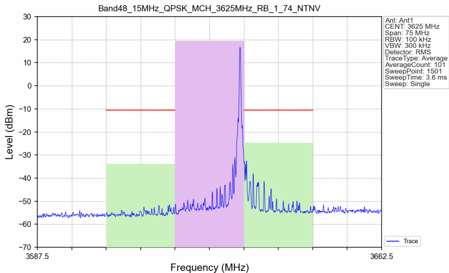
Band48_15MHz_QPSK_MCH_3625MHz_RB_1_74_NTNV
