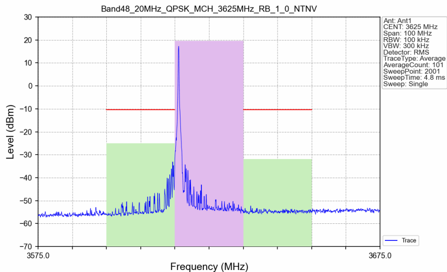
Band48_20MHz_QPSK_MCH_3625MHz_RB_1_0_NTNV
