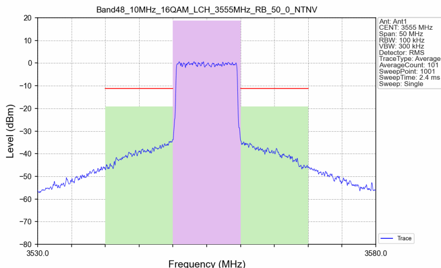
Band48_10MHz_16QAM_LCH_3555MHz_RB_50_0_NTNV
