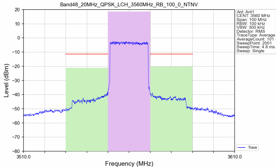
Band48_20MHz_QPSK_LCH_3560MHz_RB_100_0_NTNV
