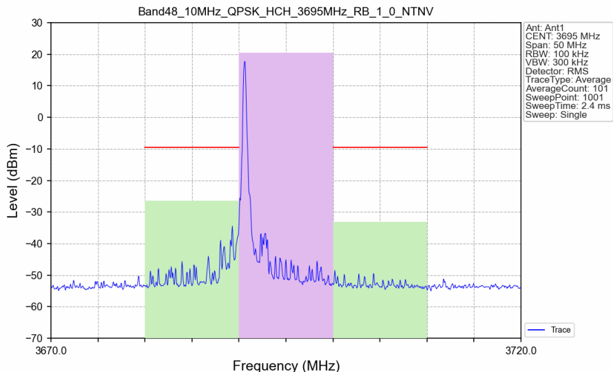
Band48_10MHz_QPSK_HCH_3695MHz_RB_1_0_NTNV
