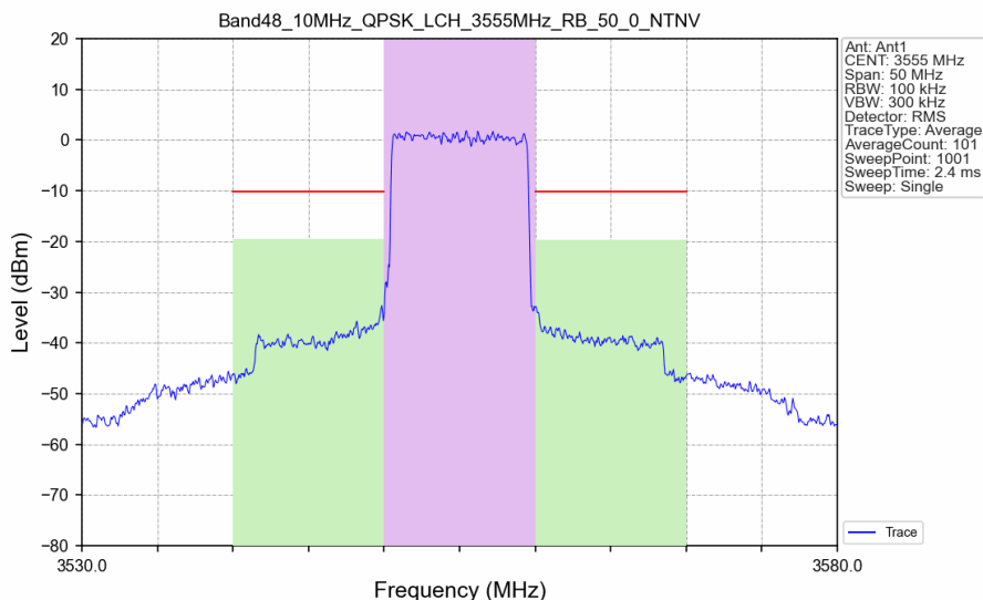
Band48_10MHz_QPSK_LCH_3555MHz_RB_50_0_NTNV
