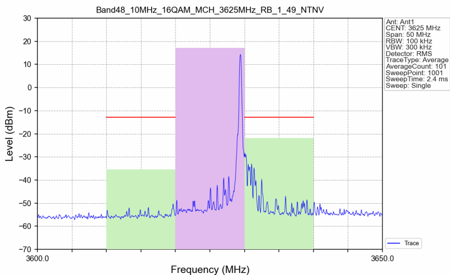
Band48_10MHz_16QAM_MCH_3625MHz_RB_1_49_NTNV
