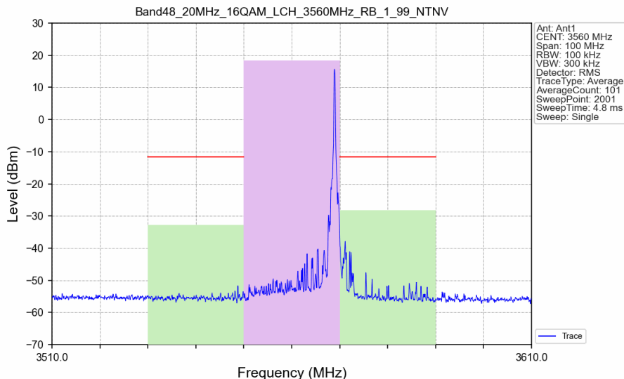
Band48_20MHz_16QAM_LCH_3560MHz_RB_1_99_NTNV
