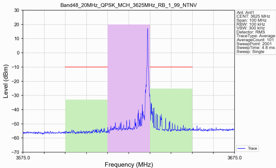
Band48_20MHz_QPSK_MCH_3625MHz_RB_1_99_NTNV
