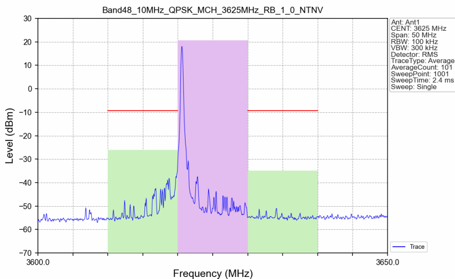
Band48_10MHz_QPSK_MCH_3625MHz_RB_1_0_NTNV
