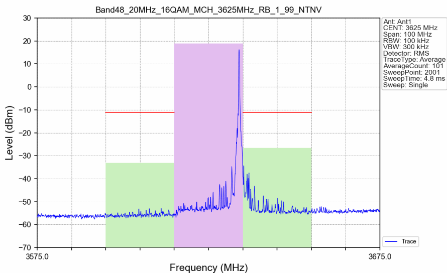
Band48_20MHz_16QAM_MCH_3625MHz_RB_1_99_NTNV
