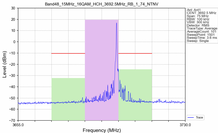
Band48_15MHz_16QAM_HCH_3692.5MHz_RB_1_74_NTNV
