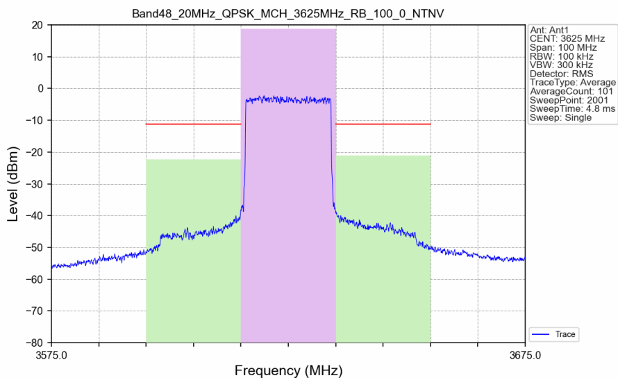
Band48_20MHz_QPSK_MCH_3625MHz_RB_100_0_NTNV
