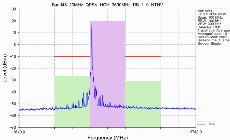
Band48_20MHz_QPSK_HCH_3690MHz_RB_1_0_NTNV
