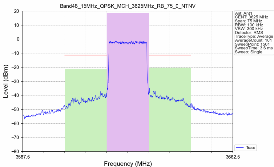
Band48_15MHz_QPSK_MCH_3625MHz_RB_75_0_NTNV
