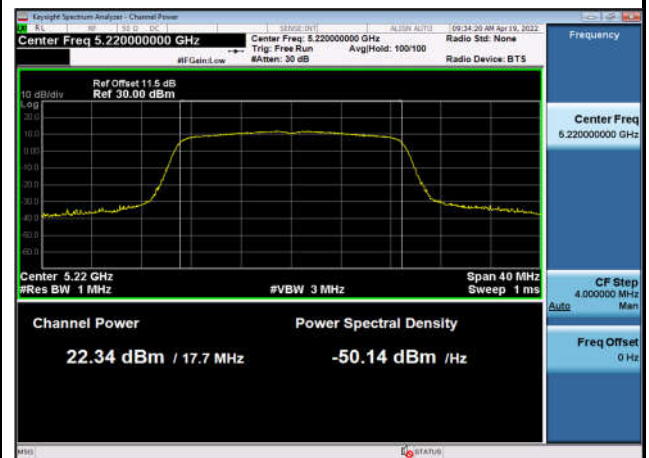
U-NII-1 Output Power-802.11ac(20MHz) ,5220MHz,Ant4
