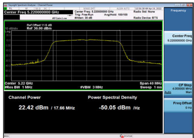
U-NII-1 Output Power-802.11ax(20MHz) ,5220MHz,Ant4
