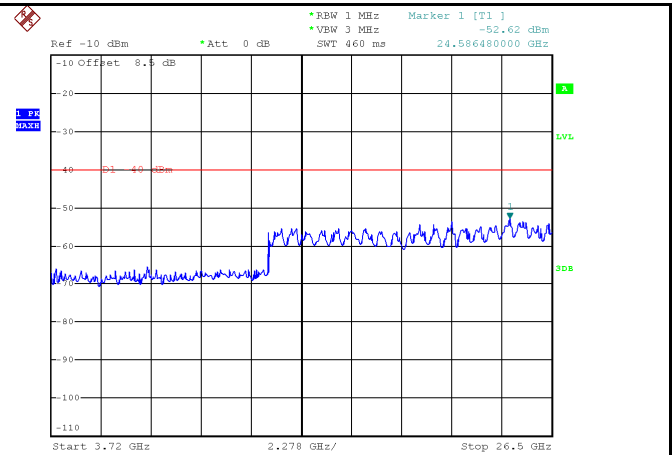
10MHz - Middle CH 3.72GHz~26.5GHz
