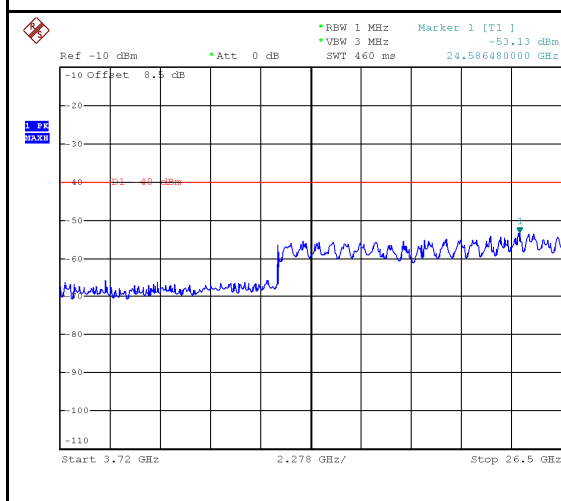
5MHz - Middle CH 3.72GHz~26.5GHz
