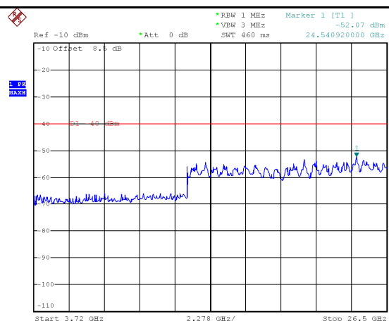
15MHz - High CH 3.72GHz~26.5GHz
