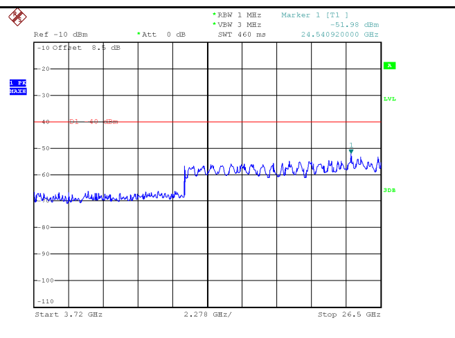
20MHz - Middle CH 3.72GHz~26.5GHz
