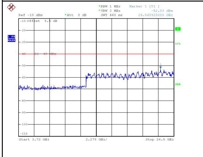
20MHz - High CH 3.72GHz~26.5GHz
