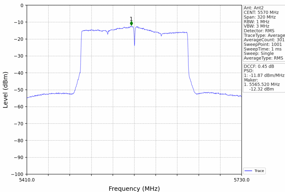
802.11ax(HEW160)_MCH_5570MHz_2xRU996_Left_Ant2_NTNV
