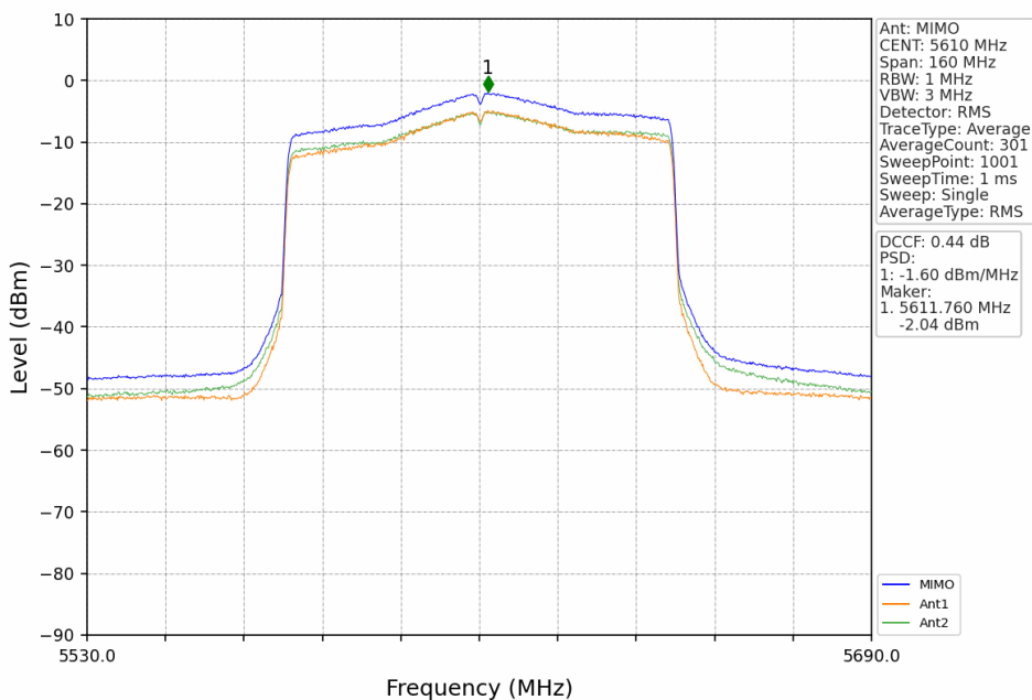
802.11ax(HEW80)_HCH_5610MHz_RU996_Left_MIMO_NTNV
