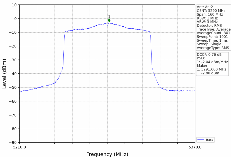
802.11ax(HEW80)_MCH_5290MHz_RU996_Left_Ant2_NTNV
