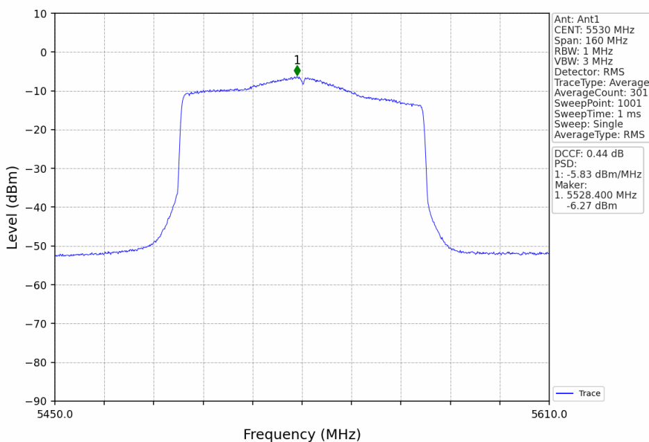
802.11ax(HEW80)_LCH_5530MHz_RU996_Left_Ant1_NTNV
