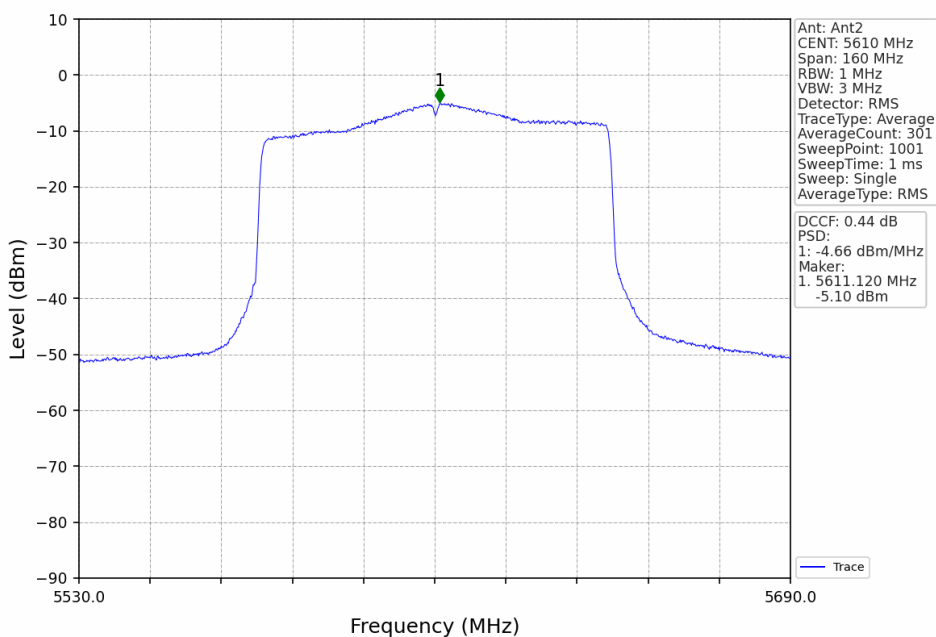
802.11ax(HEW80)_HCH_5610MHz_RU996_Left_Ant2_NTNV
