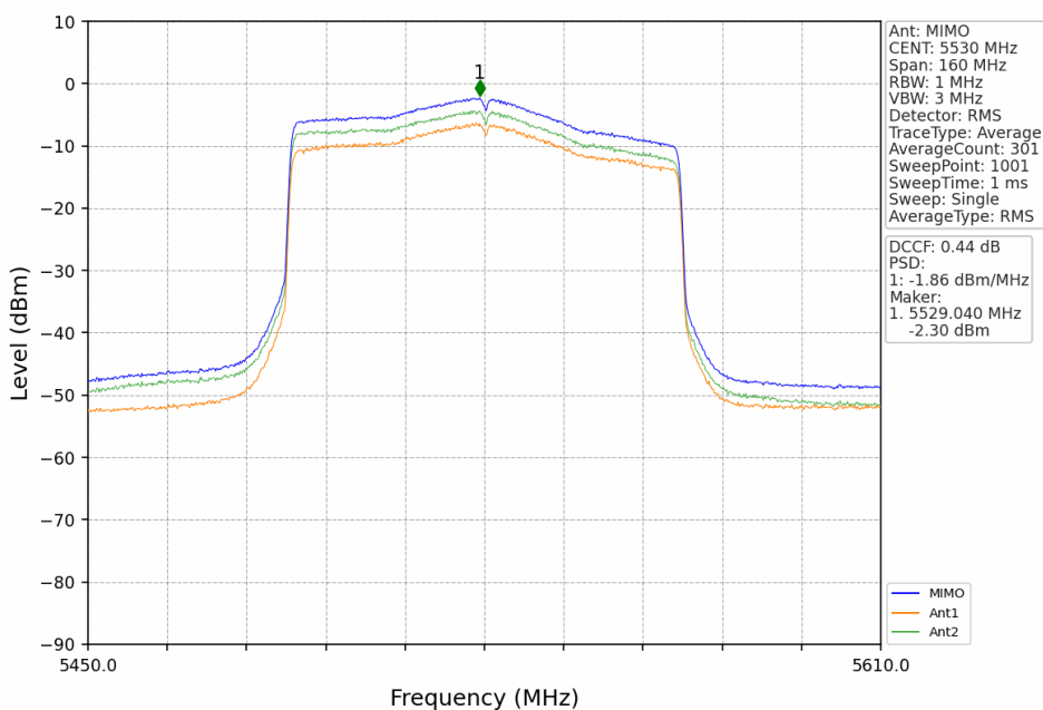
802.11ax(HEW80)_LCH_5530MHz_RU996_Left_MIMO_NTNV
