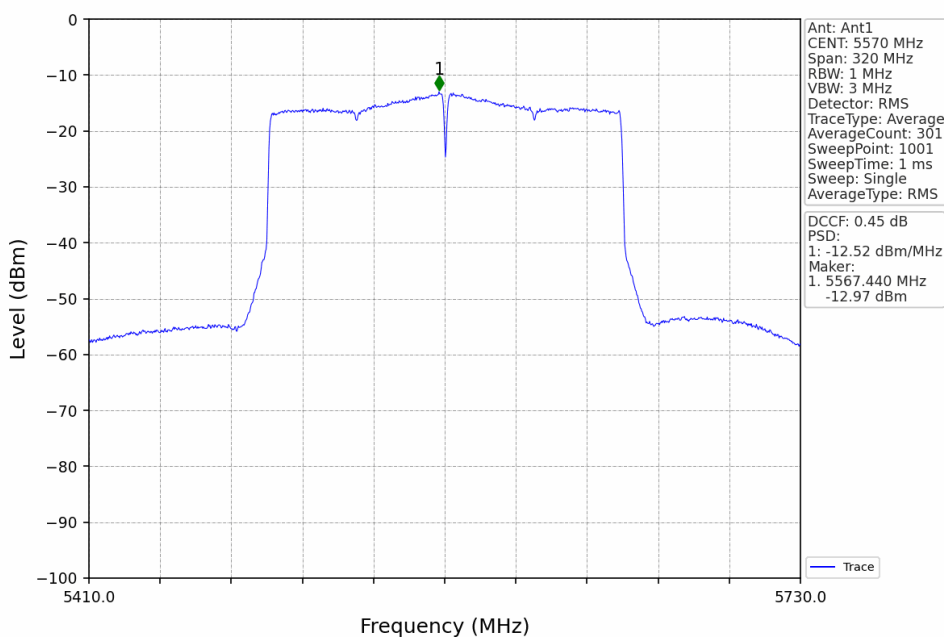
802.11ax(HEW160)_MCH_5570MHz_2xRU996_Left_Ant1_NTNV
