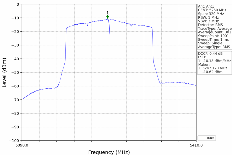
802.11ax(HEW160)_MCH_5250MHz_2xRU996_Left_Ant1_NTNV
