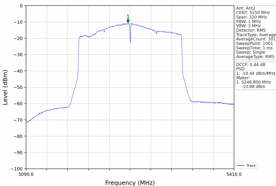
802.11ax(HEW160)_MCH_5250MHz_2xRU996_Left_Ant2_NTNV
