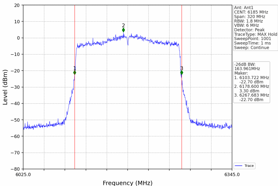
802.11ax(HEW160)_LCH_6185MHz_2xRU996_Left_Ant1_NTNV
