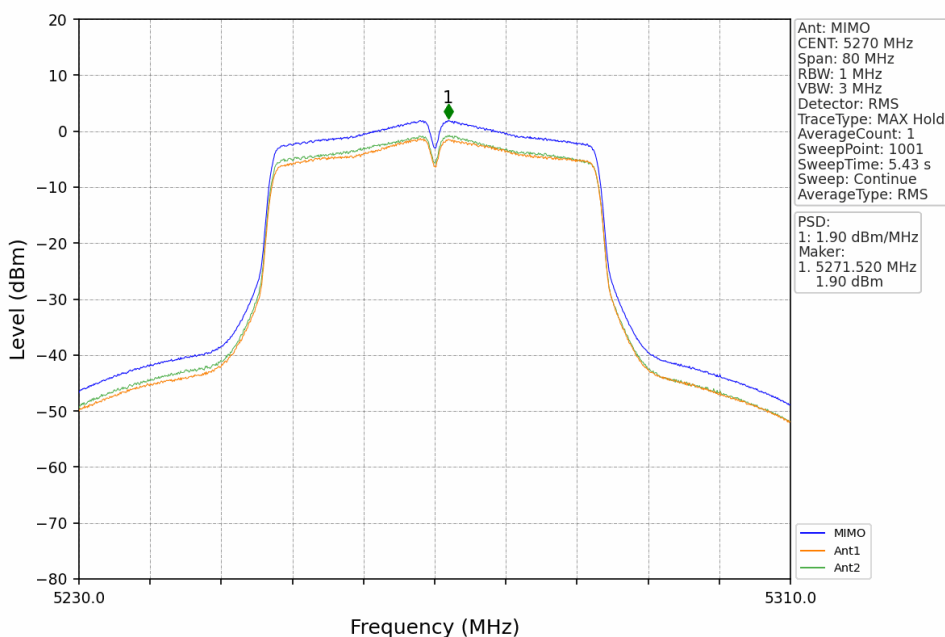
802.11n(HT40)_LCH_5270MHz_MIMO_NTNV
