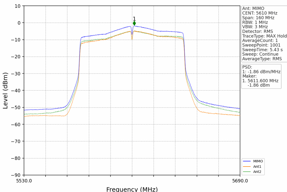
802.11ac(VHT80)_HCH_5610MHz_MIMO_NTNV
