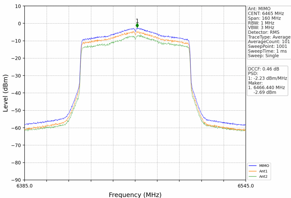
802.11ax(HEW80)_LCH_6465MHz_RU996_Left_MIMO_NTNV
