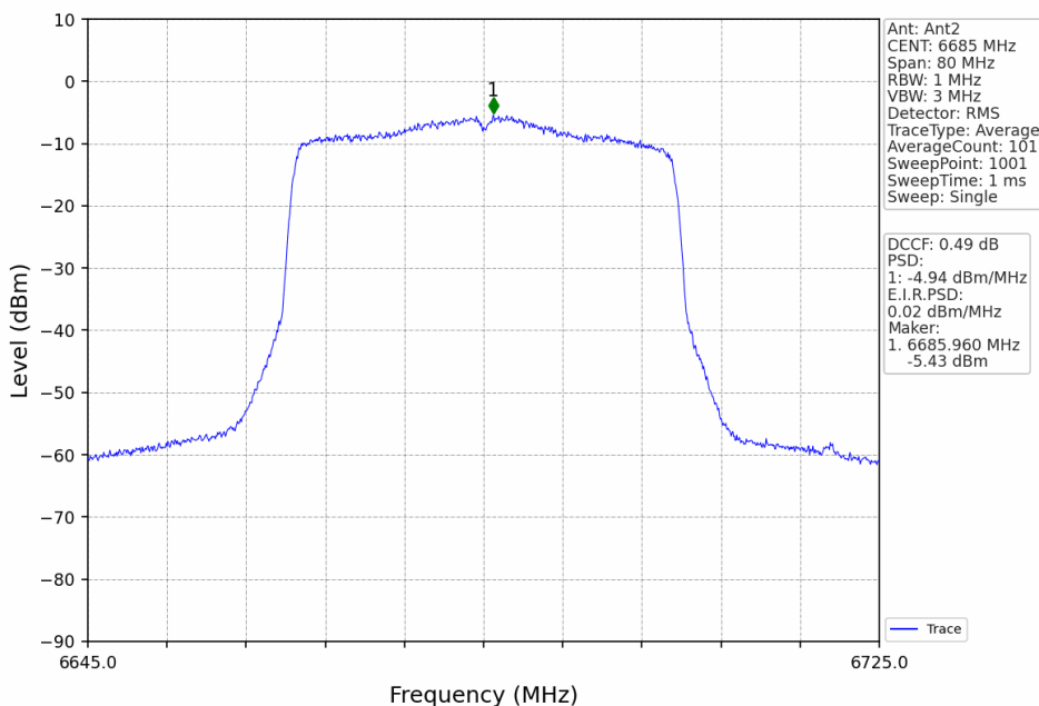
802.11ax(HEW40)_MCH_6685MHz_RU484_Left_Ant2_NTNV
