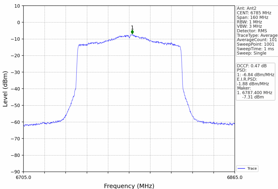
802.11ax(HEW80)_HCH_6785MHz_RU996_Left_Ant2_NTNV
