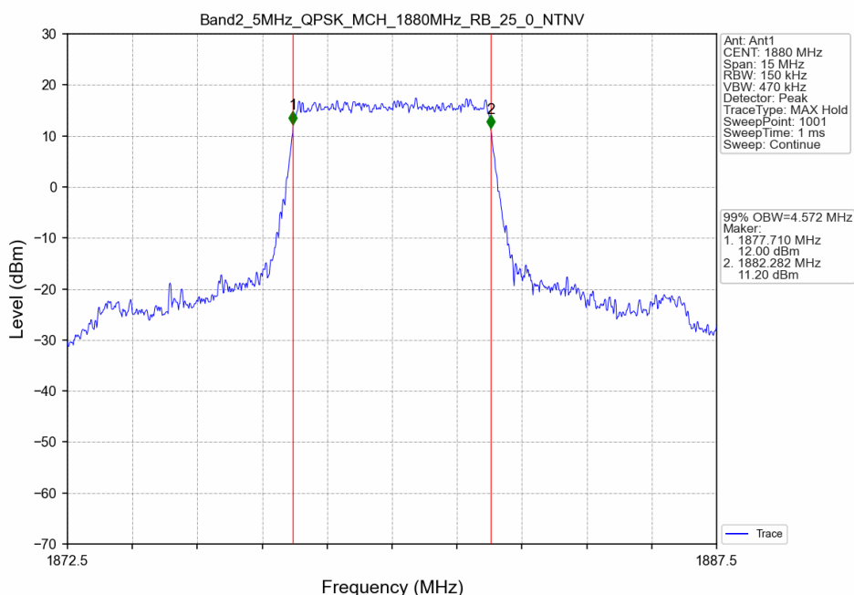
Band2_5MHz_QPSK_MCH_1880MHz_RB_25_0_NTNV
