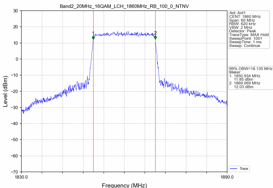
Band2_20MHz_16QAM_LCH_1860MHz_RB_100_0_NTNV
