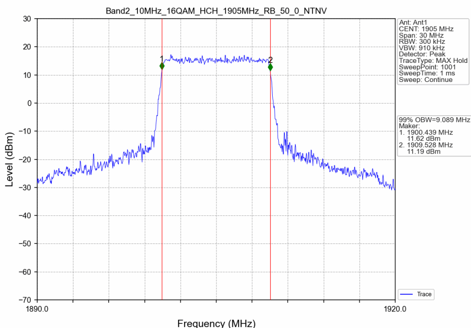
Band2_10MHz_16QAM_HCH_1905MHz_RB_50_0_NTNV
