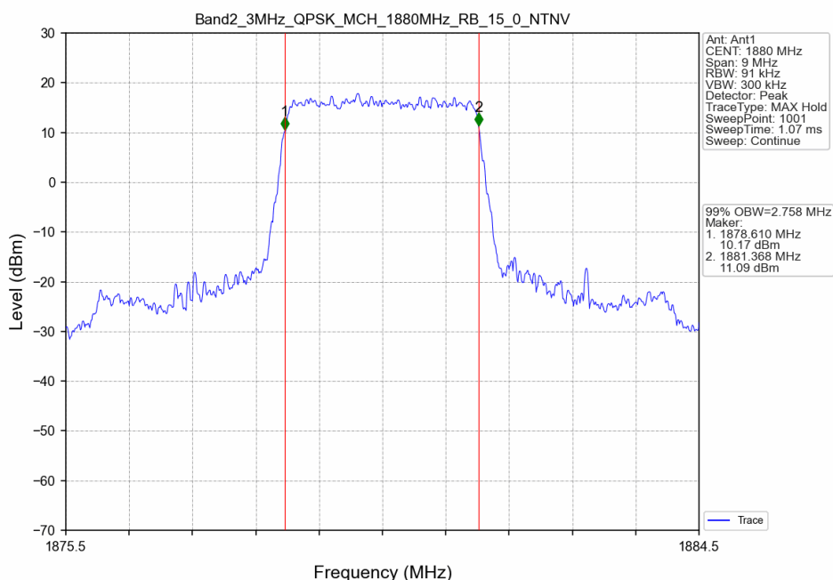
Band2_3MHz_QPSK_MCH_1880MHz_RB_15_0_NTNV
