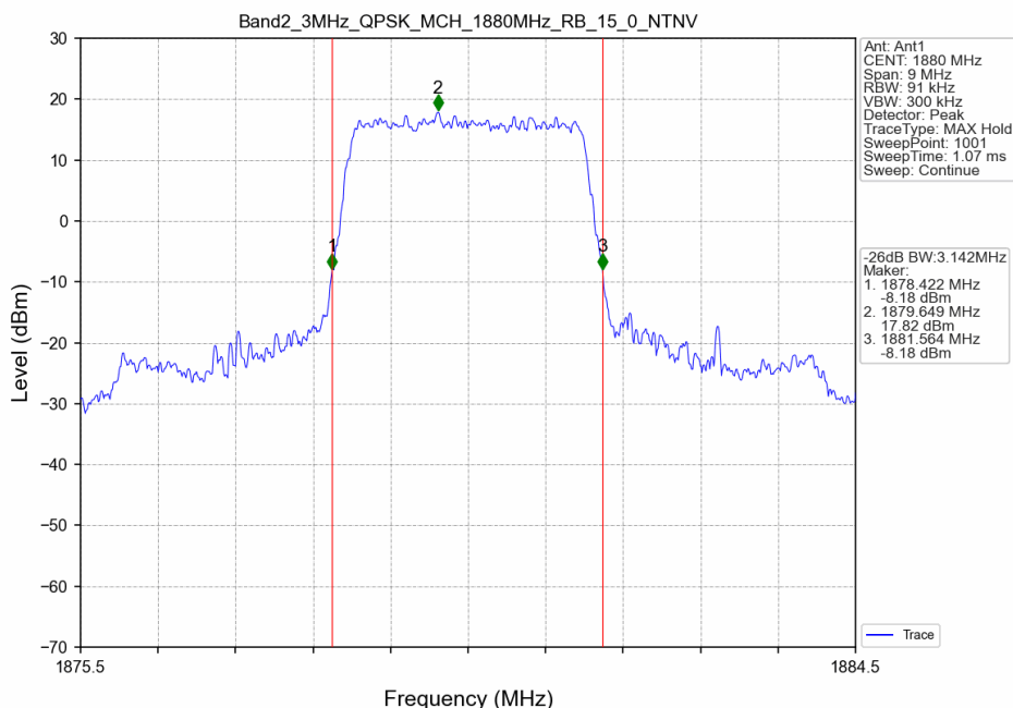
Band2_3MHz_QPSK_MCH_1880MHz_RB_15_0_NTNV
