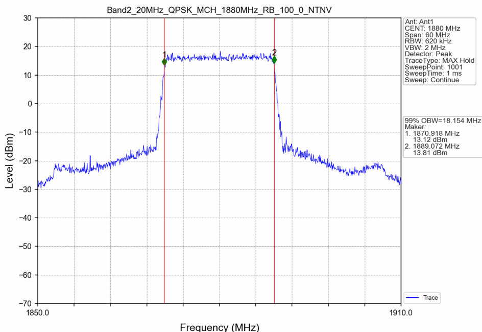
Band2_20MHz_QPSK_MCH_1880MHz_RB_100_0_NTNV
