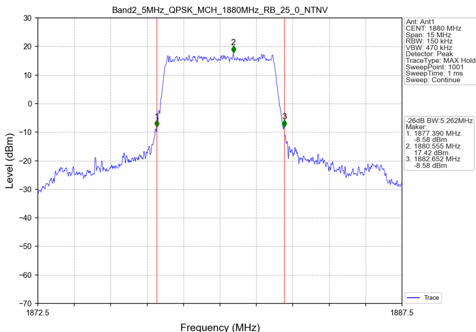
Band2_5MHz_QPSK_MCH_1880MHz_RB_25_0_NTNV
